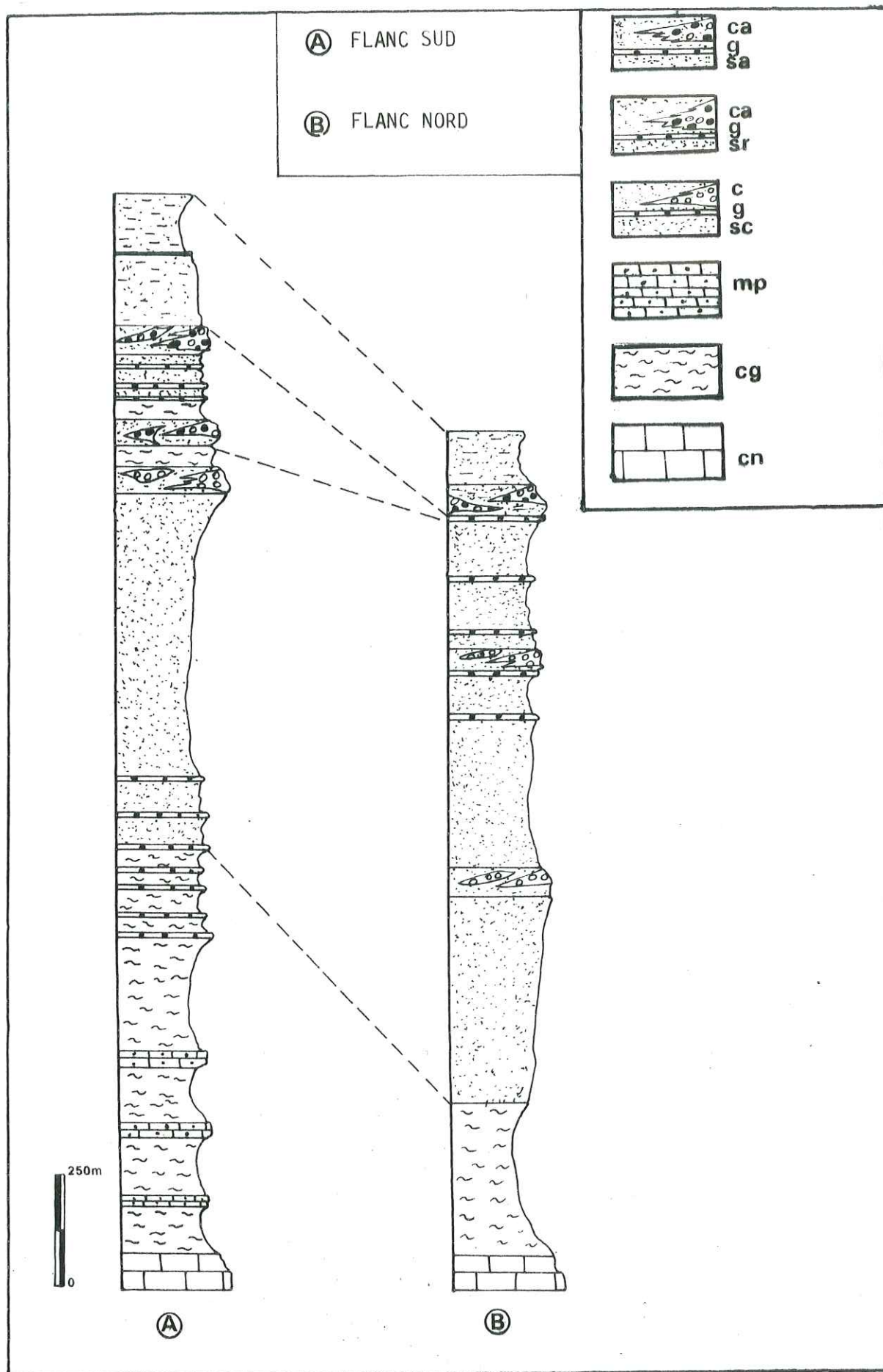
FIG.7 : COUPE DE LA PENNE
