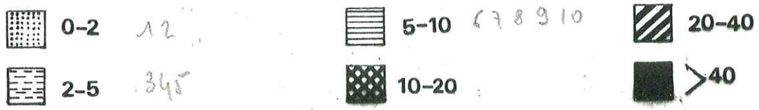
Fig.28 distribution typologique des populations de zircons des granites de Saint-Antonin dans le diagramme (I.A, I.J)
