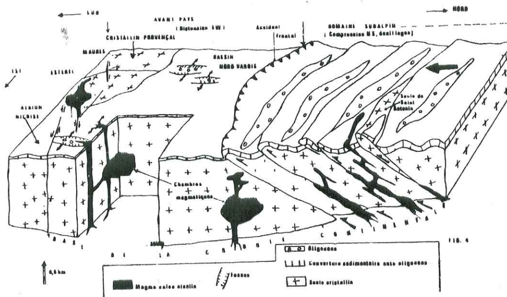
Fig.40 Bloc diagramme illustrant la mise en place du volcanisme dans son contexte structural, a l'Oligocene moyen (echelle des distances horizontales non respectee) (In J. D. GIRAUD et G. TURCO, 1981)
