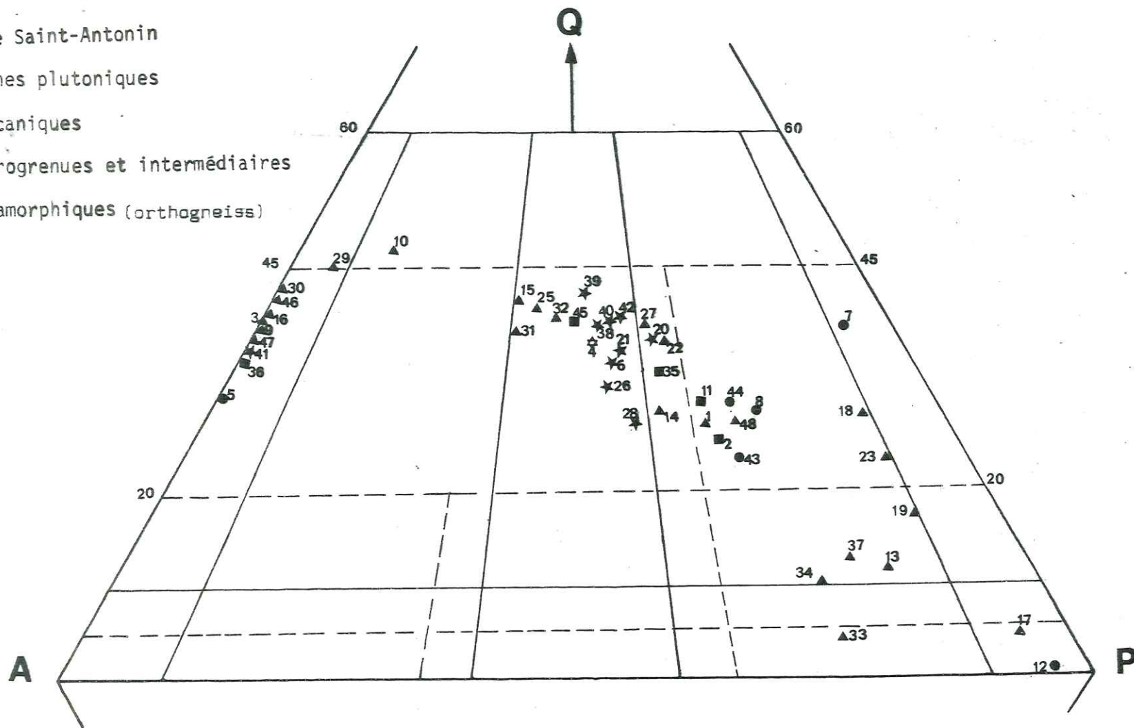
Fig.23 Répartition de quelques échantillons (galets) étudiés dans le diagramme Q. A. P. (à partir de normes C.I.P.W.)
