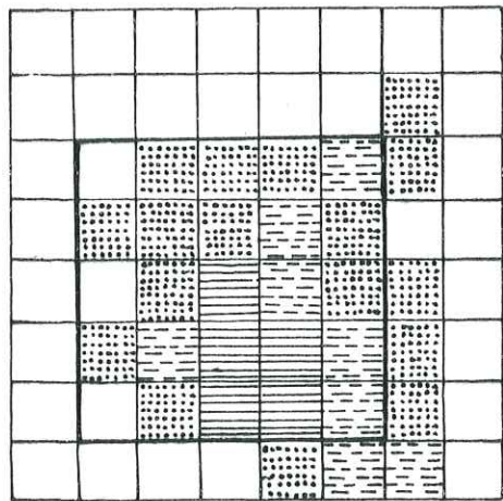
Distribution typologique de population de zircons de grès permien supérieur d'Aigue-Bonne, Estérel (ES.161 - PUPIN 1976)
