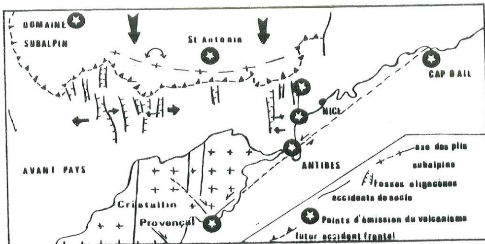
Fig. Le domaine envisage a l'Oligocene moyen-supérieur (echelles non respectees).
