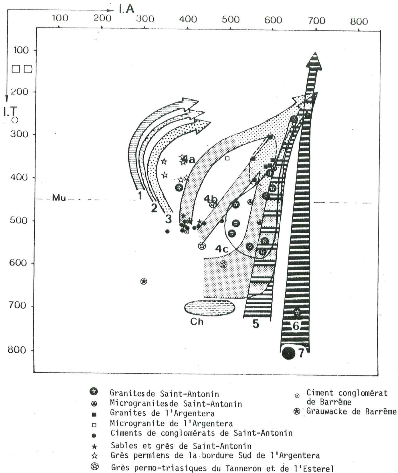
Fig.36 Points moyens de diverses populations de zircons étudiées dans le diagramme (I.A., IT)
