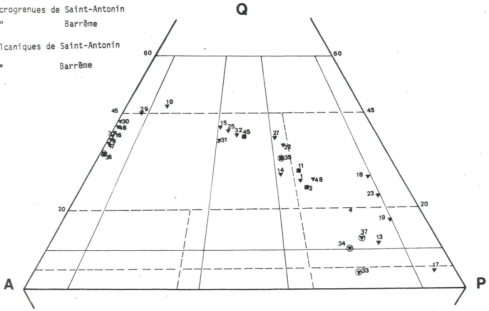
Fig.50 : Répartition des roches microgrenues et volcaniques dans le diagramme Q.A.P. (A partir de normes C.I.P.W.)
