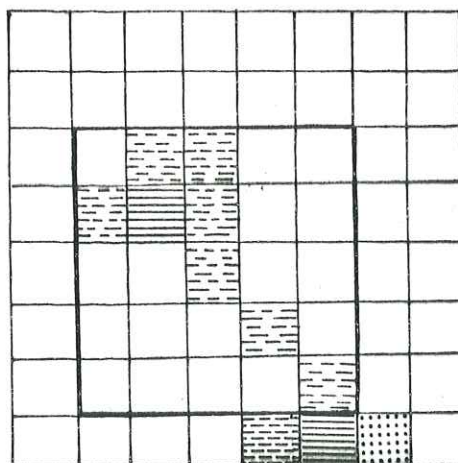
Distribution typologique de population de zircons de l'arkose de Roquebrune-sur-Argens Sud du Muy, Estérel occidental (MA. 166 - PUPIN 1976)
