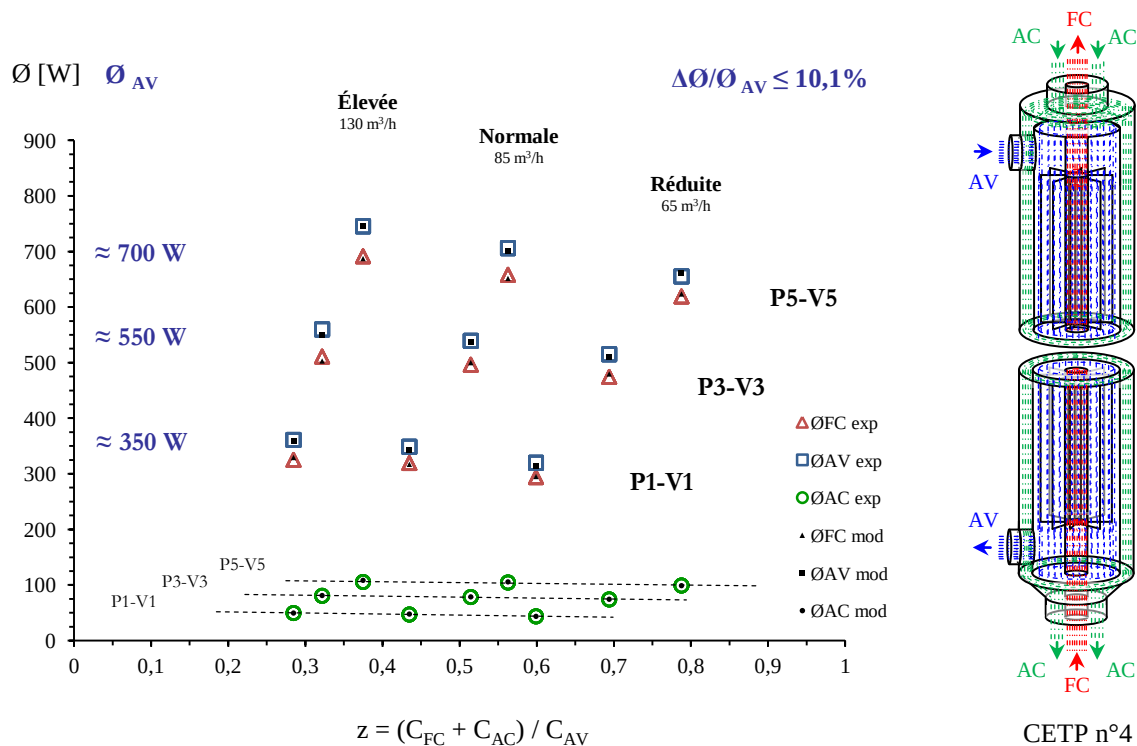
Figure 3.24 : Puissances échangées au sein du CETP n°4
