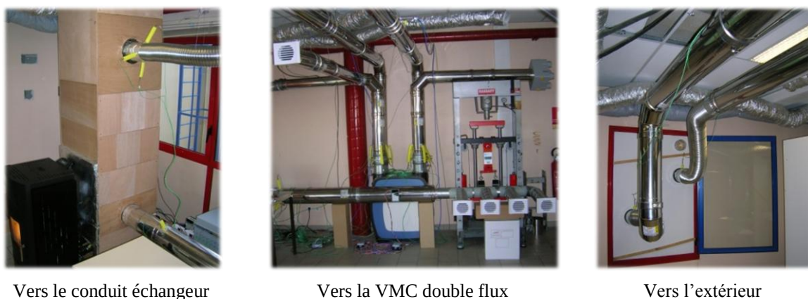
Figure 3.9 : Vues du réseau de ventilation lors des essais en laboratoire
