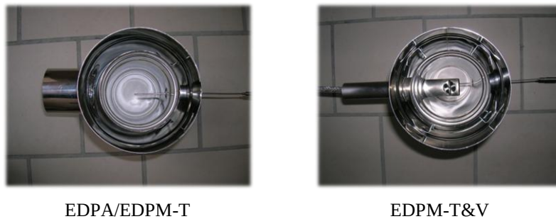
Figure 3.8 : Vue des deux éléments de prise de mesure instrumentés sur les fumées
