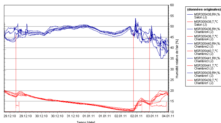
Figure 3.58 : Détails des mesures relevées dans le logement J pendant la période d'inoccupation
