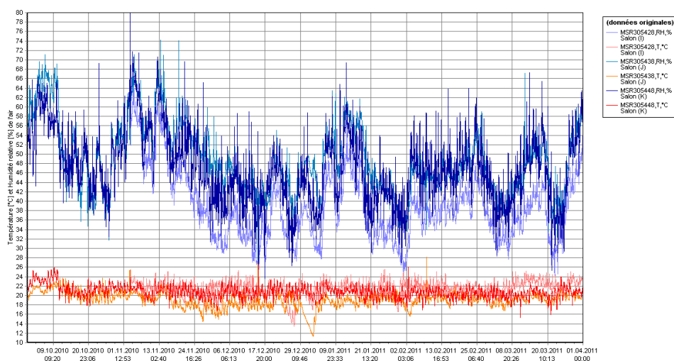
Figure 3.54 : Superposition de la température et de l'humidité relative dans le salon des trois logements
