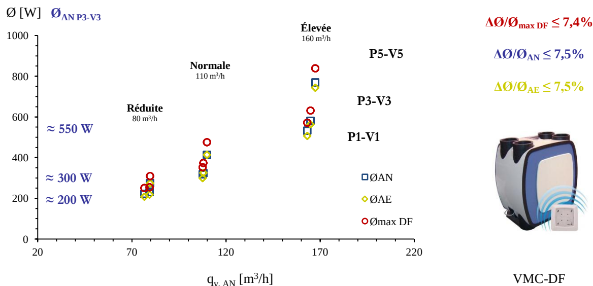
Figure 3.30 : Puissances transférées et maximum récupérables dans la VMC-DF (CETP-NI n°4)
