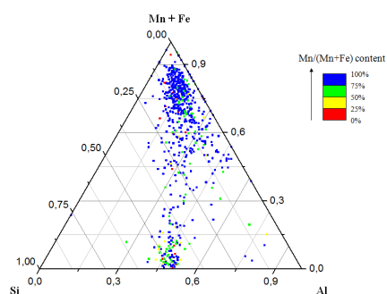
(c) Diagramme ternaire Al-Si-(Mn+Fe) pour les particules prélevées dans la cheminée B.
