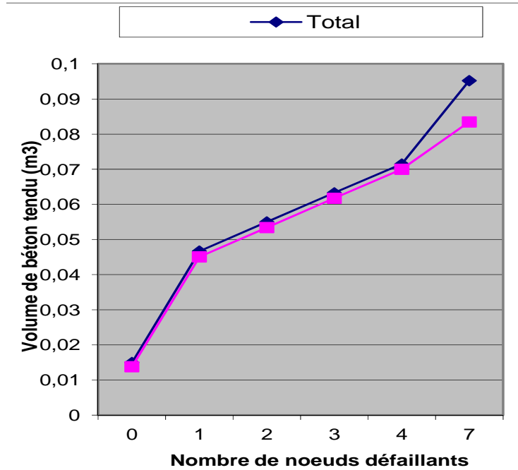
Figure 4.66. Variation du volume de béton tendu avec le nombre de nœuds défailants.
