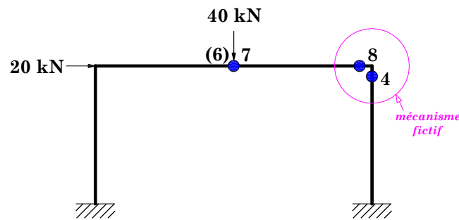
Figure 3.26. Illustration du mécanisme fictif 8 → 4.
