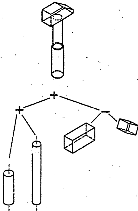
Figure 1-2 : Représentation d'un arbre CSG Cette figure est extraite de [BR084].
