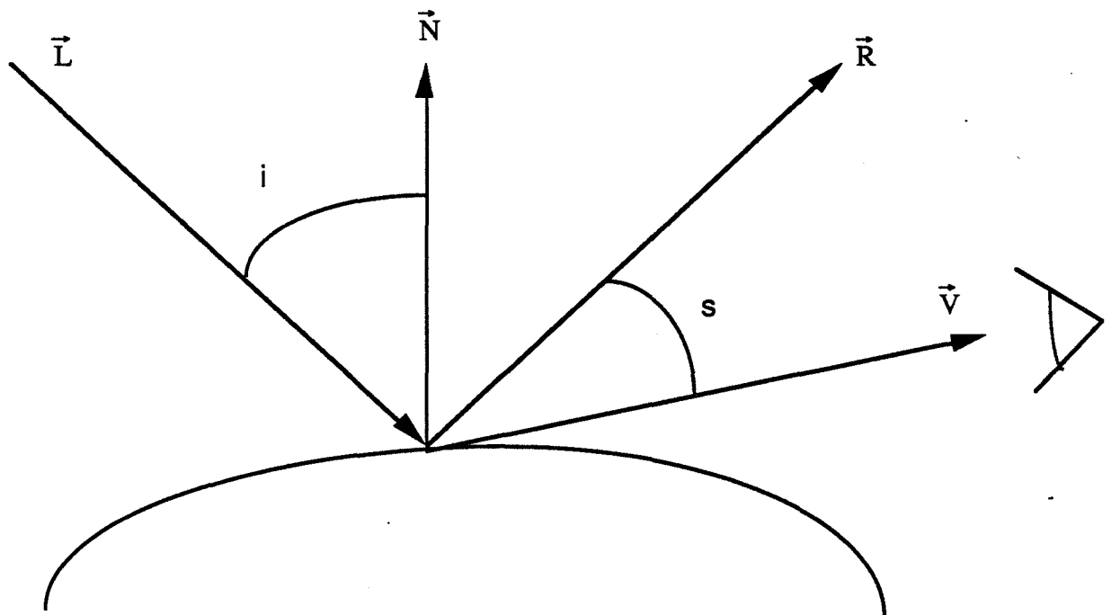
Figure 6 : Réflexion spéculaire
