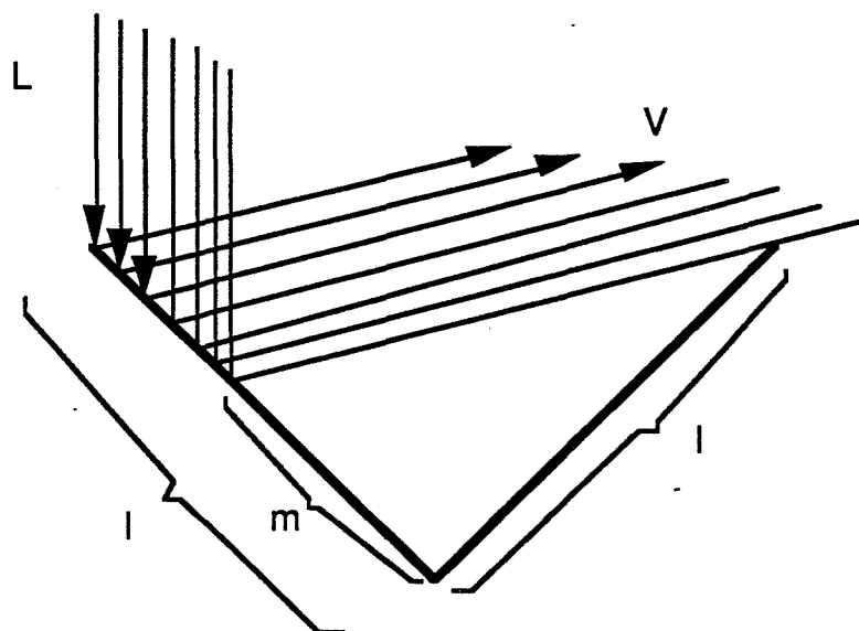
Figure 7.2 : Atténuation géométrique
