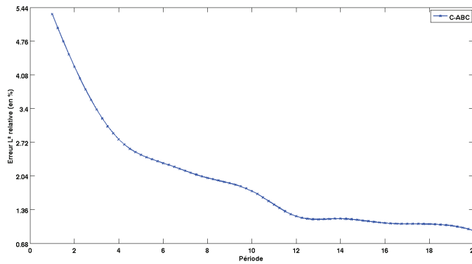
FIG. 2.27 – Erreur L^2 pour k=1
