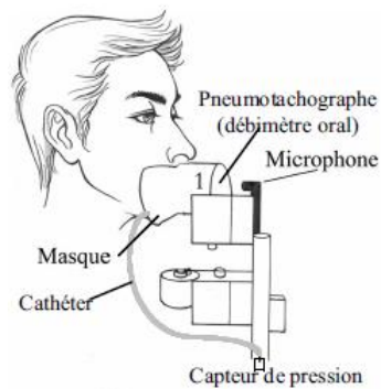
Figure 4.2 – Pièce à main du dispositif EVA2 permettant les prises de mesures simultanées de données aérodynamiques et acoustiques (d'après Basset & al. 2006).
