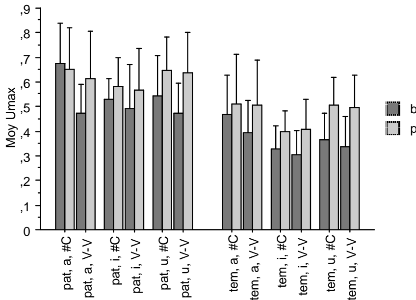
Figure 6.14 – Valeurs moyennes de U_{max} — pic du DAB — (en dm^3/s ) en fonction des sujets, du type de voyelle, du voisement et de la position dans le logatome (les barres d'erreurs représentent les écarts-types) ( n = 240 ).
