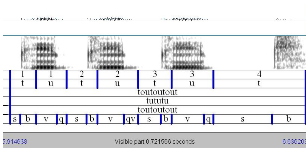
Figure 6.18 – Segmentation du logatome [tututut] sous Praat (exemple du témoin n°1). La tire que nous devons prendre en compte et qui représente une segmentation correcte est la dernière où « s » correspond au silence de l’occlusive, « b » correspond au relâchement de la consonne, « v » correspond à la voyelle et « qv » correspond au Voice Decay Time .
