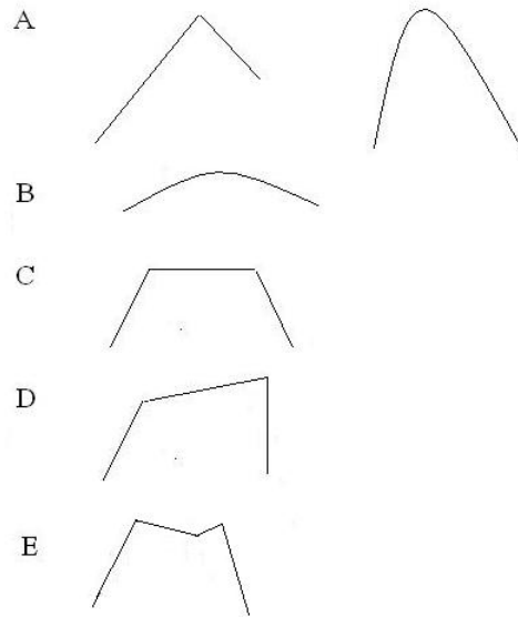
Figure 6.6 – Modélisations des patterns de PIO retrouvés dans nos données pour les logatomes contenant les labiales [p] et [b].
