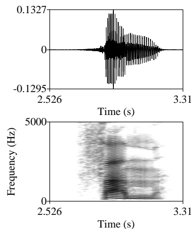
Figure 3.12 – Exemple d’un spectrogramme à bandes étroites du mot «femme» issu de Praat.
