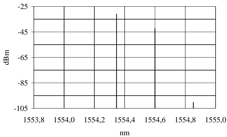
Figure IV.13 Simulations d'un filtre BLU-AALO centré à 31,5 GHz. (a) Signal DBL d'entrée, (b) réponse spectrale et (c) spectre de sortie pour des paramètres de simulation : k = 100 , \sigma = 7 mm, \alpha = 1,82 . La température du cristal est de 20^\circ .
