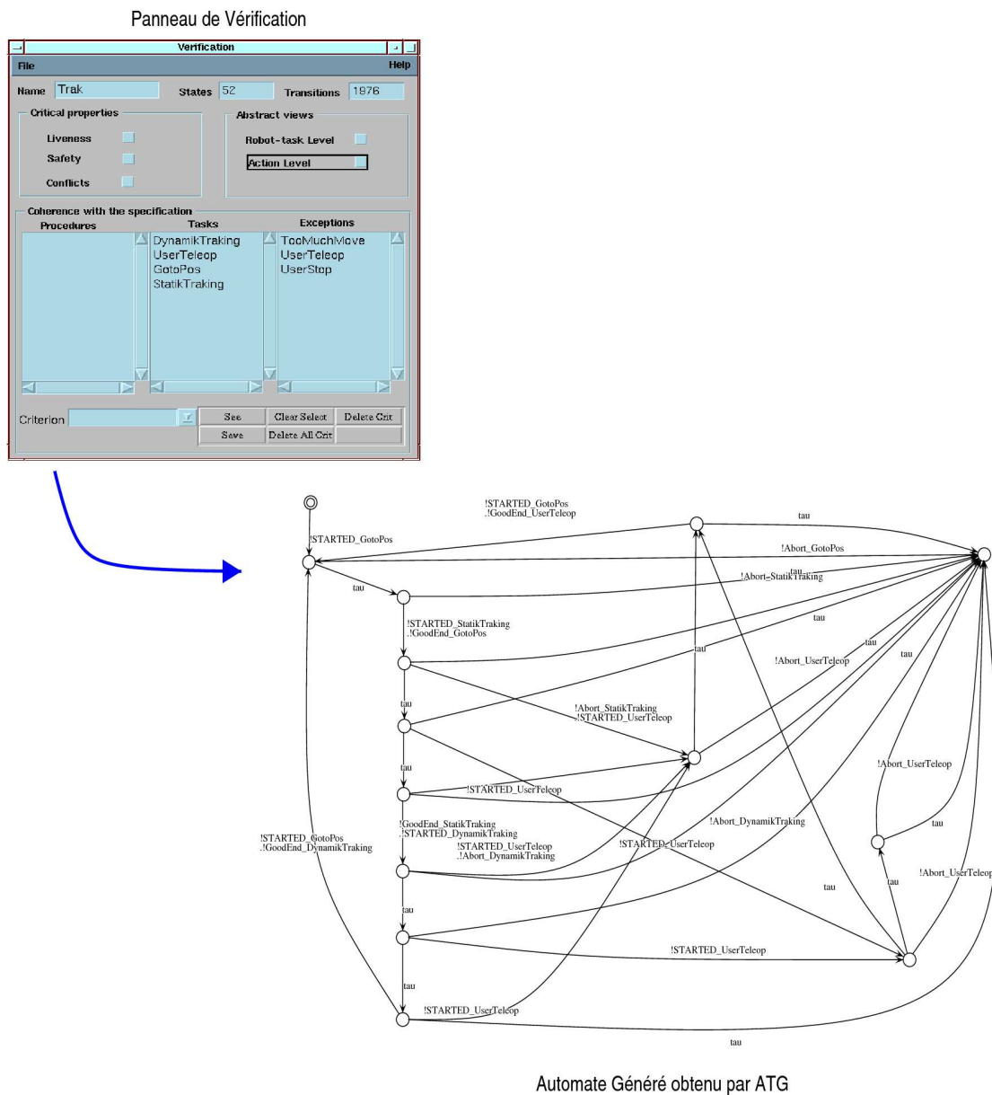
FIG. 6.10 – Visualisation sous ATG de l'automate, représentatif de l'application complète, restreint afin d'étudier le contrôle logique des actions utilisées. En l'occurrence, on observe l'enchaînement des événements de déclenchement et d'arrêt des différentes tâches composant l'application.
