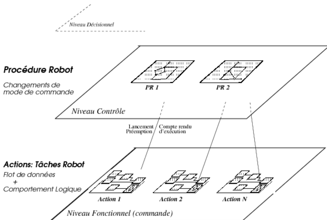
FIG. 5.1 – L'architecture ORCCAD
