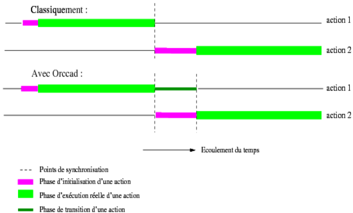
FIG. 7.1 – Synchronisation entre deux tâches successives
