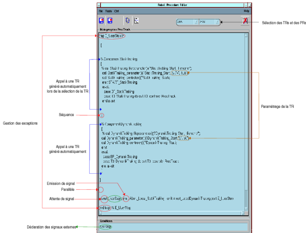
FIG. 6.8 – Spécification d'une application
