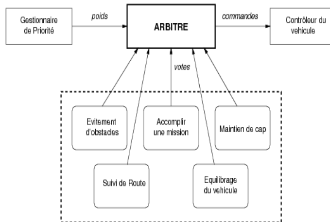
FIG. 3.2 – Structure générale de DAMN
