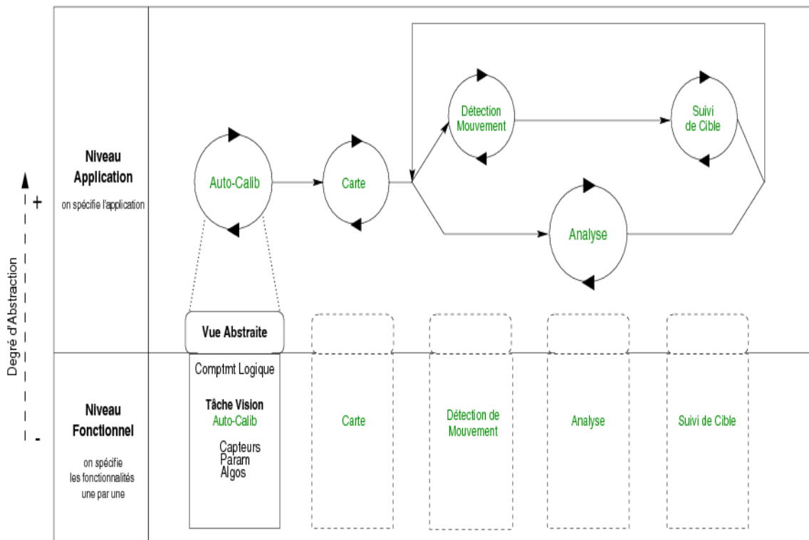
FIG. 4.14 – Hiérarchie de spécification proposée
