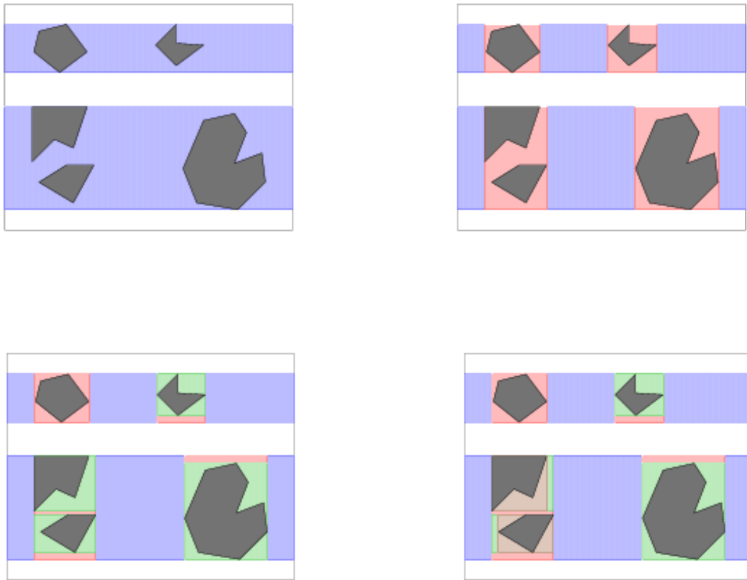
FIG. 4.5 – On commence à balayer l'image dans une direction, ici la direction horizontale et on réitère le processus pour chaque zone décelée. Ici, les zones issus du premier balayage sont en bleu, celles du deuxième balayage en rouge.
