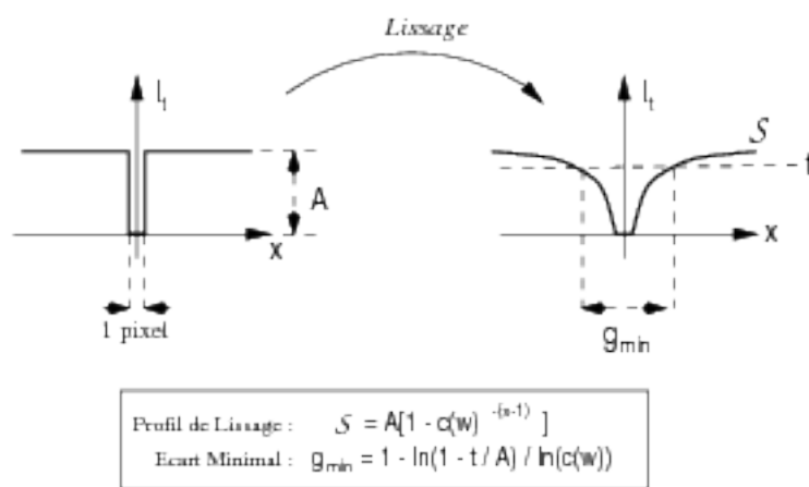
FIG. 4.11 – Évaluation de l'intervalle entre deux régions consécutives suite au lissage et seuillage de l'image. Ici les formules correspondent à un filtre récursif exponentiel (récursif au premier ordre) qui a été utilisé. Le paramètre c du filtre est lié directement à la fenêtre de lissage w .
