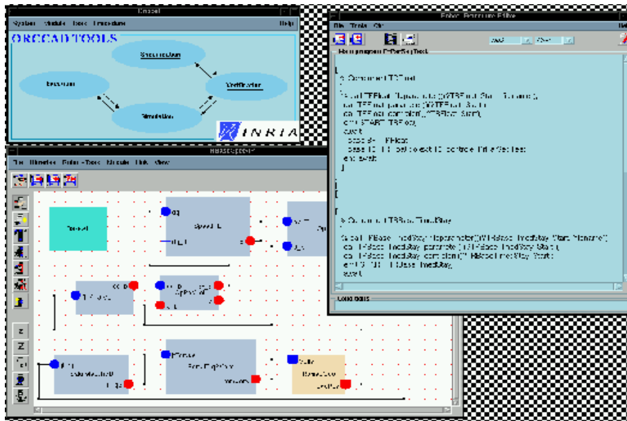
FIG. 5.3 – Une vue d'ensemble de l'environnement ORCCAD
