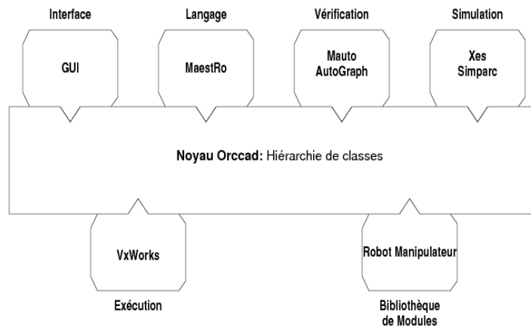
FIG. 5.4 – ORCCAD conçu comme une boîte à outils
