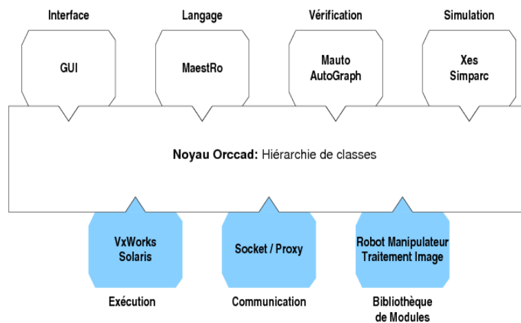
FIG. 7.4 – Nouvelle organisation de la boîte à outils ORCCAD, les contributions apparaissent en couleur.
