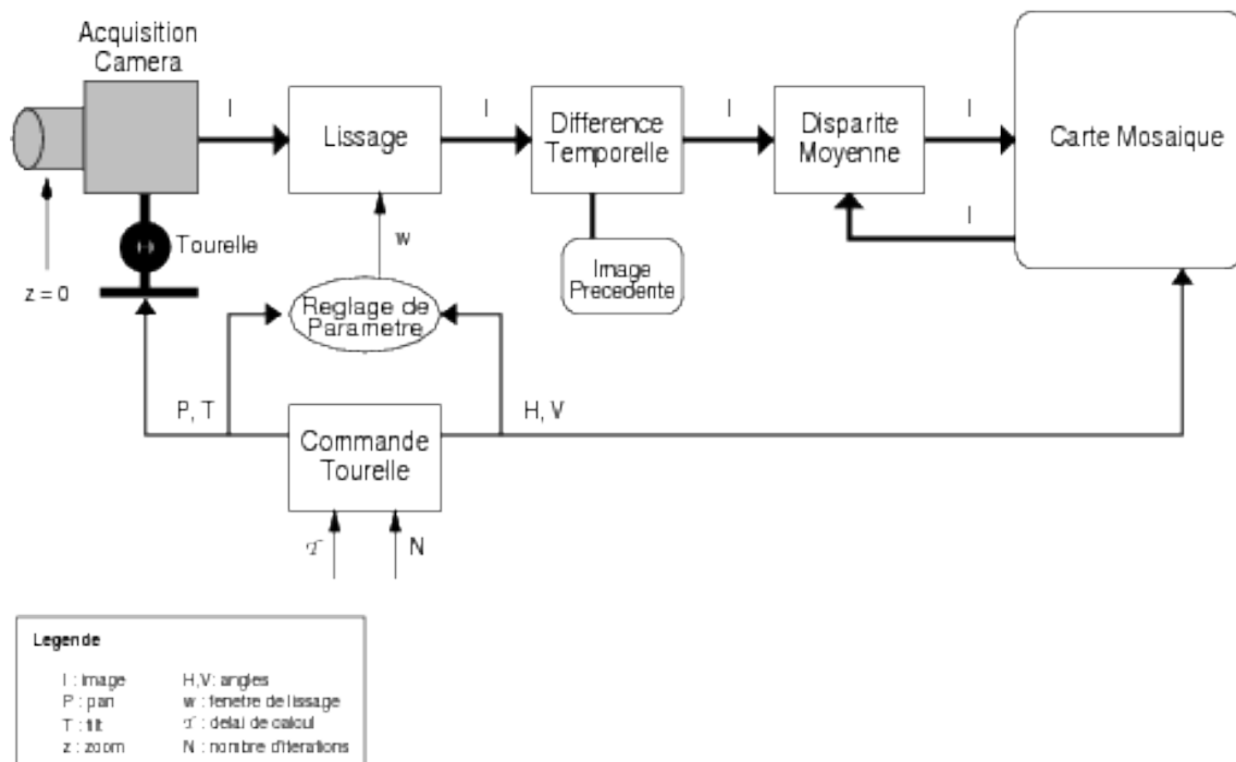
FIG. 4.1 – La séquence d'actions pour l'élaboration de la carte de la scène.
