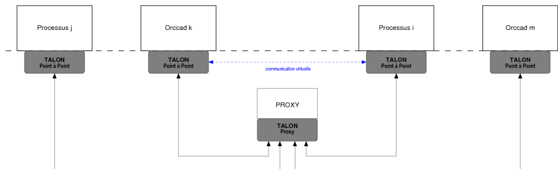
FIG. 8.5 – Architecture d'implantation en couches pour le proxy
