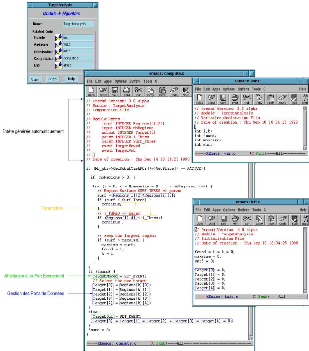
FIG. 6.6 – Spécification du code associé à un module algorithmique
