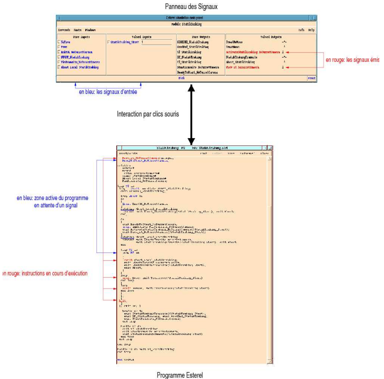
FIG. 6.12 – Interface de simulation de la partie comportement logique avec l’outil XES. Le panneau supérieur présente les signaux d’entrée (à gauche), de sortie (à droite) qui peuvent être respectivement envoyés au, ou produits par le programme ESTEREL qui figure dans la fenêtre inférieure. On sélectionne les signaux d’entrée à envoyer dans le panneau supérieur, on simule "l’instant" d’occurrence des signaux en cliquant sur le bouton tick . Alors, les signaux sont envoyés au programme et instantanément on visualise les signaux de sortie produits en réaction (panneau supérieur) et l’état du programme (fenêtre inférieure).
