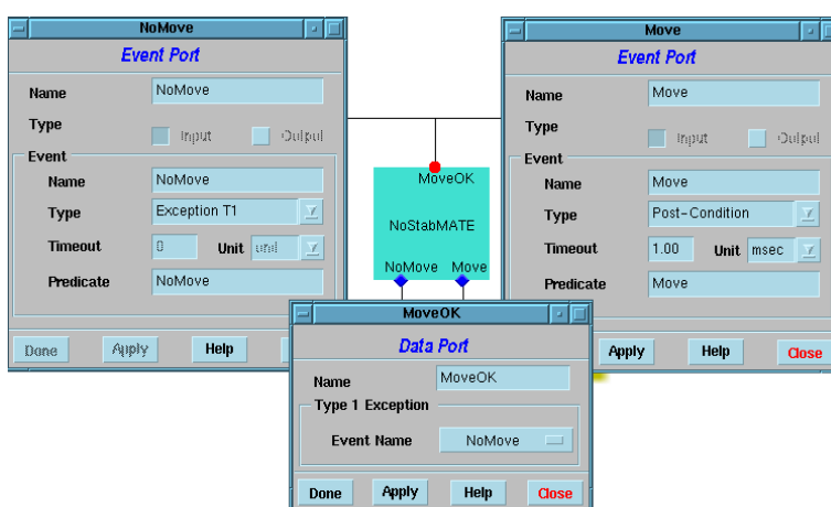
FIG. 6.7 – Spécification du module de comportement ou automate
