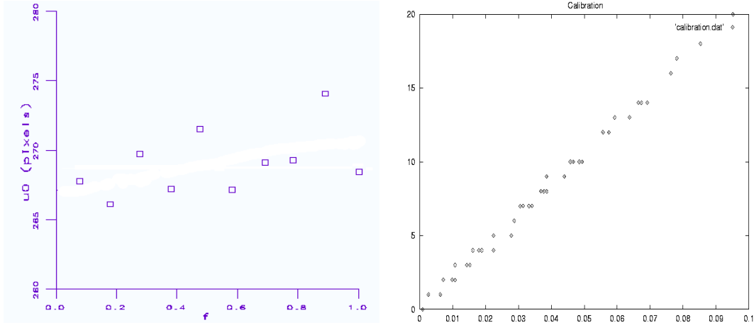
FIG. A.1 – Calibration du pan en pixel/radian : la variation du centre optique est inférieure à 10 pixels (à gauche) tandis que la linéarité du modèle par rapport à la focale est bien vérifiée (à droite).
