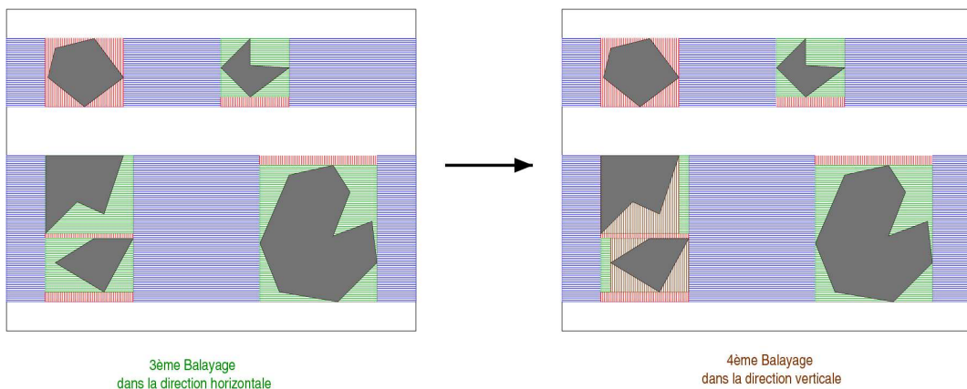
FIG. 4.6 – On continue le balayage tant que toutes les zones n'ont pas fini d'être explorées. Le troisième balayage est représenté en vert et le dernier balayage en brun.
