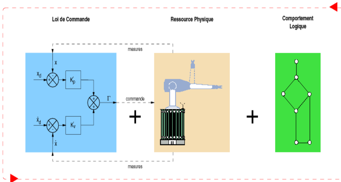
FIG. 5.2 – Définition de la Tâche Robot
