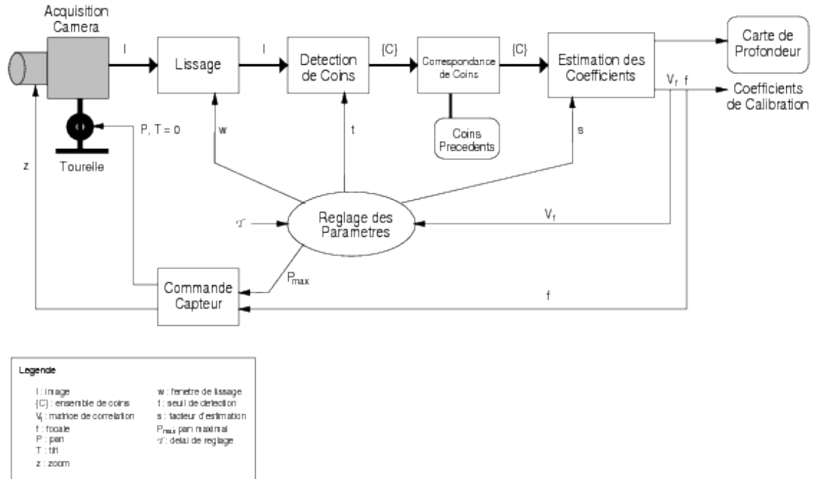
FIG. 4.2 – La séquence d'actions pour l'auto-calibration.
