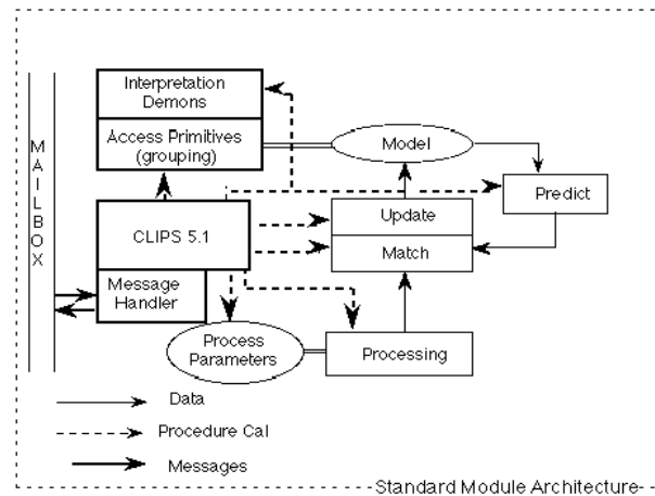
FIG. 3.3 – Structure standard du module manipulé par SAVA.
