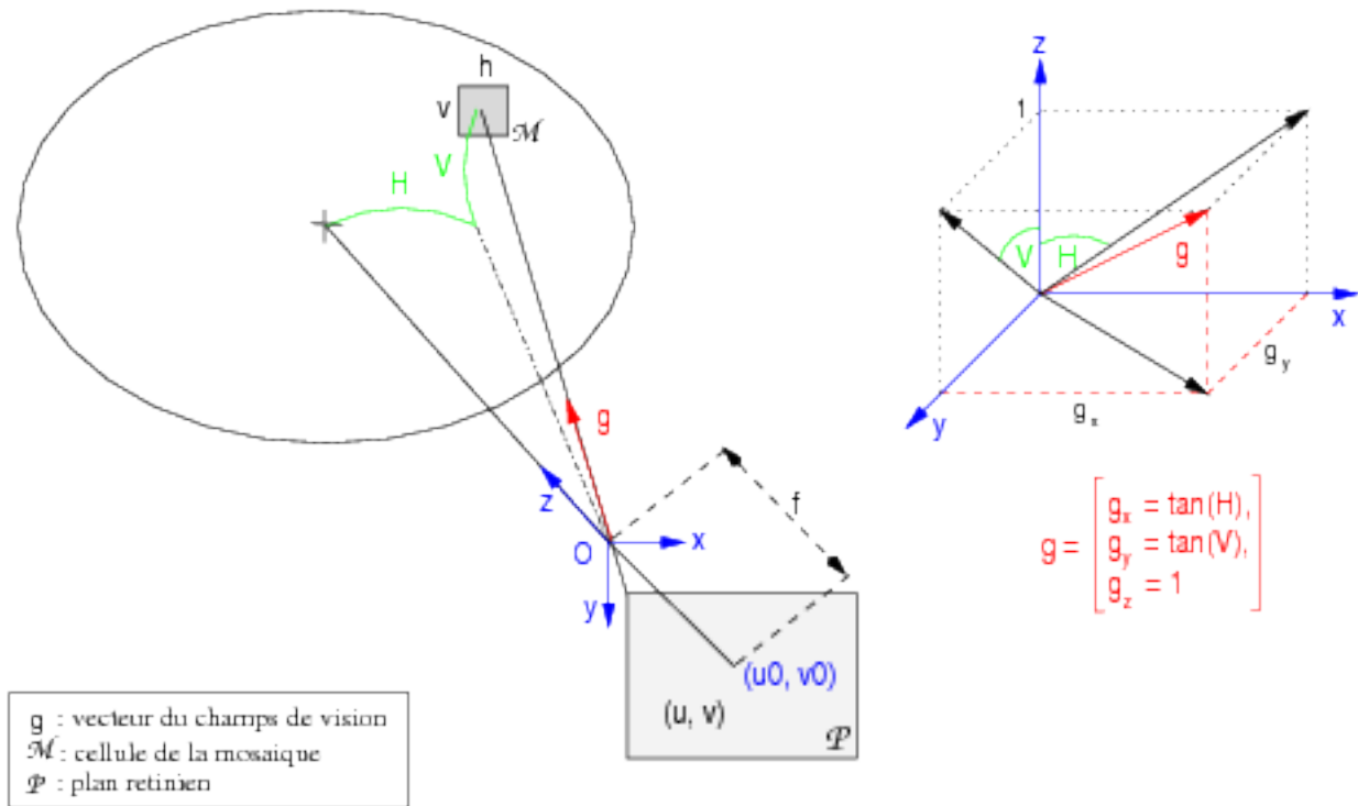
FIG. A.2 – Représentation de la mosaïque. Chaque cellule contient de l'information relative à la scène observée suivant une direction obtenue par projection sur le plan rétinien.
