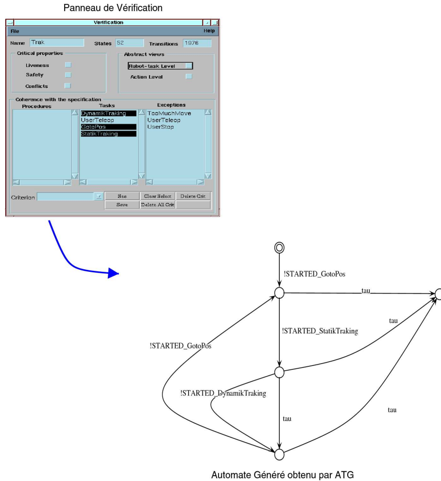
FIG. 6.11 – Automate réduit pour permettre la validation visuelle d'une propriété particulière du comportement logique d'une partie de l'application.
