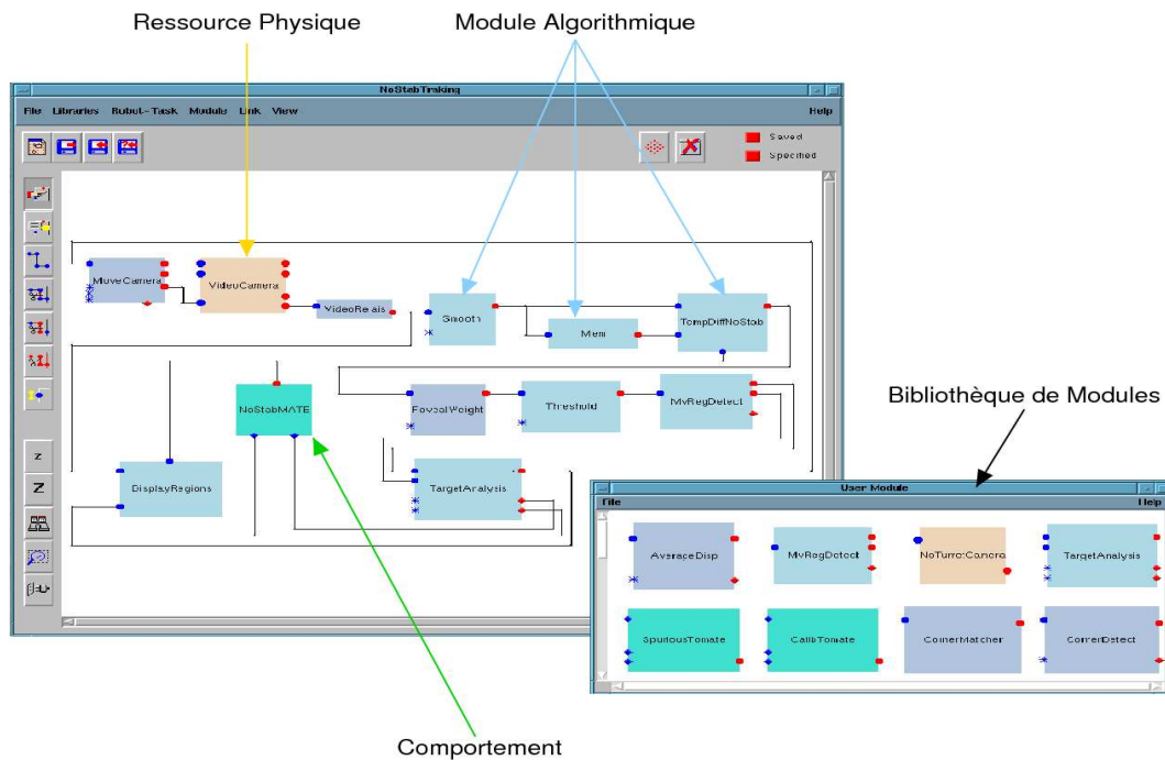
FIG. 6.2 – Spécification d'une Tâche Vision
