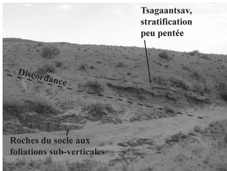
Fig. 6.19 : Discordance de la Formation de Tsagaantsav sur les roches métamorphiques du socle marquées par une foliation sub-verticale.
