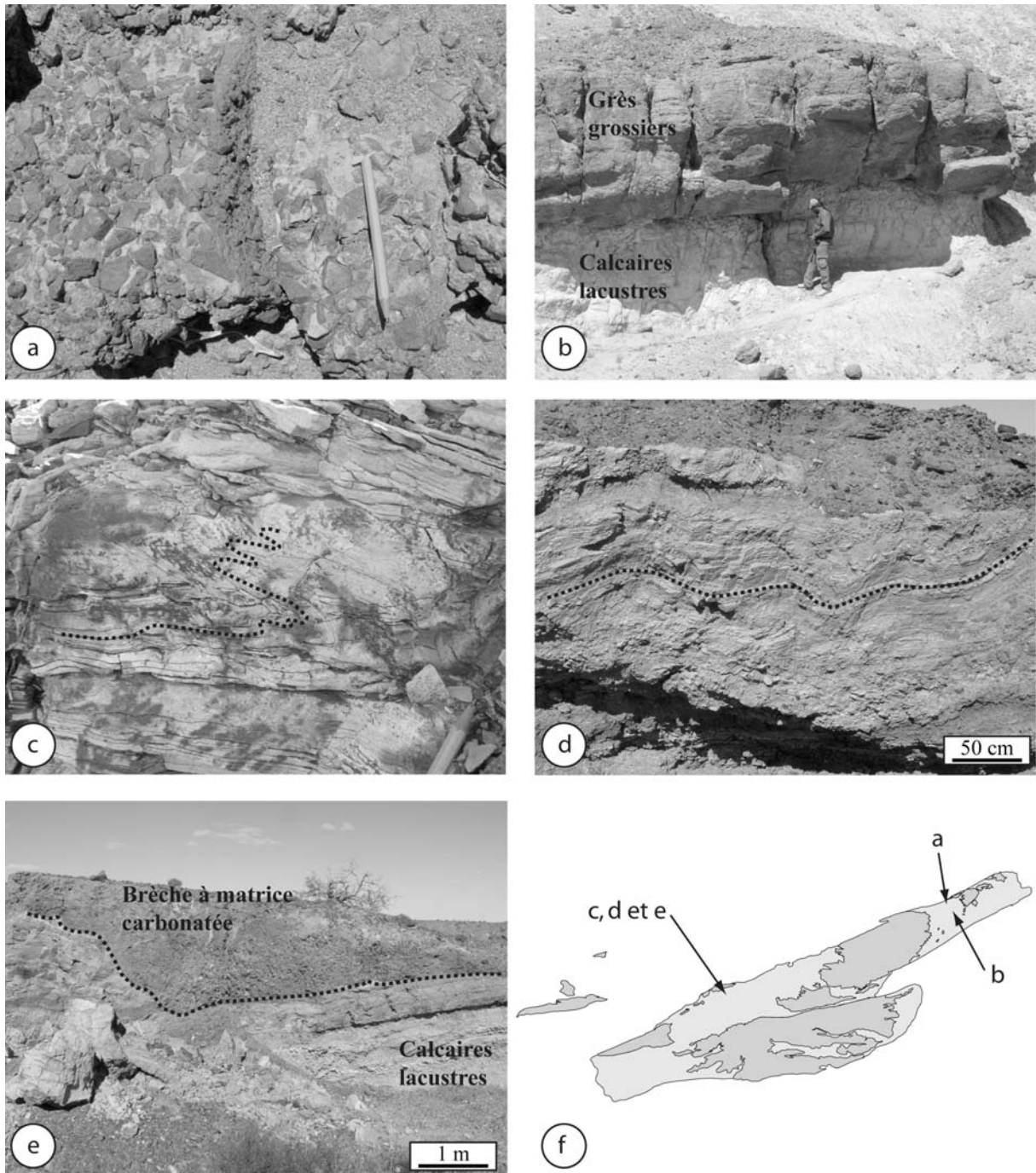
Fig. 6.20 : Principaux faciès sédimentaires de la Formation de Tsagaantsav. (a) Brèche sédimentaire à matrice carbonatée et aux éléments anguleux de schistes et de roches volcaniques basiques. (b) Alternance de niveaux de grès ocre et de calcaire lacustre blanchâtre. (c) Niveau de calcaire lacustre affecté par des plis gravitaires centimétriques. (d) Plis gravitaires métriques affectant des calcaires lacustres. (e) Chenal rempli par des brèches sédimentaires et montrant une base érosive sur les niveaux de calcaire lacustre. (f) Localisation des photographies. En gris foncé : les roches du socle. En gris clair : le domaine où affleure la Formation de Tsagaantsav.
