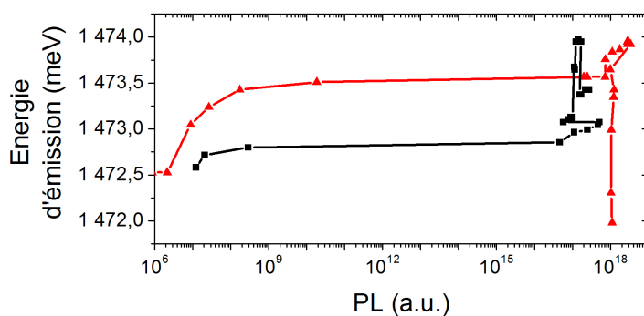
FIGURE 2.24 – Énergie des photons émis par un micropilier de diamètre \phi = 4\mu m présentant un désaccord de \delta = -1.16 meV en fonctions de l'intensité de l'émission pour une excitation non résonante E_{pompe} = 1.530 eV (carré noir) et à deux photons E_{pompe} = 738 meV (triangle rouge)
