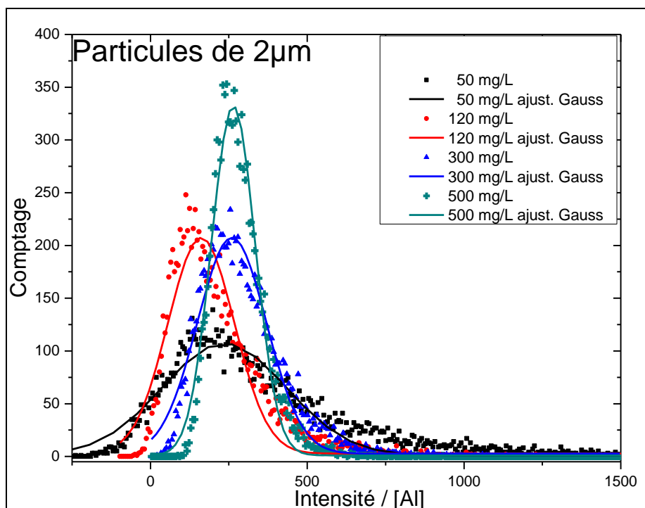
Figure III-1-8 : Histogrammes des intensités normalisées par la concentration en Al total pour des suspensions de particules d' Al_2O_3 avec diamètre de diamètre nominal de 2 \mu m à différentes concentrations (50, 120, 300, 500 ppm) et ajustées par un lissage gaussien.
