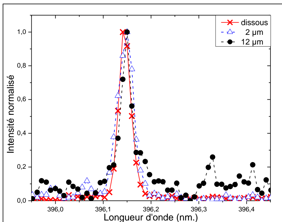
Figure III-1-3 : Comparaison des profils de la raie d'émission de l'Al dissous et des suspensions de particules de diamètres nominaux de 2 µm et 12 µm à la même concentration en Al de 300 mg/L.
