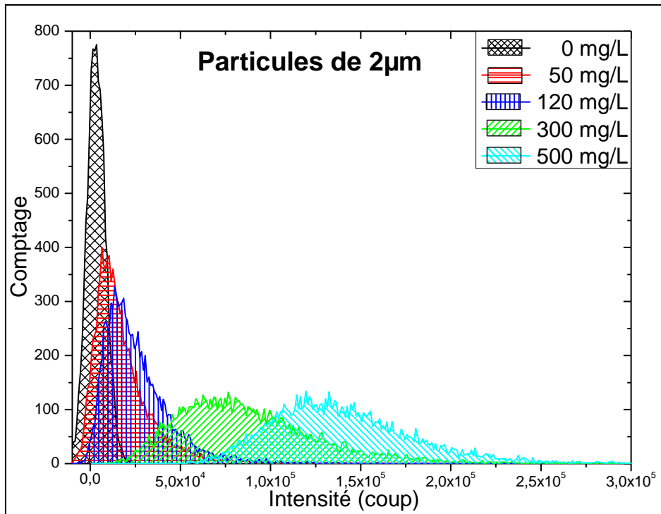
Figure III-1-7 : Histogramme des intensités obtenues pour différentes concentrations en Al total pour des suspensions de particules d' Al_2O_3 de diamètre nominal de 2 \mu m. Les 10 000 tirs sont classés dans 600 canaux.
