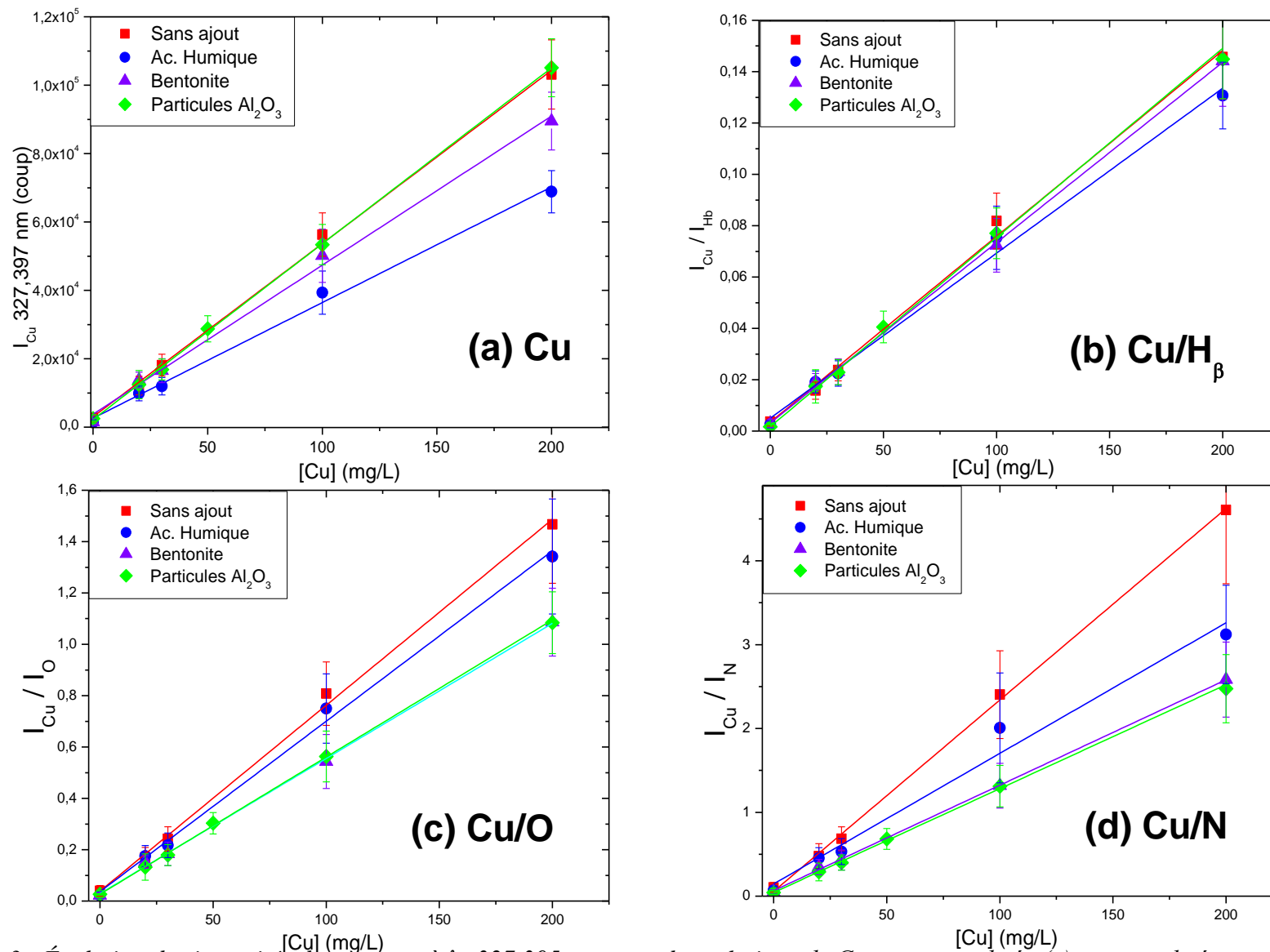
Figure III-2-3 : Évolution des intensités des signaux à \lambda=327,395 nm pour des solutions de Cu non normalisée (a) et normalisées par l'intensité des signaux H β (b), O (c) et N (d) dans des eaux avec et sans ajouts d'acide humique, de bentonite et de particules d'alumine.
