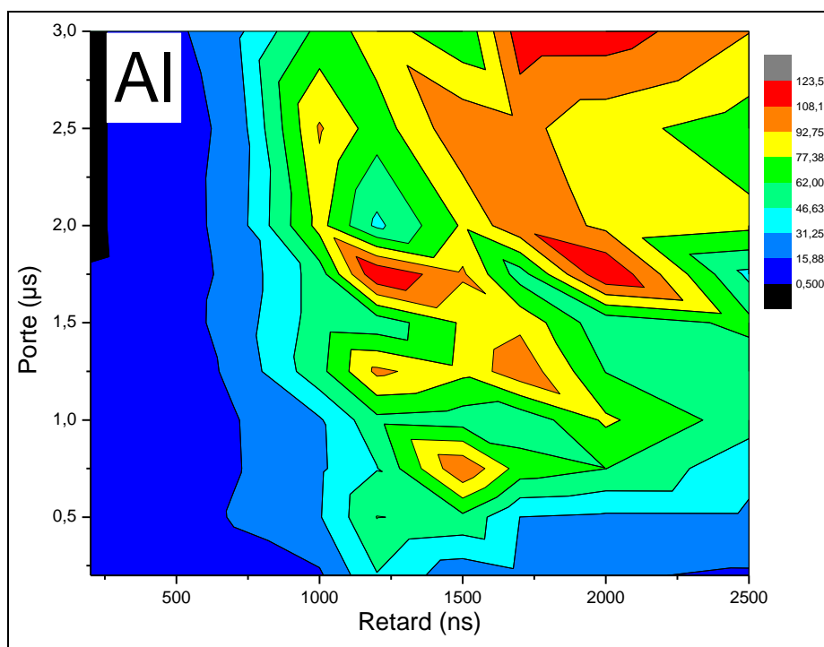
Figure II-9 : Cartographie du rapport S/B des paramètres « porte » et « retard » pour le meilleur rapport signal/bruit dans le cas de l'Al à \lambda=396,152 nm.
