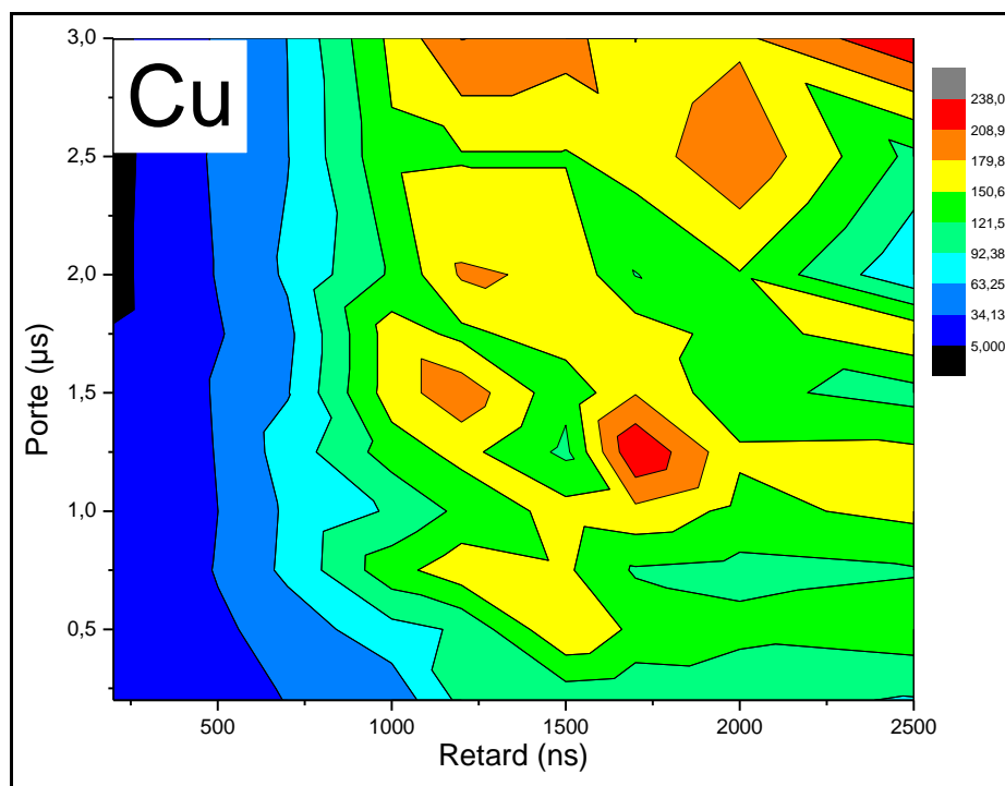
Figure II-10 : Cartographie du rapport S/B des paramètres « porte » et « retard » pour le meilleur rapport signal/bruit dans le cas du Cu à \lambda=327,395 nm.
