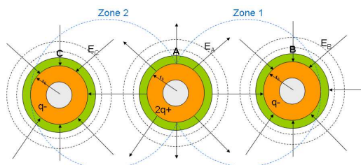
figure 3-16: Champ électrique produit par 3 TSV
