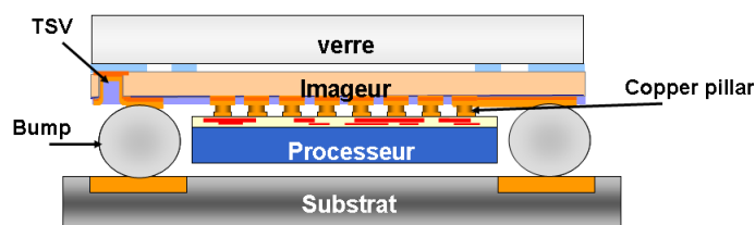
figure 0- 3: Exemple d'architecture d'un imageur en conception 3D
