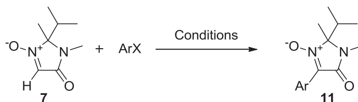
Schéma 47 Réaction envisagée pour l'arylation de la MiPNO.
