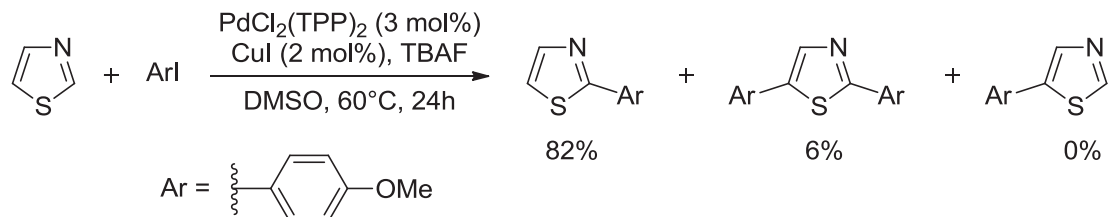
Schéma 79 Arylation directe sélective d'un thiazole par ajout de cuivre catalytique.
