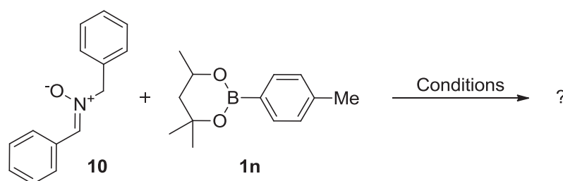
Schéma 37 Réactifs modèles pour l'addition d'arylboration sur des nitrones.
