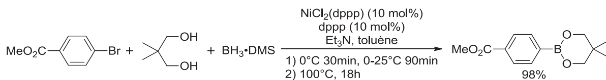
Schéma 16 Borylation catalysée au nickel.
