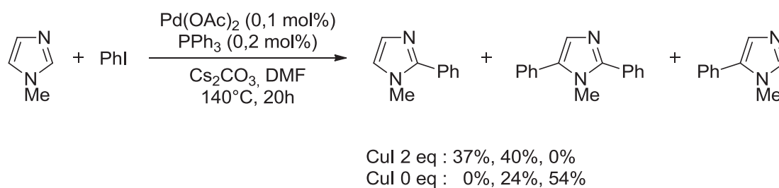
Schéma 62 Effet de CuI sur une arylation directe d'imidazole.
