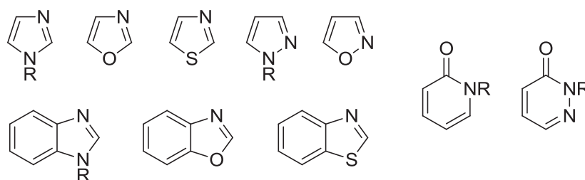
Figure 11 Exemples de structures hétérocycliques étudiées.
