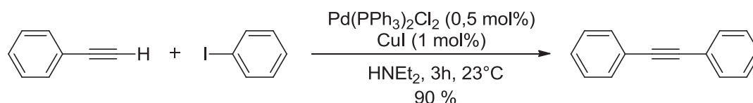
Schéma 52 Arylation d'alcyne terminal catalysée par le couple Palladium/Cuivre (Sonogashira, 1975).
