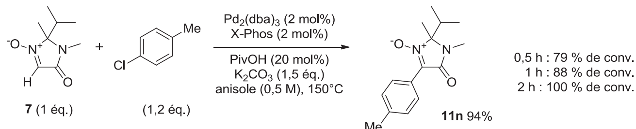
Schéma 91 Arylation avec le 4-chlorotoluène.
