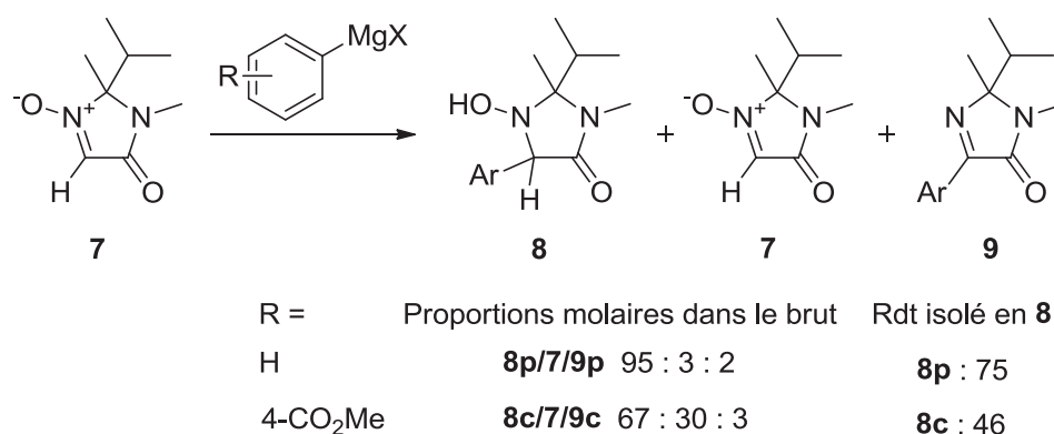
Schéma 31 Addition d'arylmagnésiens sur MipNO.
