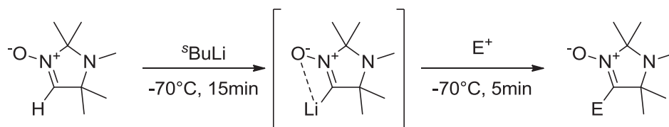
Schéma 96 Métaallation puis addition électrophile d'une nitronne (Grigor'ev, 2001).
