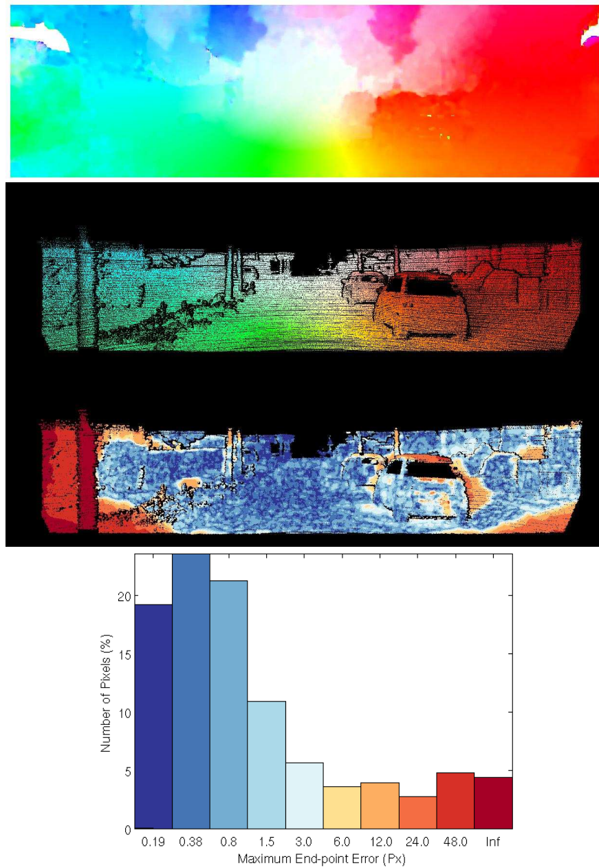
Figure 3.20 – Résultat FOLKI2 sur image 17 de la base d'apprentissage de Kitti. De haut en bas : une des deux images du couple traité ; resultat FOLKI1 et vérité terrain (même échelle de couleur) ; carte d'erreur avec une échelle de couleur associée aux cases de l'histogramme présenté en bas.
