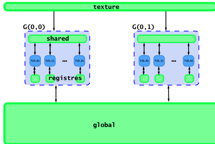
Figure 2.8 – Schéma du modèle mémoire
