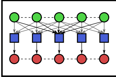
Figure 2.12 – Schéma de principe d'un filtre FIR
