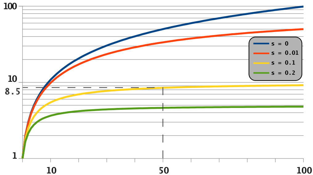
Figure 2.25 – Loi d'Amdhal : évolution de l'accélération de l'exécution d'un algorithme ayant une portion de code séquentiel s de 0%, 1%, 10% et 20% en fonction du nombre de processeurs.
