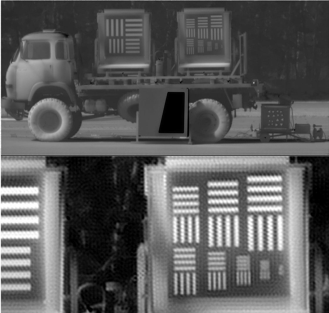
Figure 4.31 – SR quadratique pour une PSF plus étroite que l'estimée ( \sigma = 0.330 ) et un facteur de SR très élevé ( \times 15 ). L'image de dessous est un extrait de celle de dessus, pour voir le phénomène de damier. Les paramètres de traitement sont donnés en Table B.3.
