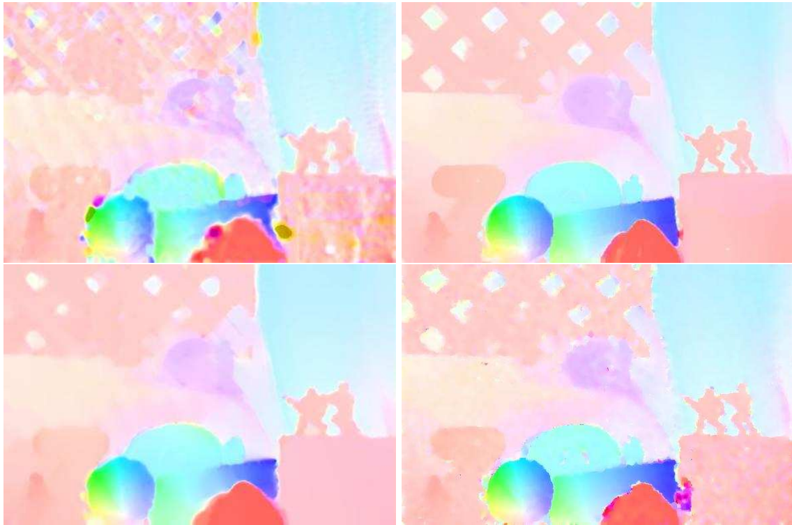
Figure 3.13 – Exemple Army du site Middlebury. L'image et la vérité terrain sont présentées en Figure 3.1. En haut, résultat FOLKI (fenêtre gaussienne, d'écart-type 2.5 pixels) et Anisotropic Huber L1 (citeWerlberger10); en bas, résultats d'extensions de FOLKI : à gauche approche MCLG ([Fezzani, 2011]), à droite, FOLKI avec les modifications proposées dans la suite de cette section. Les images de flot utilisent le codage en couleur du site Middlebury avec un déplacement max de 5 pixels.
