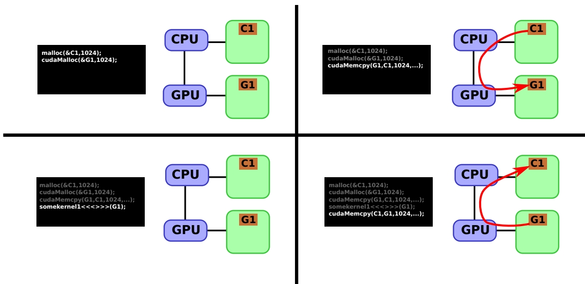
Figure 2.6 – Déroulement d'un traitement effectué par le GPU de haut en bas et de gauche à droite. On commence par allouer de la mémoire sur le GPU (G1) et le CPU (C1), on copie ensuite les données vers le GPU, on exécute la fonction sur le GPU, puis au besoin on rapatrié sur le CPU le résultat.
