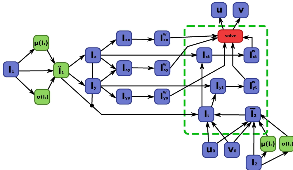
Figure 3.10 – Schémas de l'algorithme FOLKI avec normalisation des fenêtres pour la version approximée rapide, les opérations supplémentaires par rapport à l'algorithme FOLKI original sont en vert.
