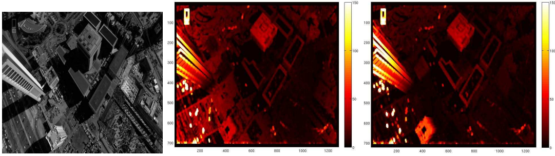
Figure 3.27 – Flot résiduel cumulé après recalage paramétrique d'une série d'images (séquence Dubai). A gauche, image d'origine, au milieu : recalage par primitive et estimation robuste, à droite : approche par recalage dense et régression robuste proposée ici.
