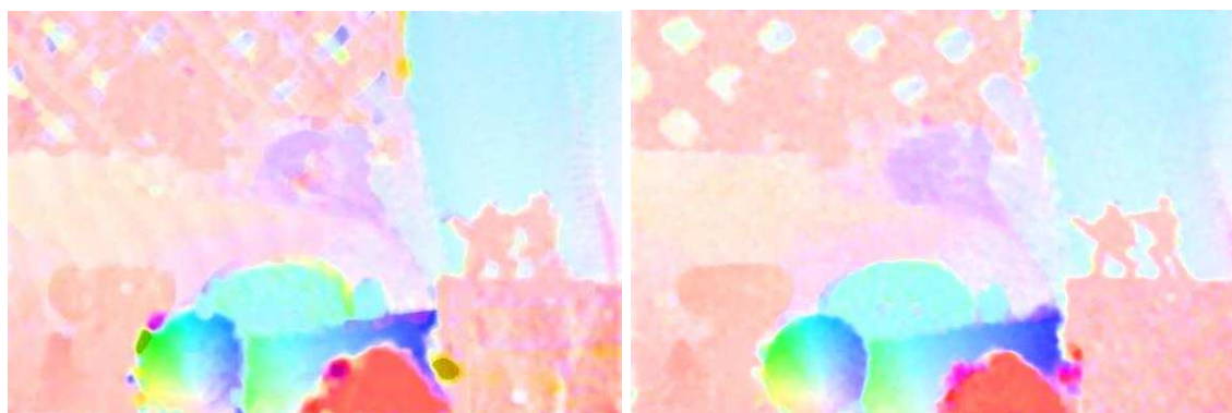
Figure 3.15 – Réduction de l'empâtement des objets par la transformée Rank. A gauche, résultat de FOLKI (fenêtre gaussienne d'écart-type 2.5) sur l'exemple Army ; à droite, même algorithme appliqué à l'image issue d'un Rank-4. Les images de flot utilisent le codage en couleur du site Middlebury avec un déplacement max de 5 pixels.
