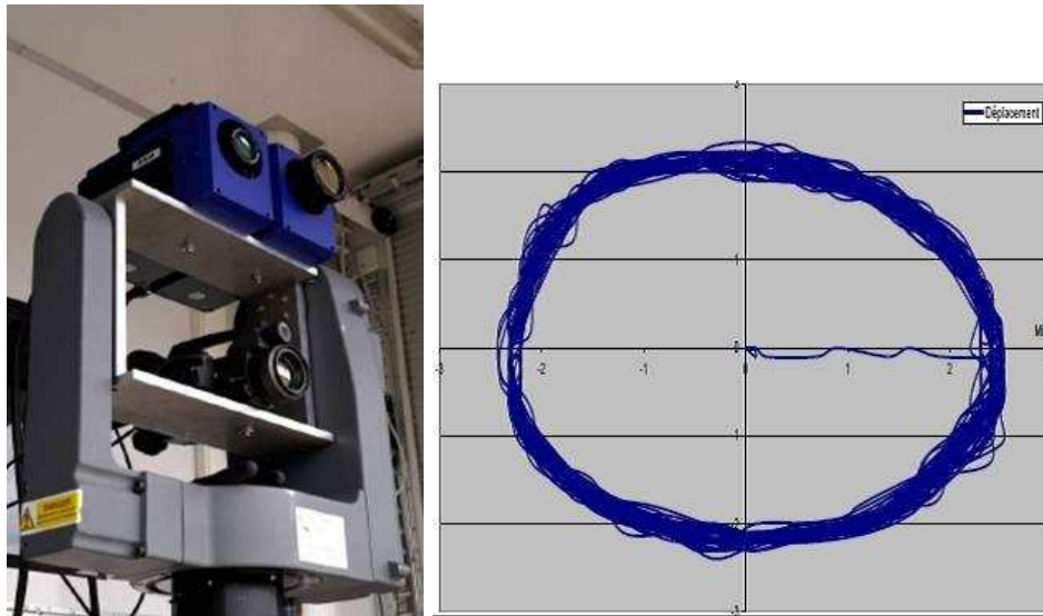
Figure 4.24 – Dispositif d'acquisition mis en place par la DGA pour l'évaluation d'algorithmes de SR sur images réelles Infra-rouges (images extraites de [Weißet al., 2012]). Trois caméras IR sont montées sur un support mobile : celle dont nous traitons les images dans cette section est une caméra bolométrique FLIR SC660 de résolution 640 \times 480 pixels. Le support est animé de mouvements de précession tel que celui présenté à droite.
