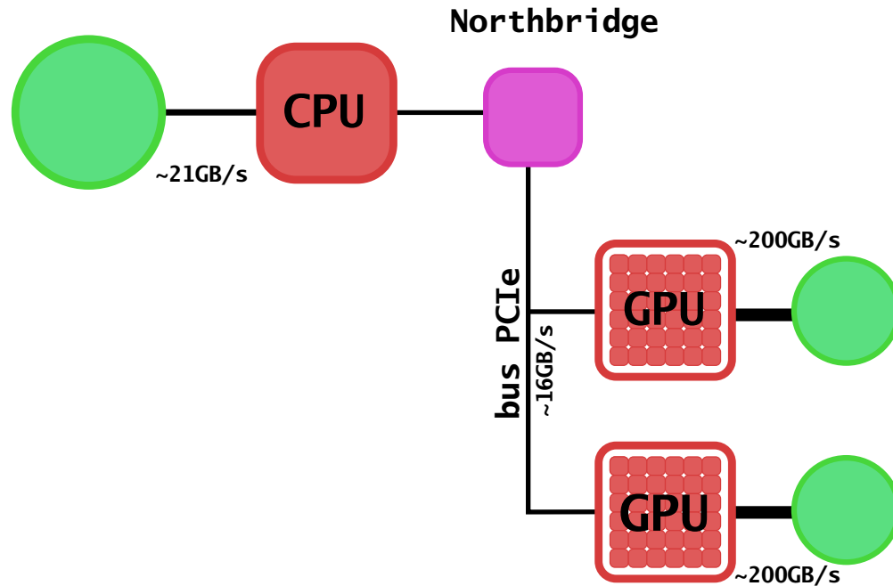
Figure 2.5 – Structure générale de l'architecture d'un PC moderne
