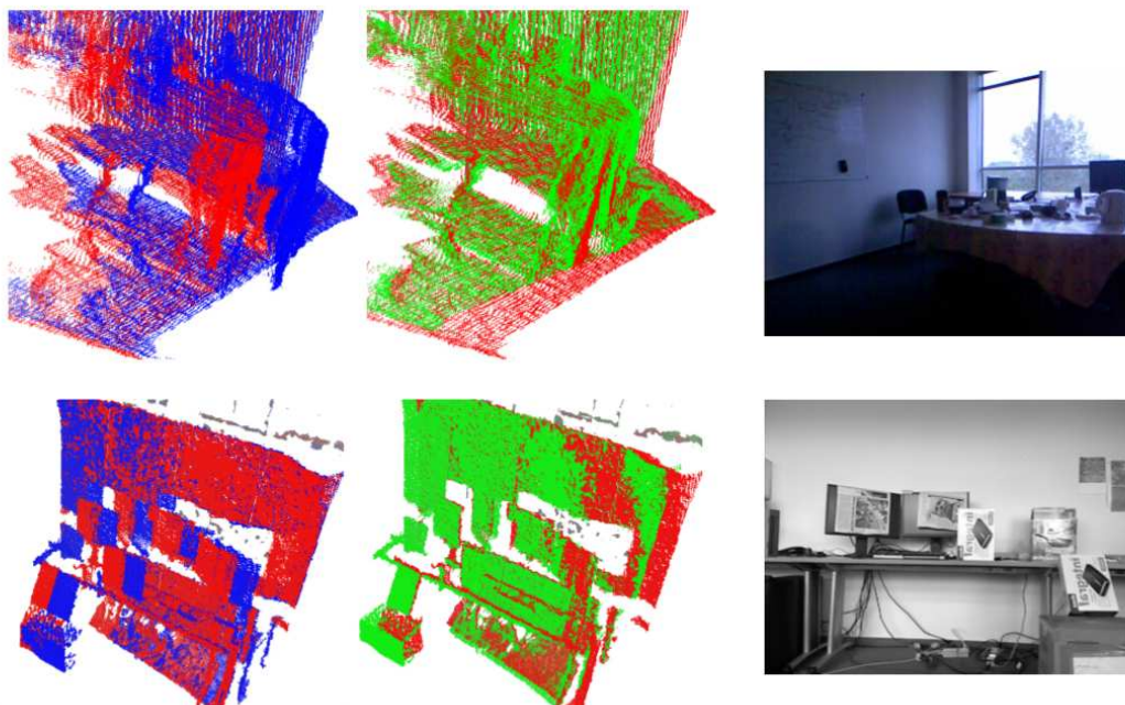
Figure 5.2 – Résultat d'un calcul de pose par un algorithme massivement parallèle utilisant la correspondance de segments extraits des images de profondeur fournies par un Kinect (extrait de [Israël and Plyer, 2013])
