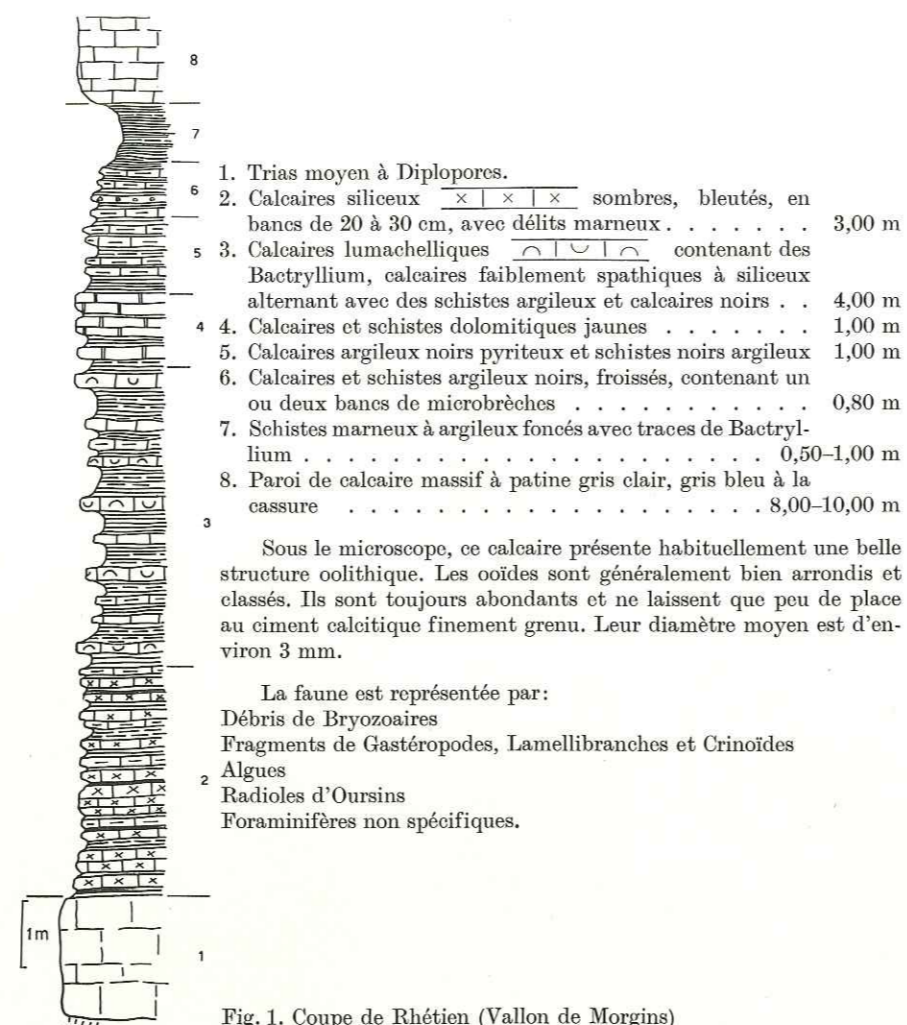
Fig. 1. Coupe de Rhétien (Vallon de Morgins)
