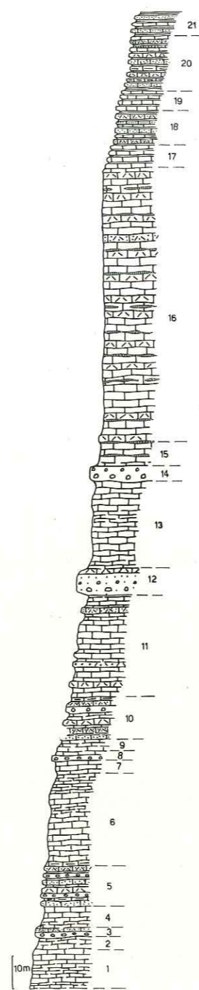
Fig. 13. Coupe de la Brèche supérieure (ravin de la Forge)
