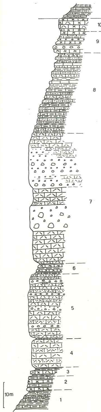
Fig. 7. Coupe de la Brèche inférieure dans le ravin de Cornillon
