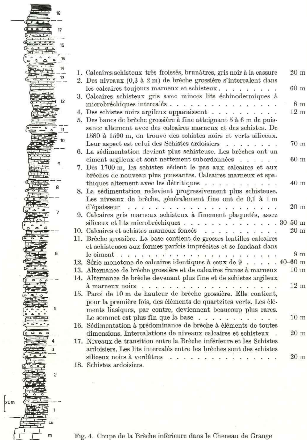
Fig. 4. Coupe de la Brèche inférieure dans le Cheneau de Grange
