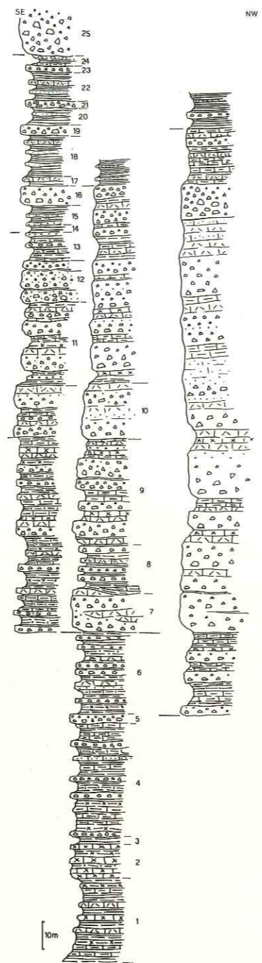
Fig. 6. Coupe de la Brèche inférieure dans le versant N du Mont de Grange
