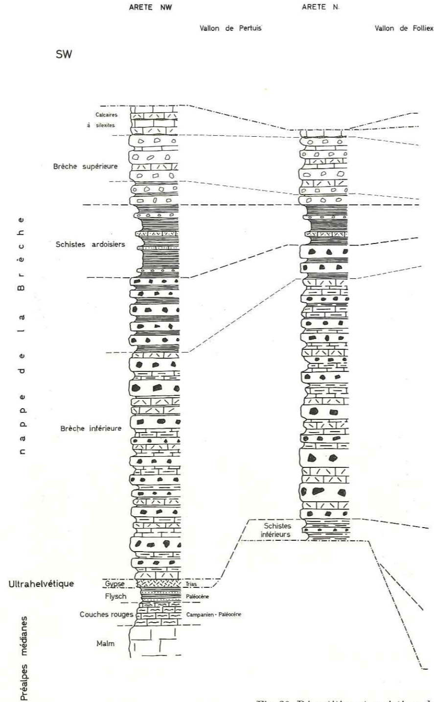
Fig. 20. Répartition et variations des faciès
