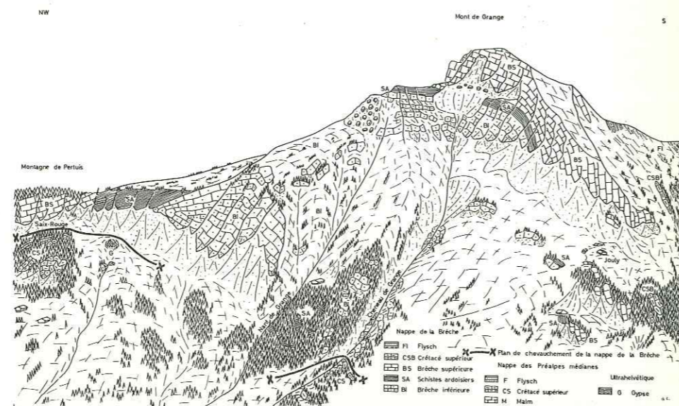
Fig. 24. Versant SW du Mont de Grange
