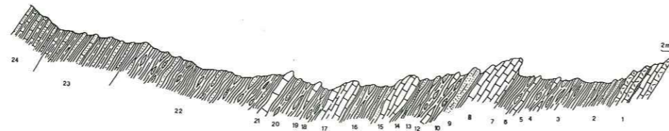
Fig. 17. Passage Brèche supérieure-Flysch (Les Mattes)
