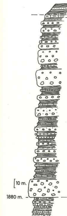
Fig. 5. Partie supérieure de la Brèche inférieure dans le Nant de Grange
