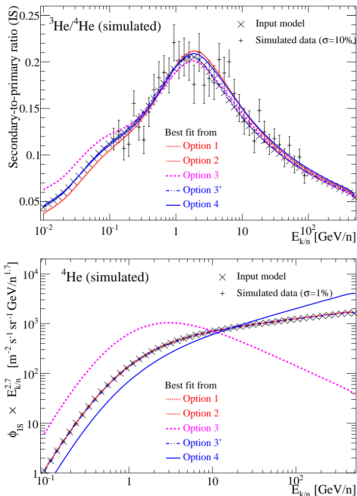
FIGURE 4.9 – Analyse des données simulée du rapport {}^3\text{He}/{}^4\text{He} (en haut), du flux {}^3\text{He} multiplié par E_{k/n}^{2.7} (en bas) en utilisant le modèle II (symboles \times ). Les différentes courbes de meilleur ajustement correspondent aux différentes options données dans la section 4.4.2 et les valeurs des paramètres correspondants sont données dans la table 4.4. Figures issues de [51].
