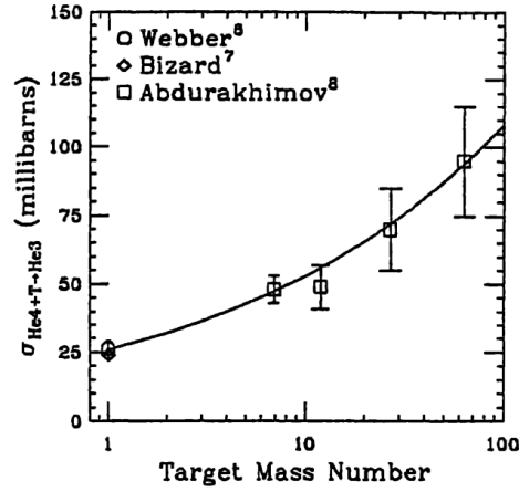
FIGURE 4.4 – Compilation des sections efficaces de production de {}^3\text{He} en fonction du numéro atomique de la cible tirée de [58]. Ces sections efficaces peuvent être paramétrées en fonction de la section efficace sur cible d’hydrogène comme \sigma^{P+T \rightarrow F} = \sigma^{P+p \rightarrow F} A_T^{0.31} .
