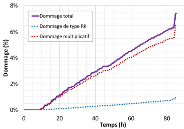
Figure II-67 : Simulation du domage total et des deux types de dommages pendant l'essai 150H
