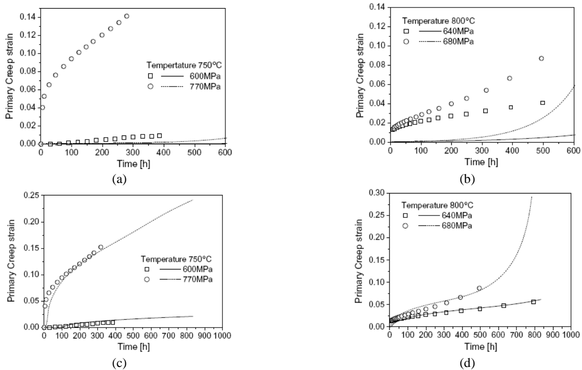
Figure II-8 : Prédictions de déformation en fluage à 750 et 800°C pour une orientation cristalline proche [001] (lignes), comparées aux courbes expérimentales (points) en considérant les mécanismes de glissement de la matrice uniquement (a et b) et en considérant les mécanismes de glissement de la matrice et des précipités (c et d) [60]
