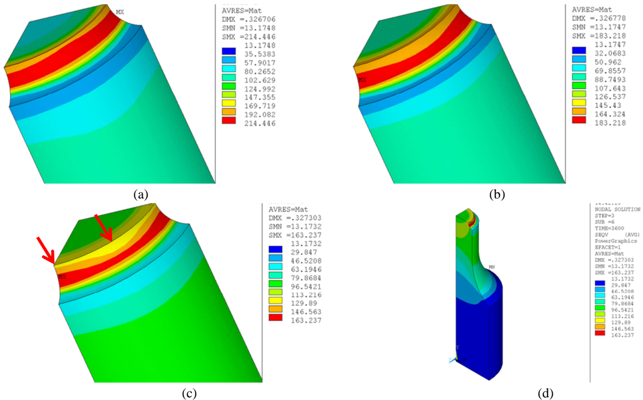
Figure A-5 : Contrainte de Von Mises au niveau de l'entaille pour – (a) 36 secondes ; (b) 6 minutes ; (c) 1 heure ; (d) vue d'ensemble
