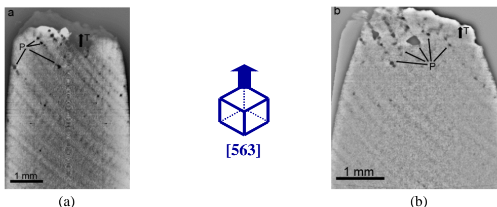
Figure I-121 : Microstructures observées par tomographie à rayons X après essais de fluage à 1050°C et 140MPa – (a) isotherme, (b) tir OEI 30s sans préfluage [73]
