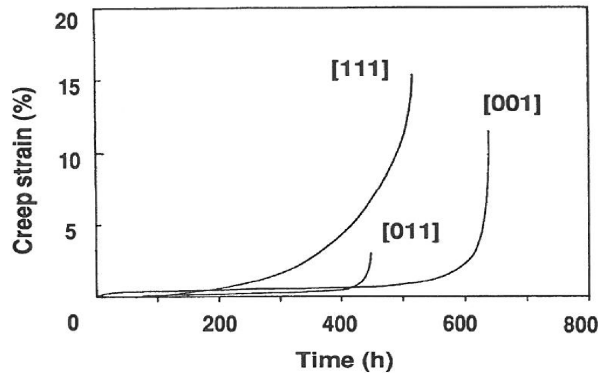
Figure I-22 : Courbes de fluage à 1050°C et 120 MPa sur AM3 pour 3 orientations cristallines– [001], [011] et [111] [35]
