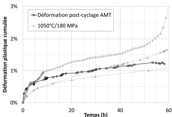
Figure II-62 : Comparaison du post-fluage expérimental de l'essai AMT (1055°C/180 MPa) et des essais isothermes d'identification du modèle (1050°C/180 MPa)
