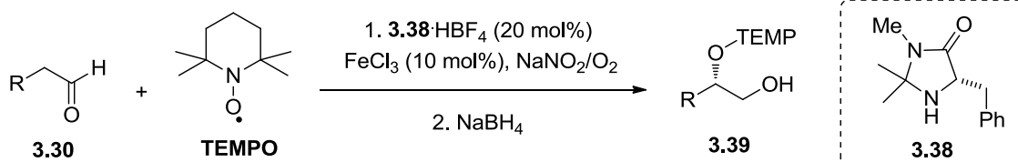
Schéma 116 : \alpha -oxyamination asymétrique d'aldéhydes en présence de Fe(III)
