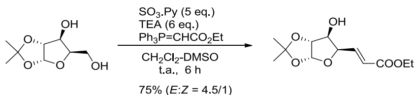
Schéma 17 : Processus tandem oxydation/oléfination à l'aide de \text{SO}_3\cdot\text{Py}
