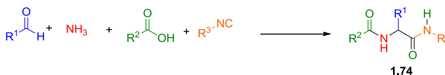
Schéma 31 : Ugi-4CR à partir d'ammoniac
