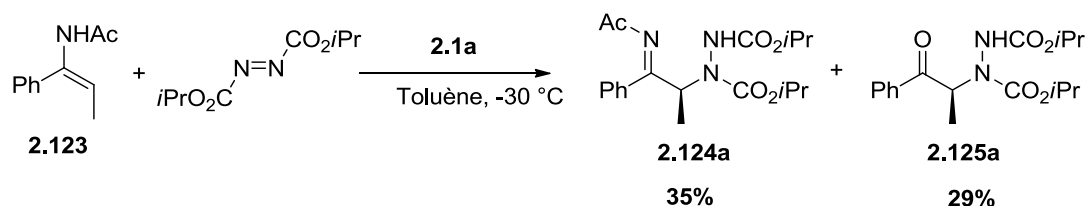
Schéma 98 : 1 er essai d' \alpha -hydratation catalysée par un acide phosphorique
