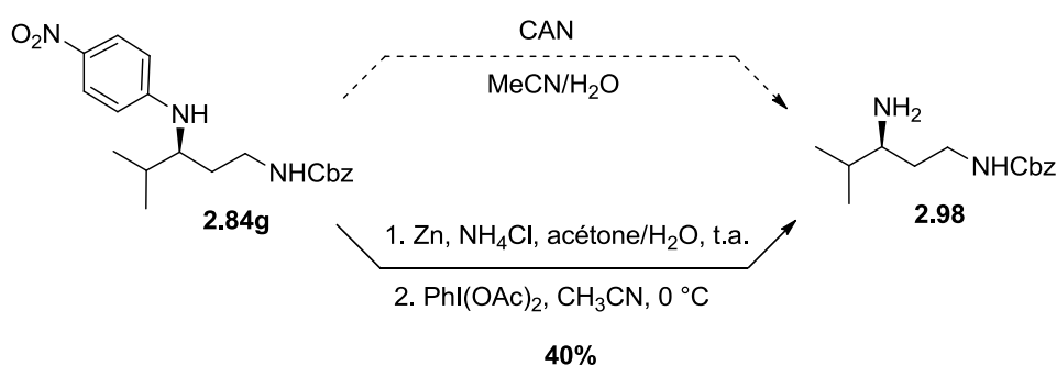
Schéma 90 : Déprotection du groupement p -nitrophényle
