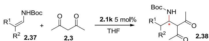
Schéma 65 : Réaction de Mannich à partir d'énecarbamates
