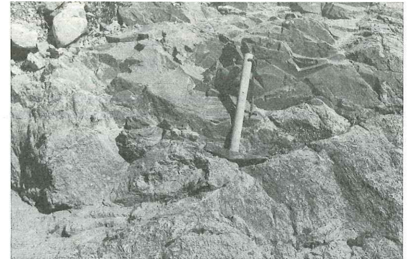
FIG. 28. — « Inclusion » de sédiments (plus ou moins albitisés, à stilpnomélane parfois) dans le gabbro. La Mouille-Ronde ( point 15 ).
