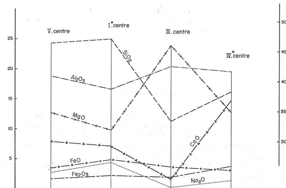
FIG. 40. — VARIATIONS DES TENEURS EN PRINCIPAUX OXYDES DANS LA PARTIE CENTRALE DE QUATRE TYPES BIEN DISTINCTS D'OPHIOPHÉRITES.
