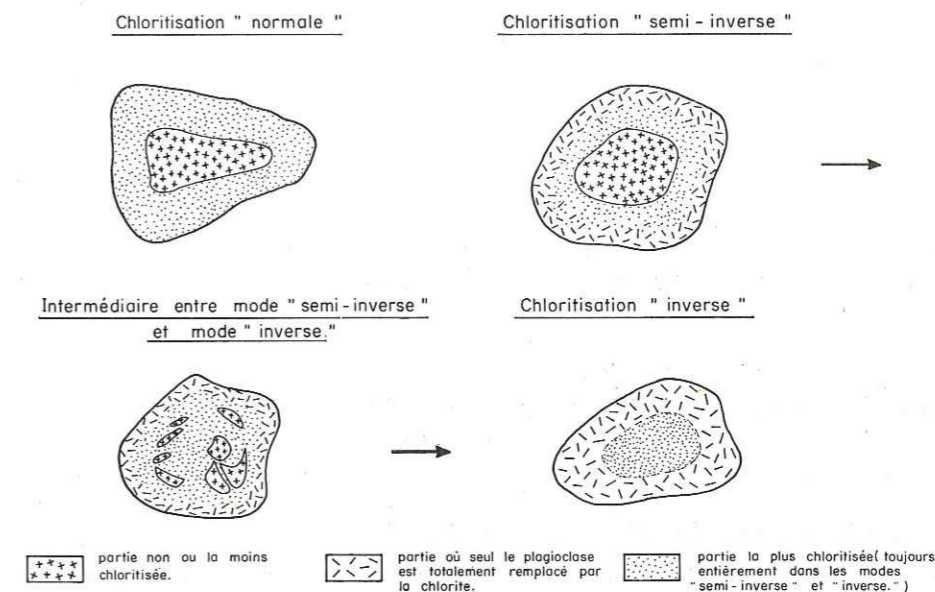
FIG. 32. — REPRÉSENTATION SCHÉMATIQUE DES TROIS PRINCIPAUX MODES DE CHLORITISATION DES OPHISPHÉRIDES.
