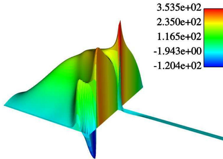
FIG. 3.8 – \rho v y -momentum map
