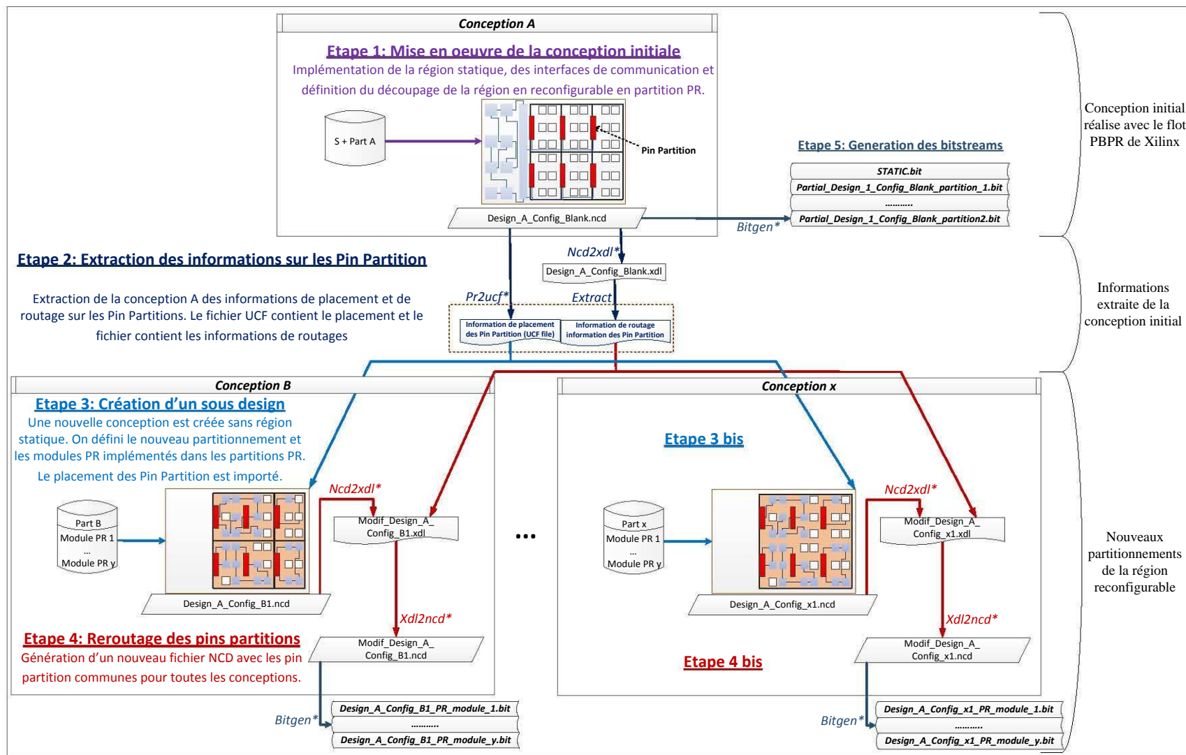
FIGURE 4.10 – Flot de conception pour la conception d'une architecture avec des partitions PR adaptable. *Fonction native de Xilinx.
