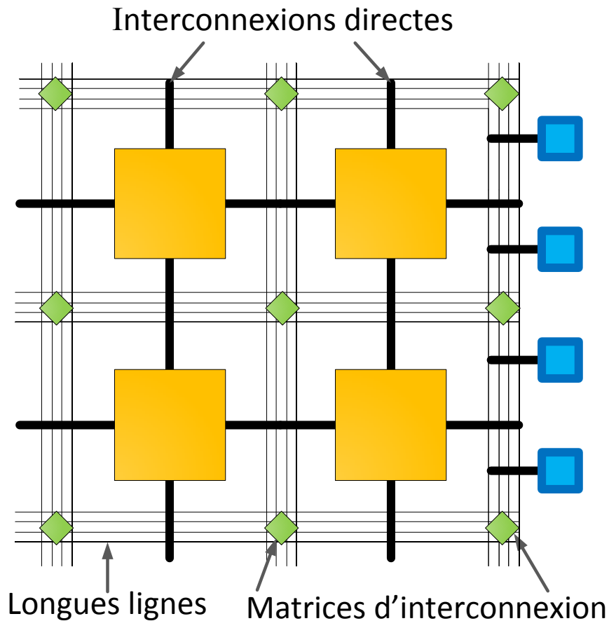
FIGURE 1.5 – Interconnexion interne d'un FPGA.
