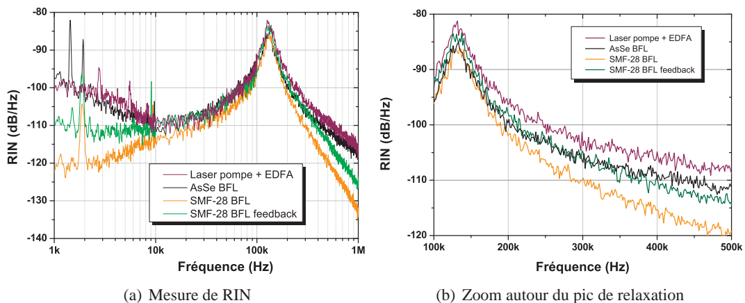
FIGURE 4.24 – Comparaison du RIN entre une cavité Brillouin faite de fibre silice classique et une autre faite de fibre AsSe.
