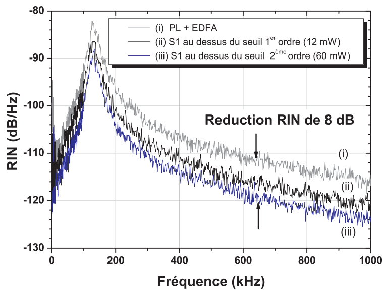
FIGURE 4.37 – RIN de la composante S1 pour deux différentes puissances pompe. Le bruit d'intensité de la composante de S1 peut être réduite en créant une composante S2 dans la cavité. Ainsi le bruit issu de la pompe est transféré vers la composante S2, ce qui diminue le bruit de S1.
