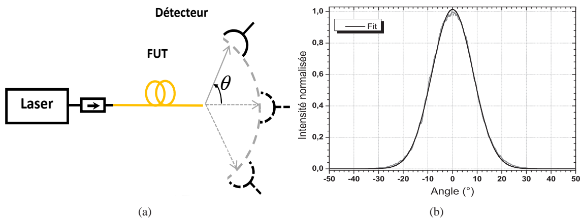
FIGURE 2.12 – (a) Schéma de principe de la mesure d'aire effective d'une fibre quelconque et (b) exemple de mesure obtenu par le banc entre [-50^{\circ} à 50^{\circ}] .
