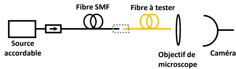
FIGURE 2.13 – Schéma de principe pour l'analyse modale d'une fibre quelconque.
