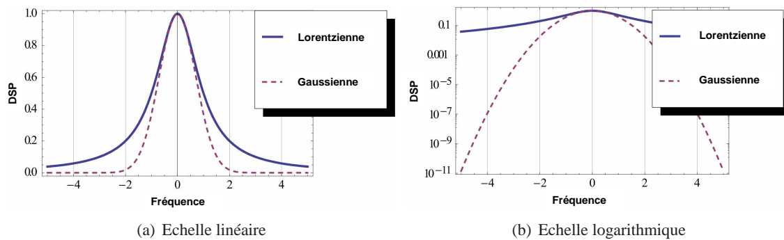
FIGURE 1.17 – Comparaison Lorentzienne/Gaussienne.
