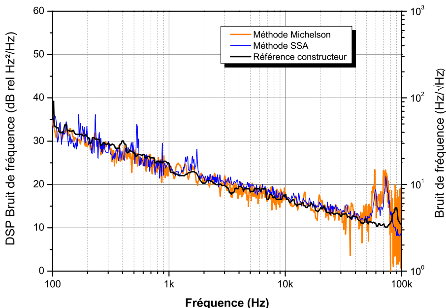
FIGURE 1.31 – DSP de bruit de fréquence du laser Koheras Adjustik mesurée avec les deux méthodes. Méthode Michelson : méthode avec discriminateur de fréquence et Méthode SSA : méthode auto-hétérodyne corrélée.
