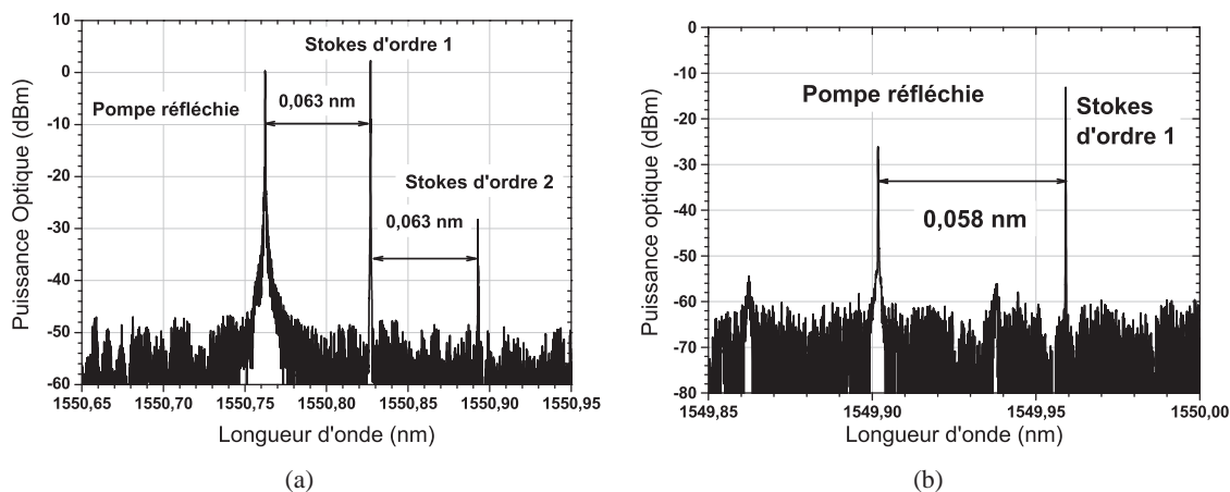
FIGURE 3.18 – Spectre optique de la composante rétrodiffusée dans une fibre (a) à cœur suspendu AsSe de 1 mètres pour une puissance injectée de 27 dBm et (b) microstructurée GeAsSe de 3 mètres pour une puissance injectée de 12 dBm.
