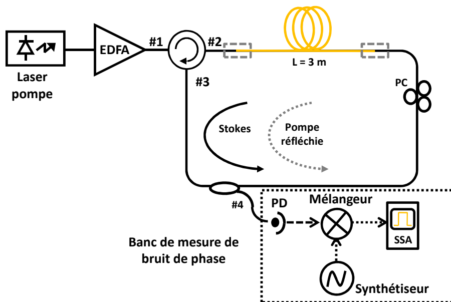
FIGURE 5.6 – Génération d'un signal optique RF à partir du BFL. Le battement entre une onde pompe et sa composante Stokes est "down-converted" en utilisant un mélangeur et un synthétiseur afin de pouvoir effectuer la mesure avec notre analyseur de bruit de phase.
