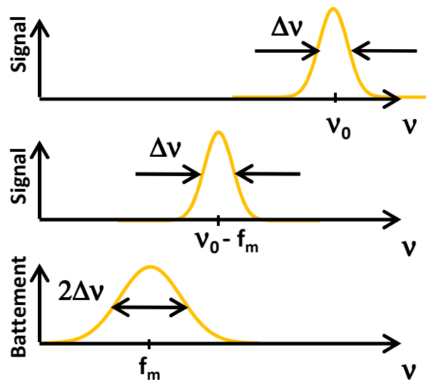
FIGURE 1.25 – Battement auto-hétérodyne.
