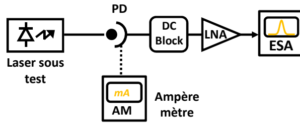
FIGURE 1.18 – Banc de mesure de bruit d’intensité.
