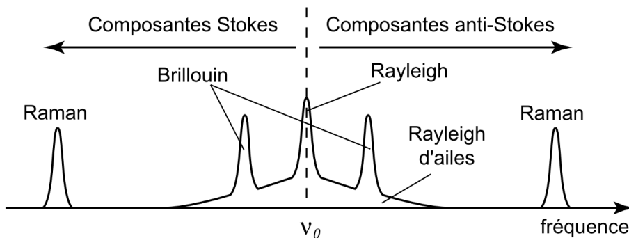
FIGURE 3.1 – Spectre typique de lumière diffusée spontanément par un milieu diffusant quelconque.
