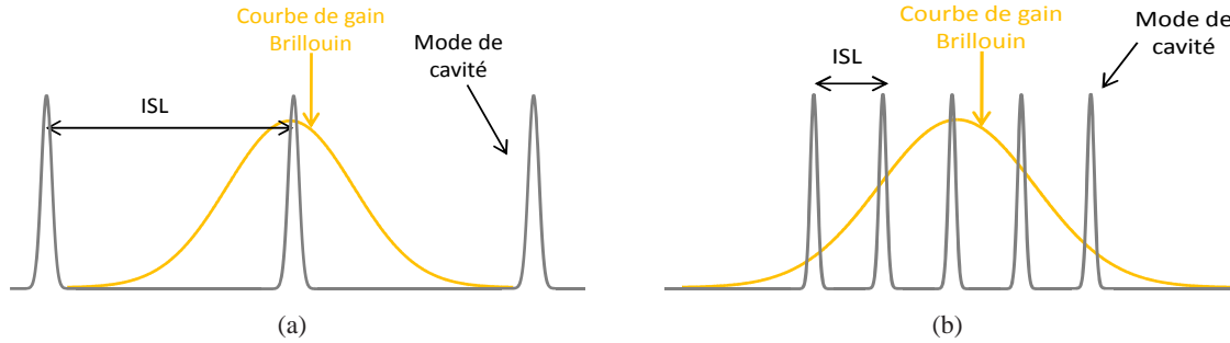
FIGURE 4.1 – Répartition des modes de cavités sous la courbe de gain Brillouin.
