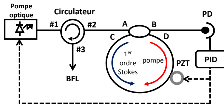
FIGURE 4.2 – BFL en anneau avec pompe résonante dans la cavité. PID : Régulateur Proportional Intégral Dérivé, PZT : Céramique piézoélectrique.
