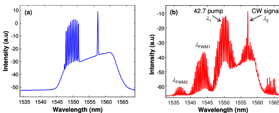
FIGURE 2.18 – Le mélange à quatre ondes dans une fibre AsSe MOF.
