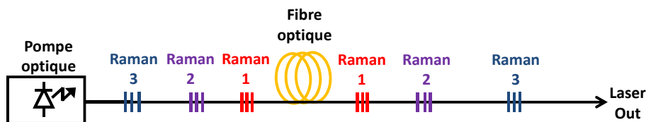
FIGURE 1.10 – Cavité laser basée sur la diffusion Raman stimulée.
