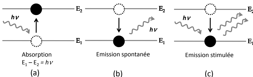
FIGURE 1.2 – (a) Absorption, (b) émission spontanée et (c) émission stimulée.
