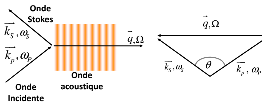
FIGURE 3.2 – Représentation schématique de la diffusion Brillouin spontanée
