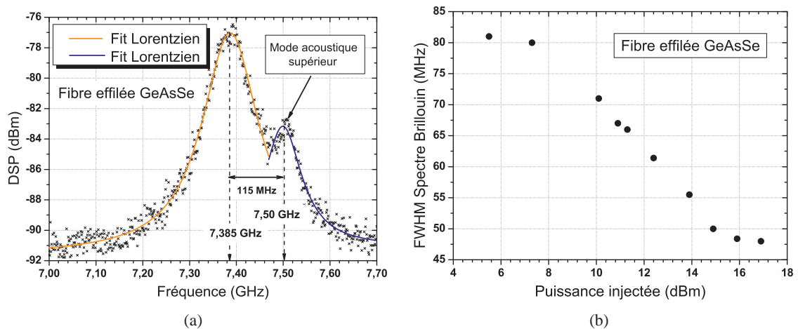
FIGURE 3.26 – (a) Spectre de diffusion Brillouin pour une puissance injectée de 13,4 dBm (b) FWHM du pic principal en fonction de la puissance injectée dans une fibre microstructurée GeAsSe de diamètre 1,6 \mu\text{m} . Le fit Lorentzien a été réalisé sur l'ensemble du spectre dû au mode fondamental acoustique. Les valeurs FWHM du spectre Brillouin mesurées prennent donc en considération les deux modes de biréfringence de la fibre.
