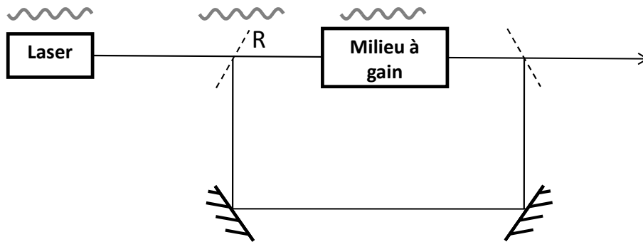
FIGURE 4.15 – Représentation schématique des différentes sources de bruit d'un laser
