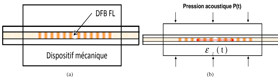
FIGURE 4 – Sous l'effet d'une pression acoustique, le dispositif mécanique déforme axialement le DFB FL; ce qui résulte en un décalage de sa longueur d'onde d'émission.
