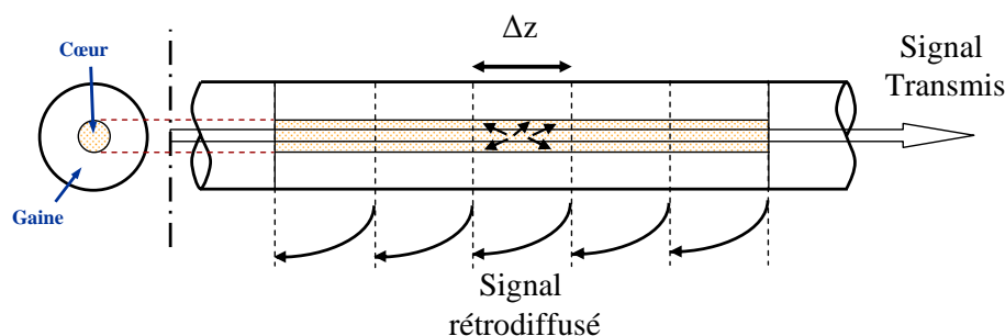
FIGURE B.1 – Illustration de la rétrodiffusion Rayleigh.
