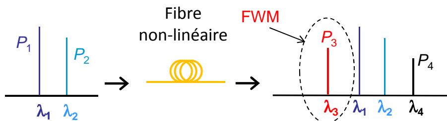
FIGURE 2.17 – Concept de base du mélange à quatre ondes.
