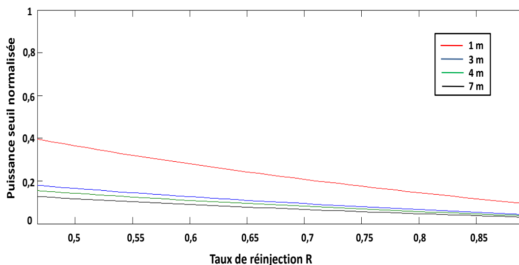
FIGURE 4.13 – Puissance laser seuil normalisée par rapport au taux de réinjection dans des cavités BFL pour différentes longueurs de fibre AsSe SC 5 (zoom sur la partie R = 0,5 à R = 0,9 ).
