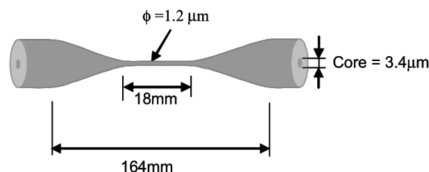
FIGURE 2.6 – Tapers avec un \gamma de 68\,000 W^{-1}.km^{-1} selon MÄGI.
