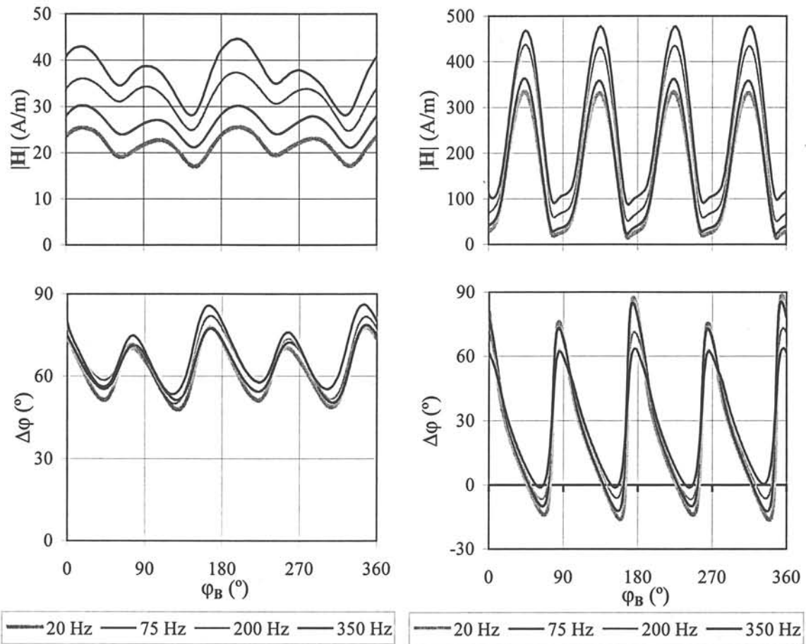
Figure III-23 : Variation de |\mathbf{H}| et de \Delta\varphi en fonction \varphi_B , fréquence variable : 20, 75, 200 et 350 Hz ; tôle FeNi
