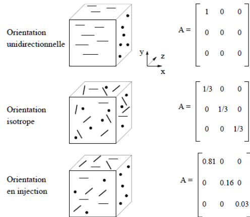
Figure A.6 : Exemples de tenseurs d'orientation \underline{\underline{a}}_2 pour différentes orientations théoriques. (Redjeb, 2007).
