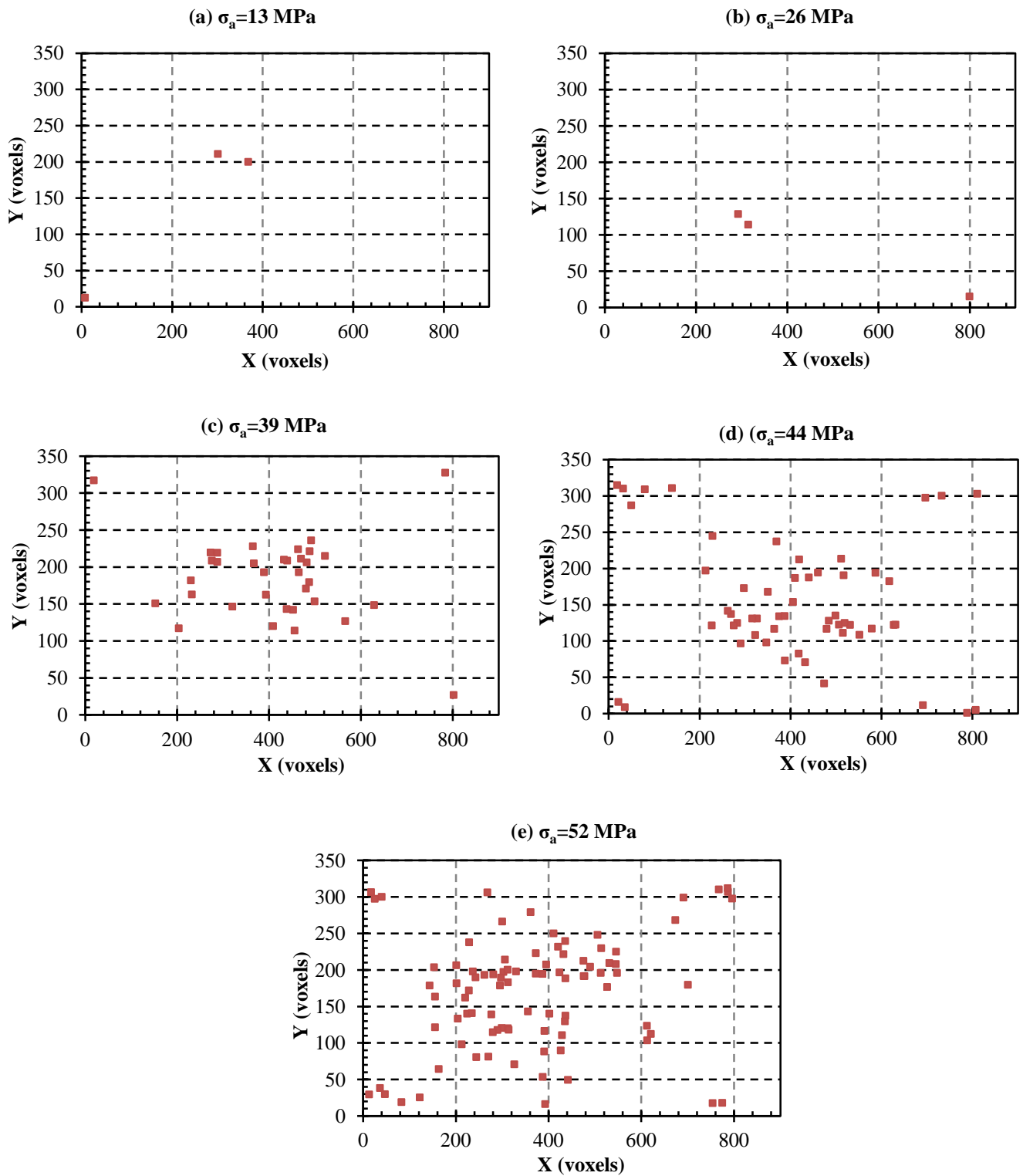
Figure 2.69 : Positions dans la section (\bar{X}; \bar{Y}) des défauts > 500 voxels pour les différentes amplitudes de contrainte.
