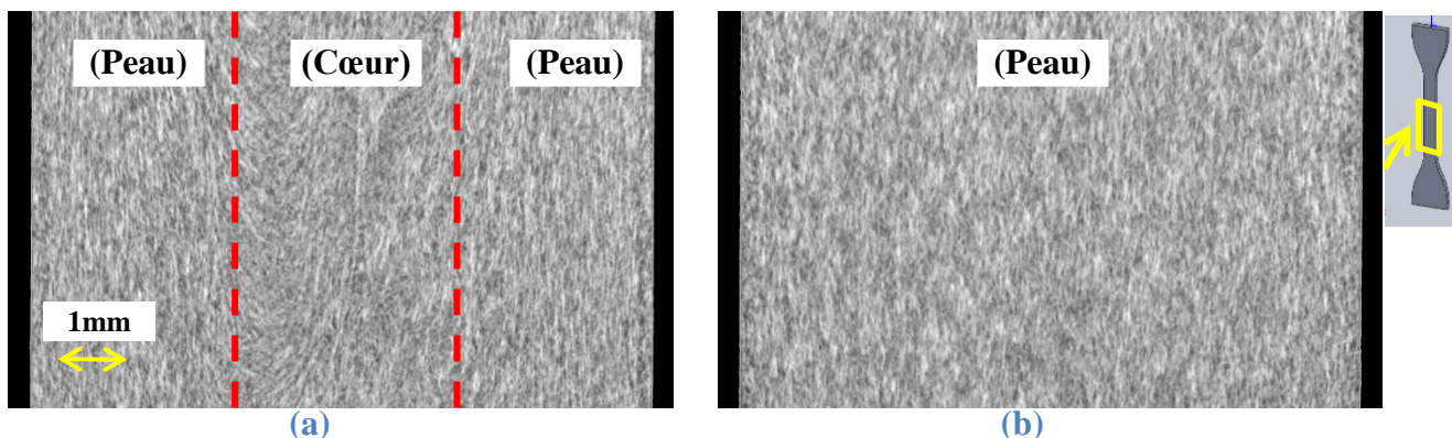
Figure 2.22 : ISO527 vue en coupe ( \vec{Y} ; \vec{Z} ) obtenue en MTRX ; (a) dans le plan médian de l'éprouvette ; (b) dans un plan intermédiaire
