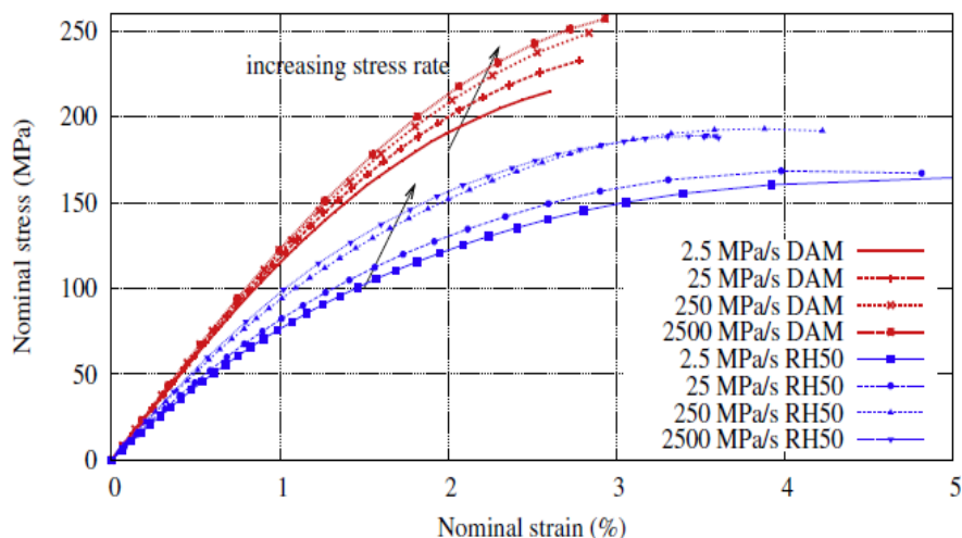
Figure 1.32 : (a) Courbes de traction-rupture à différentes vitesses de sollicitation sur un PA66GF35 DAM et RH50%. (Launay, 2011)
