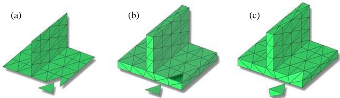
Figure 2.10 : Différents types de maillage du logiciel Moldflow®. (Source société Moldflow corporation)
