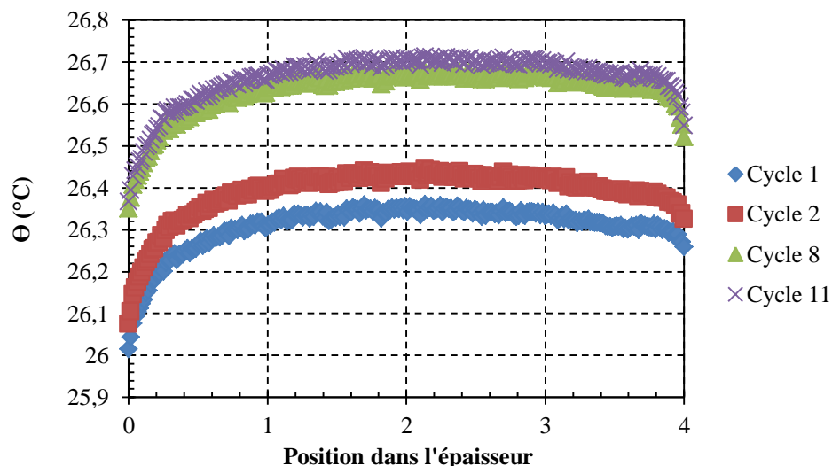
Figure 5.7 : Evolution de la température dans l'épaisseur d'une éprouvette ISO527 durant les premiers cycles d'auto-échauffement.
