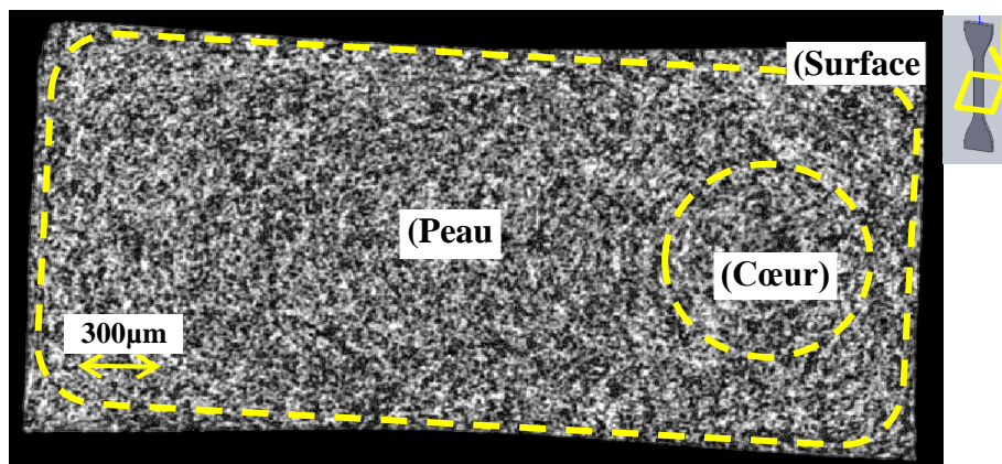
Figure 2.25 : H2 vue en coupe (\vec{X}; \vec{Y}) obtenue en MTRX et mise en évidence de la structure en « caisson »
