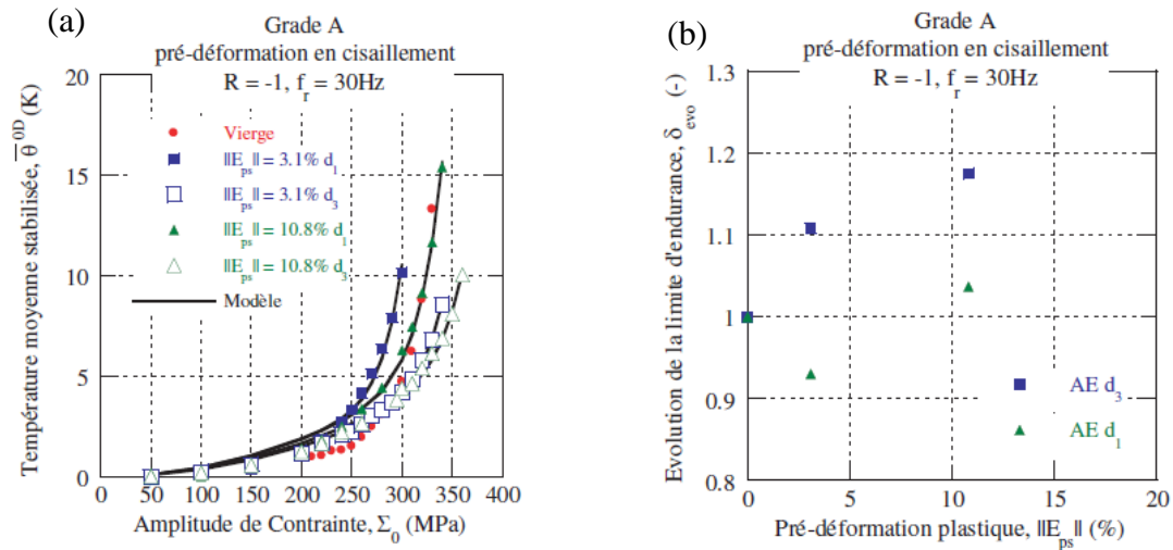
Figure 1.61 : (a) Indentification des paramètres du modèle sur les courbes d'auto-échauffement d'un acier grade A après une pré-déformation plastique en cisaillement ; (b) Prédiction de l'évolution des propriétés en fatigue d'un acier grade A après pré-déformation plastique dans les directions d_1 et d_3 . (Munier, 2012)
