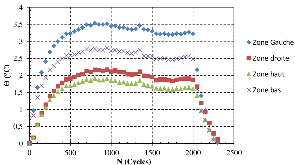
Figure 5.22 : Evolution de la température \Theta au cours d'un palier d'auto-échauffement (amplitude de contrainte théorique 30 MPa) pour les 4 zones mesurées autour du trou.
