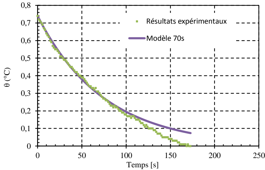
Figure 5.24 : Identification de \tau_{\epsilon q} sur la courbe de refroidissement de la zone à gauche du trou sur éprouvette Kt2.5 à l'endroit du point chaud (zone 5 sur la Figure 5.18).
