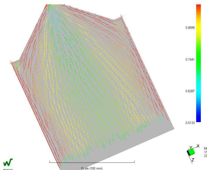
Figure 2.29 : Prévion de la composante a_{11} du tenseur d'orientation des fibres, en peau, après injection des plaques - simulation rhéologique Moldflow®
