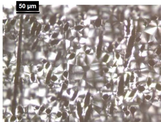
Figure 1.30 : Observation de la structure cristalline dans un polyamide renforcé de fibres de verre par microscopie optique à polarisation croisée. (Mourglia, 2009).
