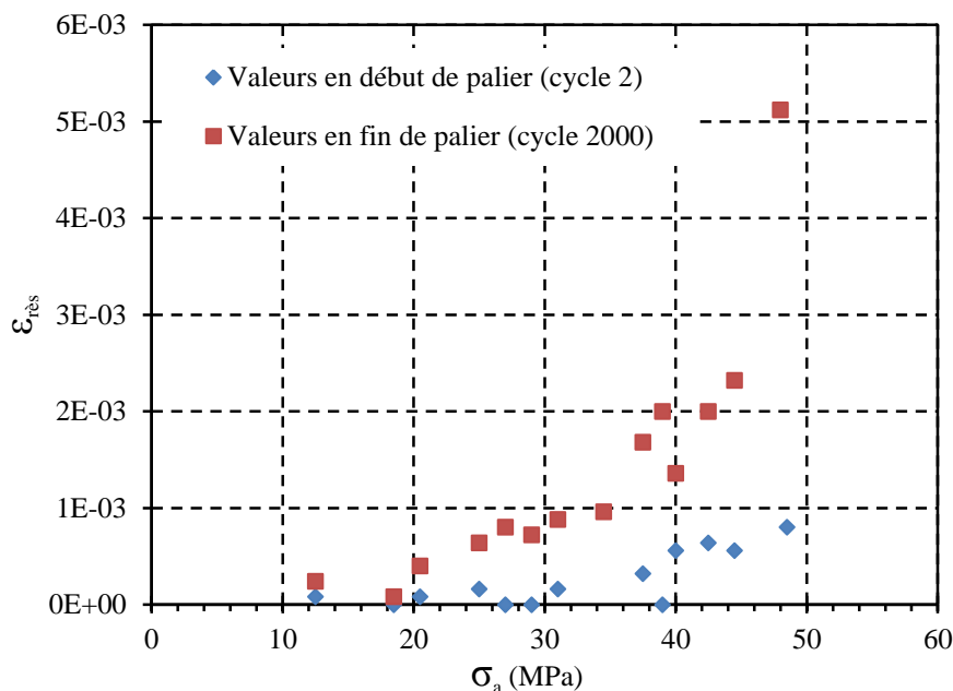
Figure 2.57 : Evolution de la déformation résiduelle en début et en fin de palier d'auto-échauffement pour les Tests 1, 2 et 3.
