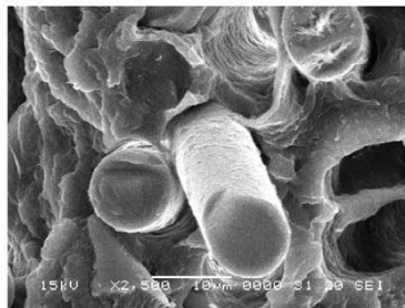
Figure 1.25 : Faciès de rupture d'un PA66 renforcé obtenu par MEB. (Fu, 2005).
