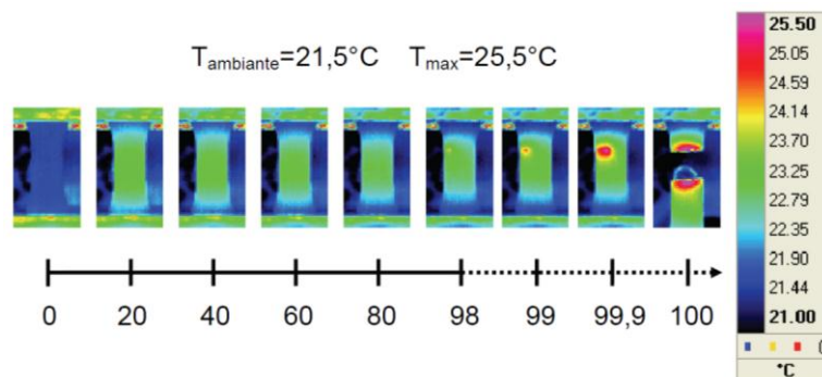
Figure 1.66 : Echauffement mesuré par thermographie infrarouge à la surface d'un polymère renforcé en fonction de sa fraction de durée de vie. (Klimkeit, 2009)
