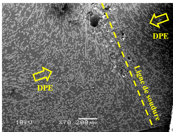
Figure 2.36 : Microstructure d'une ligne de soudure vue au MEB.
