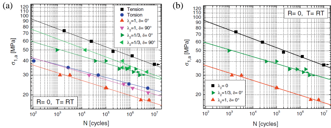
Figure 1.46 : Courbe de Wöhler obtenue en traction-torsion sur éprouvettes « diabolos tubulaires » injectées en PA66GF35 et sollicité à R=0 , à température ambiante (a) influence de l'interaction bi-axialité/déphasage, (b) influence de la bi-axialité. (De Monte, 2009)
