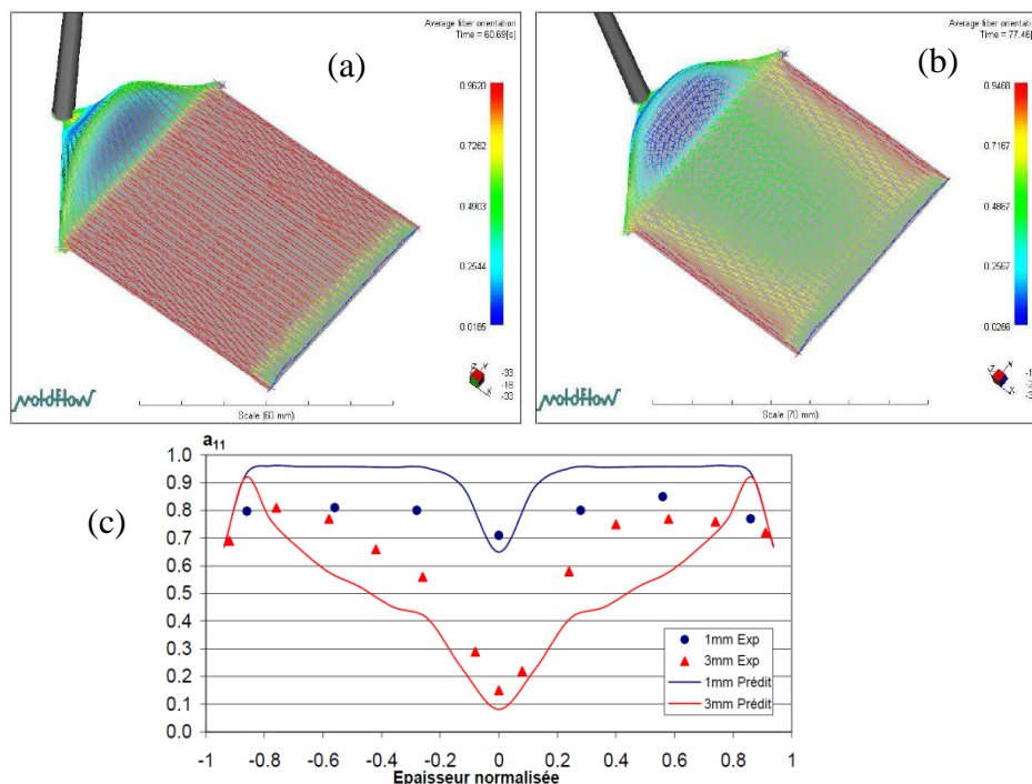
Figure 1.22 : Prévission moyenne des tenseurs d'orientation (composante a_{11} ) obtenue par le logiciel Moldflow dans une plaque de 1mm d'épaisseur (a) ou de 3mm d'épaisseur (b), (c) Prévission dans l'épaisseur de la composante a_{11} pour les 2 plaques et comparaison avec les mesures expérimentales. Matériau Polyarylamide renforcé à 30% en masse. (Dray, 2006)
