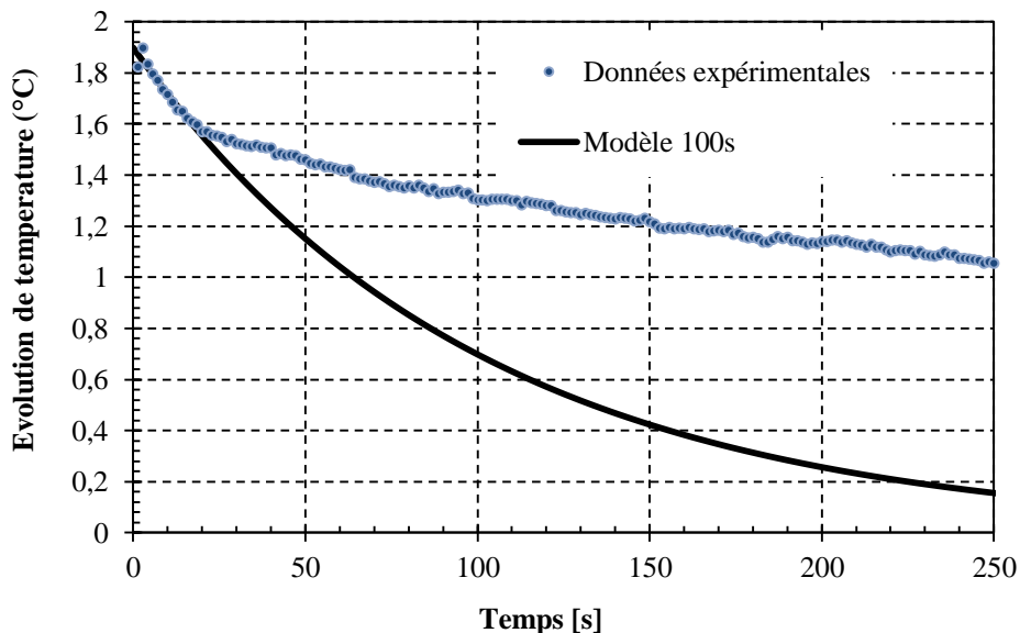
Figure 5.44 : Identification de \tau_{\acute{e}q} sur la courbe de refroidissement du palier F_a=7.5\text{ kN} lors d'un essai d'auto-échauffement sur pièce prototype en PA66GF50 RH35%.
