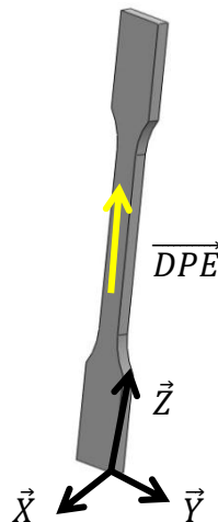
Figure 2.9 : Vue 3D d'une éprouvette ISO avec son repère orthonormé de référence.
