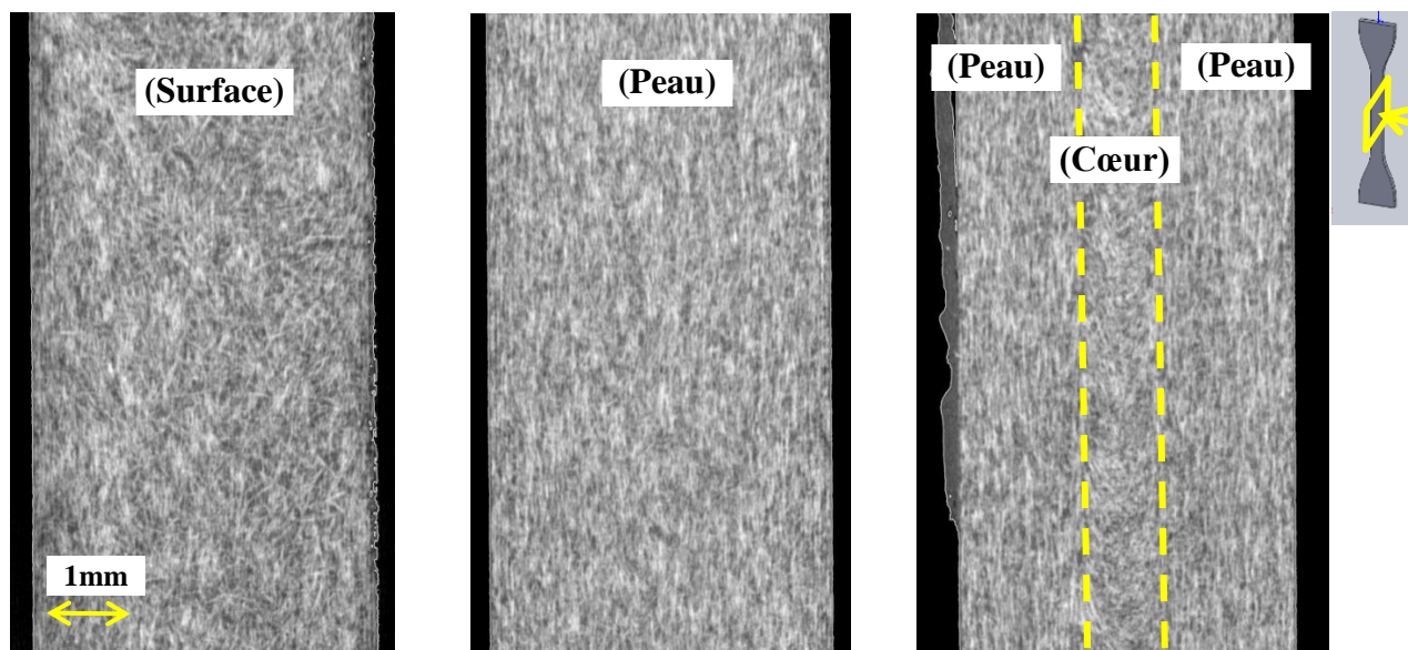
Figure 2.23 : ISO527 vue en coupe ( \vec{X}; \vec{Z} ) obtenue en MTRX ; (a) zone de surface ; (b) zone de peau ; (c) plan médian de l'éprouvette
