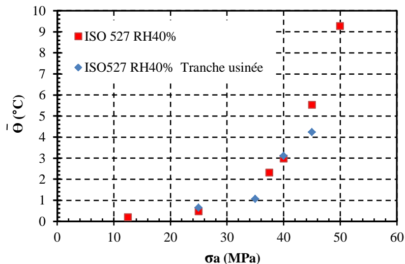
Figure 5.4 : Comparaison des courbes d'auto-échauffement obtenues sur éprouvettes ISO527 RH40% : mesures sur la surface de la zone utile (carrés rouges) et mesures sur la surface de la tranche après usinage (losanges bleus).
