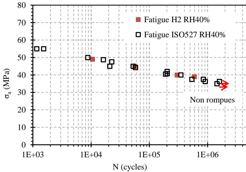
Figure 3.6 : Comparaison des essais de fatigue réalisés sur un PA66GF50 pour des éprouvettes ISO527 RH40% et des éprouvettes H2 RH40%, à R=0, f=1Hz et T_{amb}=23^{\circ}C .
