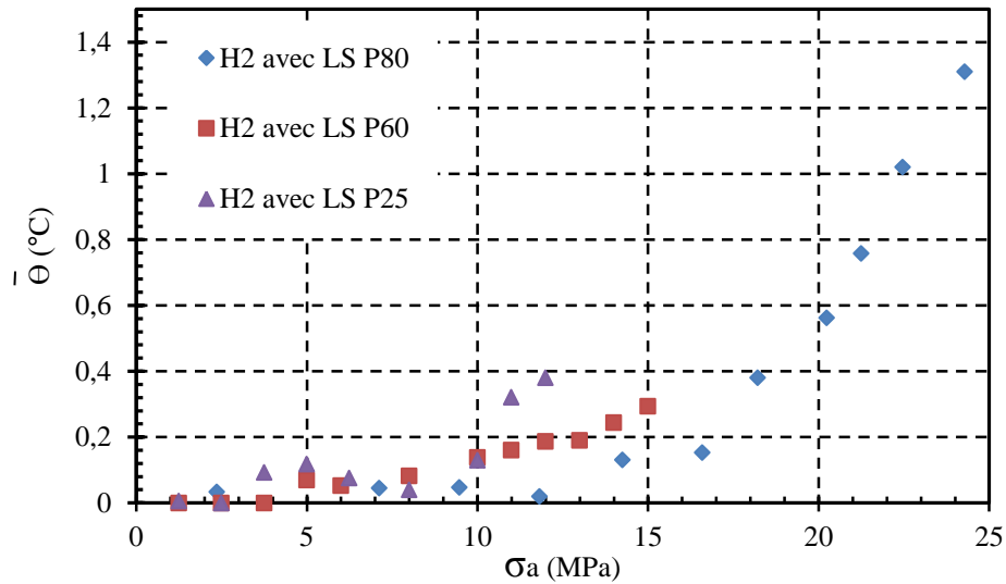
Figure 3.38 : Comparaison des courbes obtenues en caractérisation « rapide », pour un PA66GF50, sous forme d'éprouvettes H2 (RH50%) avec LS, pour une pression de maintien de 80 bar, 60 bar et 25 bar.
