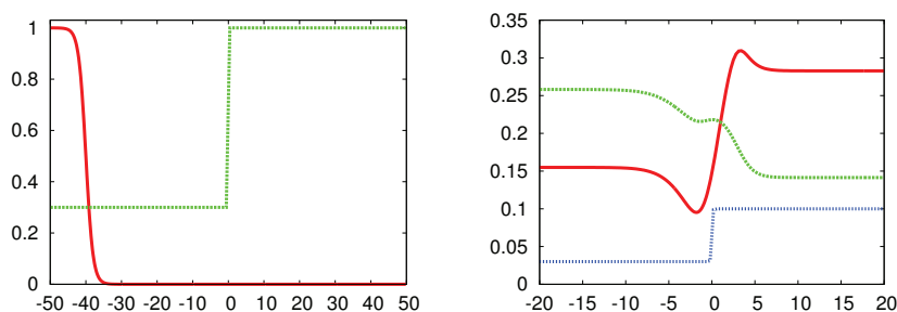
FIGURE III.8 – Interaction d'un front avec un défaut antisymétrique étroit. Le panneau de gauche montre le front incident u(x, 0) avec le défaut s(x) . Le panneau de droite montre la vitesse \dot{x}_0 et la largeur (mise à l'échelle) w/10 du front en fonction de sa position centrale x_0 . Les paramètres sont s_l = 0, 3 , s_r = 1 (saut de 0, 7) et d = 0, 1 .
