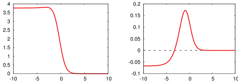
FIGURE IV.8 – Tracés des termes sources pour un « Heaviside » : \int_{-\infty}^{\infty} (11 - 12U(z)) R_m(U(z)) dz (à gauche) et \int_{-\infty}^{\infty} (1 - 2U(z)) R_m(U(z)) dz (à droite) en fonction de la variable z .
