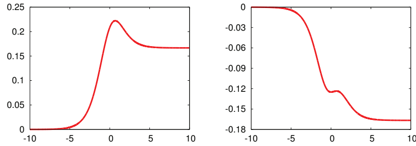
FIGURE III.15 – Tracés des termes sources T_1 et T_2 pour une zone sans réaction : T_1(y) = \int_{-\infty}^y R_b(U(z)) dz et T_2(y) = \int_{-\infty}^y (1-2U(z))R_b(U(z)) dz en fonction de la variable y . Ici on a choisi a = \frac{1}{3} .
