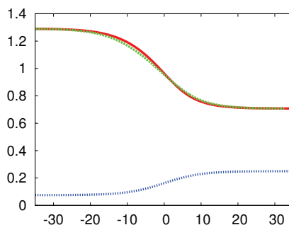
FIGURE III.10 – Tracé (x_0, w) pour l'équation aux dérivées partielles (III.1) en trait continu (rouge) et pour les équations d'évolution des coordonnées collectives (III.2) en trait discontinu (vert), dans le cas d'un défaut antisymétrique présenté en pointillé (bleu).
