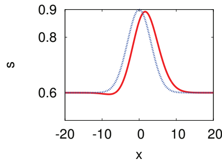
FIGURE III.17 – Estimation de la topographie du défaut s(x) obtenue à partir de la solution de l'équation aux dérivées partielles. Cette estimation venue de (III.17) est présentée en trait pointillé (bleu), tandis que le s(x) réel est en trait plein (rouge).
