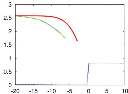
FIGURE III.13 – Tracé (x_0, w) pour l'équation aux dérivées partielles (III.1) en trait continu (rouge) et pour les équations d'évolution des coordonnées collectives (III.8) en trait discontinu (vert), dans le cas d'un défaut antisymétrique étroit présenté en pointillé (bleu). Il montre le défaut (mis à l'échelle) s(x)/10 .
