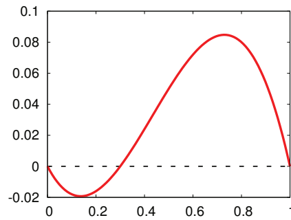
FIGURE III.1 – Terme de réaction bistable. Ici on a choisi a = 0,3 .
