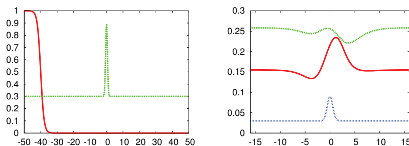
FIGURE III.5 – Mouvement d'un front alors qu'il rencontre un défaut étroit. Le panneau de gauche montre le front incident avec le défaut s(x) . Le panneau de droite montre en rouge la vitesse \dot{x}_0 et en vert la largeur mise à l'échelle w/10 du front en fonction de la position centrale x_0 . Le défaut mis à l'échelle s(x)/10 est rappelé en bleu. Les paramètres sont s_0 = 0,3 , s_1 = 0,6 et d = 0,3 .
