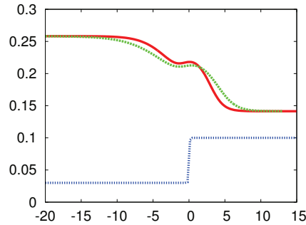
FIGURE III.12 – Tracé (x_0, w) pour l'équation aux dérivées partielles (III.1) en trait continu (rouge) et pour les équations d'évolution des coordonnées collectives (III.8) en trait discontinu (vert), dans le cas d'un défaut antisymétrique étroit présenté en pointillé (bleu). Les paramètres sont s_l = 0, 3 , s_r = 1 (saut de 0, 7) et d = 0, 1 .
