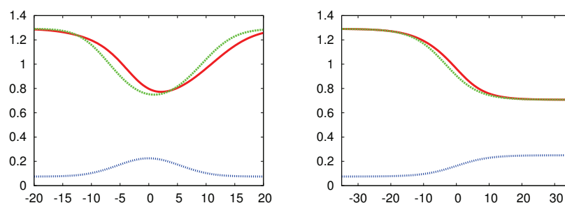
FIGURE III.9 – Tracés (x_0, w) pour l'équation aux dérivées partielles (III.1) en trait continu (rouge) et pour les équations d'évolution des coordonnées collectives (III.4) en trait discontinu (vert). Le panneau de gauche (respectivement de droite) correspond à un défaut symétrique (respectivement antisymétrique). Les défauts sont rappelés au bas de chaque panneau.
