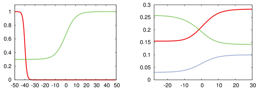
FIGURE III.7 – Interaction d'un front avec un défaut antisymétrique large. Le panneau de gauche montre le front incident u(x,0) avec le défaut s(x) . Le panneau de droite montre la vitesse \dot{x}_0 et la largeur (mise à l'échelle) w/10 du front en fonction de sa position centrale x_0 . Les paramètres sont s_l = 0,3 , s_r = 1 (saut de 0,7) et d = 10 .
