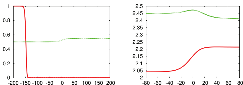
FIGURE IV.3 – Mouvement adiabatique d'un front. Le panneau de gauche montre le front incident u(x, 0) en trait continu (rouge) avec le défaut (mis à l'échelle) s(x)/2 en trait pointillé (vert). Le panneau de droite montre la vitesse \dot{x}_0 et la largeur w du front en fonction de la position centrale x_0 . Les paramètres sont s_l = 1 , s_r = 1, 1 et d = 20 .
