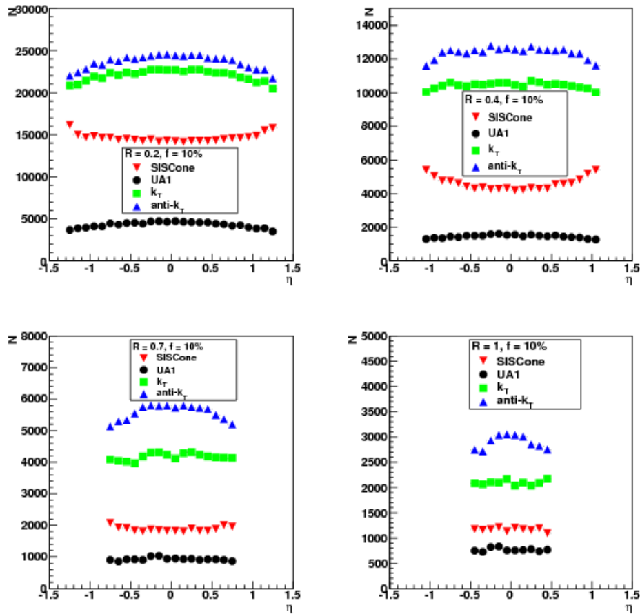
FIGURE 8.22 – Distribution selon \eta des jets (haut intervalle de p_{T,\text{hard}} ) reconstruits par UA1 (points noirs), k_T (carrés verts), \text{anti-k}_T (triangles bleus) et par SISConc (triangles inversés rouges), pour un paramètre de recouvrement de 10% et un rayon de 0.2 (en haut à gauche), 0.4 (en haut à droite), 0.7 (en bas à gauche) et 1 (en bas à droite).
