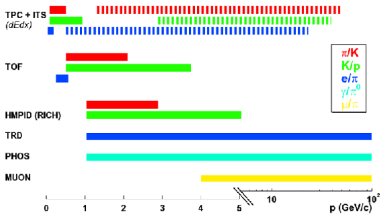
FIGURE 4.21 – Capacité d’identification des particules par ALICE, pour une séparation à 3\sigma (en ligne continue) et à 2\sigma (en ligne hachurée), en fonction de l’impulsion de sparticules.
