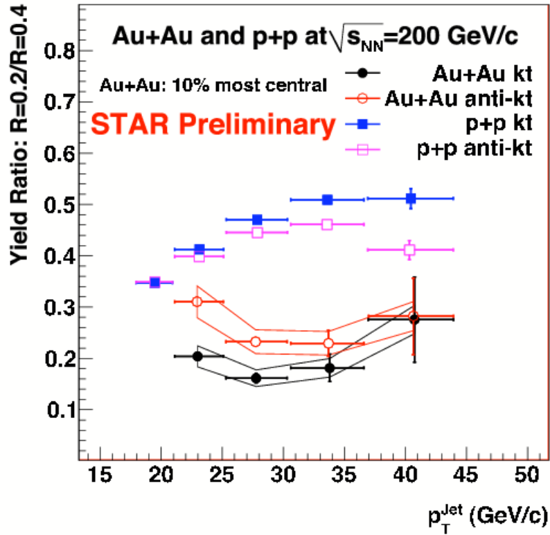
FIGURE 3.15 – Rapports de taux de production de jets reconstruits avec un rayon de 0.2 aux jets reconstruits avec un rayon de 0.4 dans les collisions p+p (carrés) et Au+Au (cercles) à 200 GeV. Les jets ont été reconstruits avec deux algorithmes : k_T (symboles pleins) et anti- k_T (symboles vides) [62].
