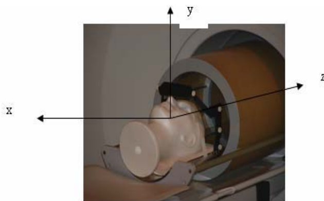
Figure 9 : Représentation du repère spatial « x » : gauche/droite, « y » : arrière/avant et « z » : bas/haut.
