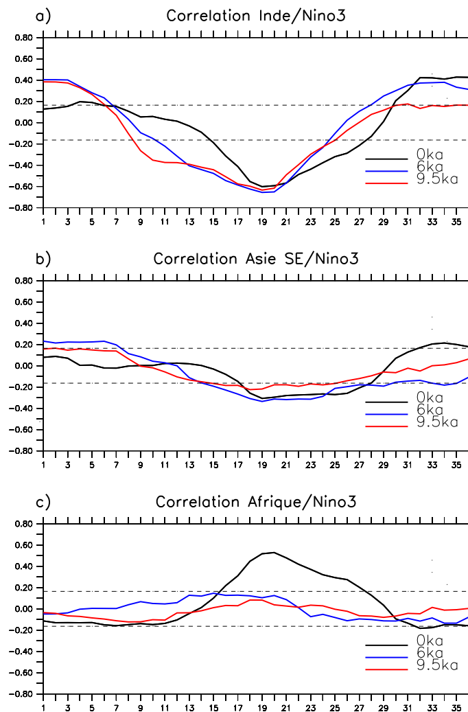
FIGURE 3.5: Corrélation glissante entre les précipitations de mousson JJAS de l'année 0 (mois 18 à 21) et les SSTs de la région Niño3 de l'année précédente (mois 1 à 12) à l'année suivante (mois 25 à 36) pour (a) l'Inde, (b) l'Asie du sud-est, (c) l'Afrique. Les traits en pointillé représentent les niveaux de significativité à 90% des corrélations.
