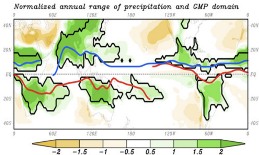
FIGURE 2.1: Variation saisonnière des précipitations (été moins hiver, normalisé par la moyenne annuelle, couleur). Domaine de précipitation de mousson globale : variation saisonnière \geq 2\text{mm}/\text{jour} et 70% de la moyenne annuelle (contours noirs). Position de la ZCIT en été (juillet-août, ligne bleue) et en hiver (janvier-février, ligne rouge). Figure issue de Wang and Ding (2008)
