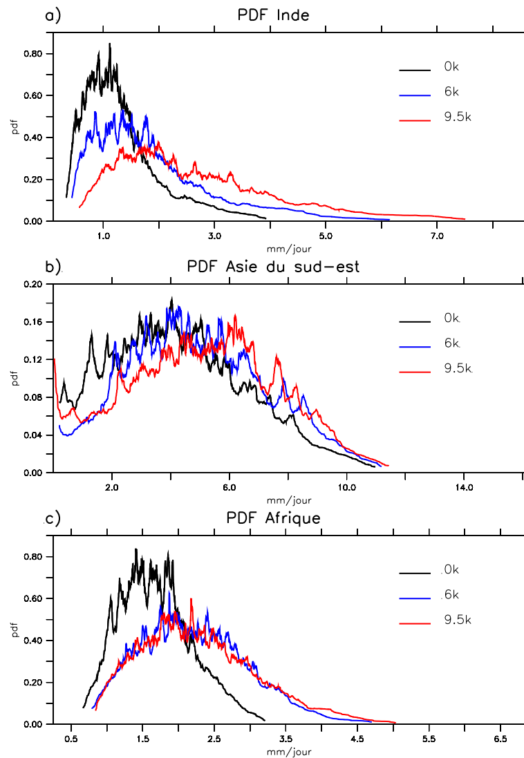
FIGURE 3.2: Densité de probabilité de 31 ans de précipitations journalières de juin à septembre pour 0, 6 et 9.5 ka moyennées sur (a) l'Inde ( 70-100^{\circ}\text{E} , 10-35^{\circ}\text{N} ), (b) l'Asie du sud-est ( 105-135^{\circ}\text{E} , 20-45^{\circ}\text{N} ) et (c) le Sahel ( 20^{\circ}\text{O}-20^{\circ}\text{E} , 7-18^{\circ}\text{N} )
