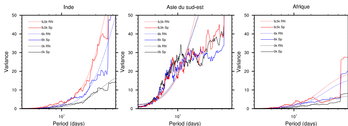
FIGURE 3.1: Transformée de Fourier de 31 ans de précipitations journalières de juin à septembre pour 0, 6 et 9.5 ka moyennées sur (a) l'Inde (70-100°E, 10-35°N), (b) l'Asie du sud-est (105-135°E, 20-45°N) et (c) le Sahel (20°O-20°E, 7-18°N). Les courbes en pointillé représentent le spectre du bruit rouge correspondant à chaque série temporelle.
