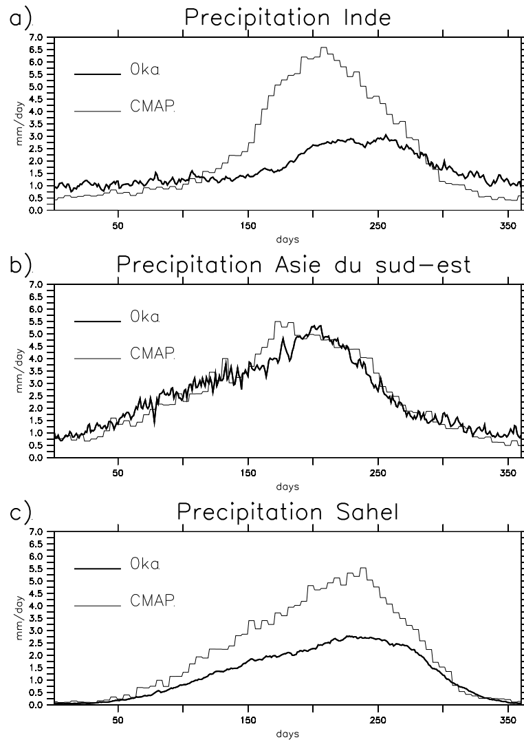
FIGURE 2.4: Cycle saisonnier des précipitations continentales sur (a) l'Inde ( 70-100^{\circ}\text{E} , 10-35^{\circ}\text{N} ), (b) l'Asie du sud-est ( 105-135^{\circ}\text{E} , 20-45^{\circ}\text{N} ) et (c) le Sahel ( 20^{\circ}\text{O}-30^{\circ}\text{E} , 5-17^{\circ}\text{N} ) pour les données CMAP (pentad, trait fin) et pour 0 ka (journalières, trait gras).
