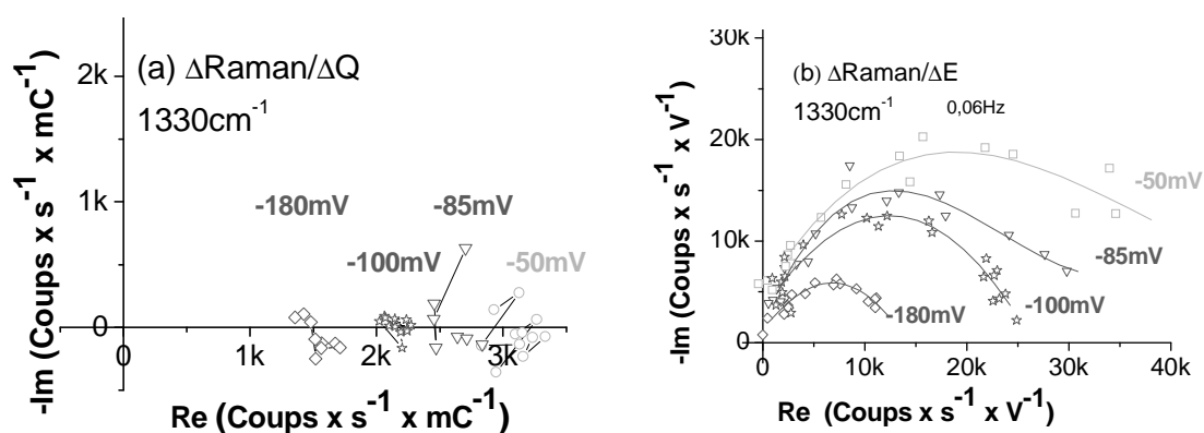
Figure 41 : Réponses des fonctions de transfert (a) \Delta Raman/\Delta Q et (b) \Delta Raman/\Delta E pour la bande Raman à 1330\text{ cm}^{-1} ; à pH 2.5 et pour quatre potentiels
