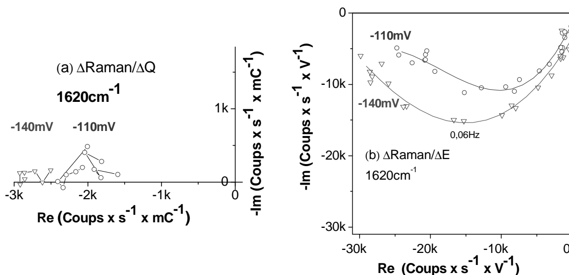
Figure 57 : Réponses des fonctions de transfert (a) \Delta Raman/\Delta Q et (b) \Delta Raman/\Delta E pour la bande Raman à 1620\text{cm}^{-1} , à pH 3.7 et pour deux potentiels
