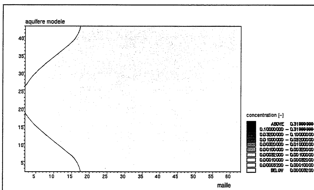
Fig. III.3.6 : Dispersion d'un nuage en 3 dimensions, source intermittente, \alpha_T(300m) = 25m
