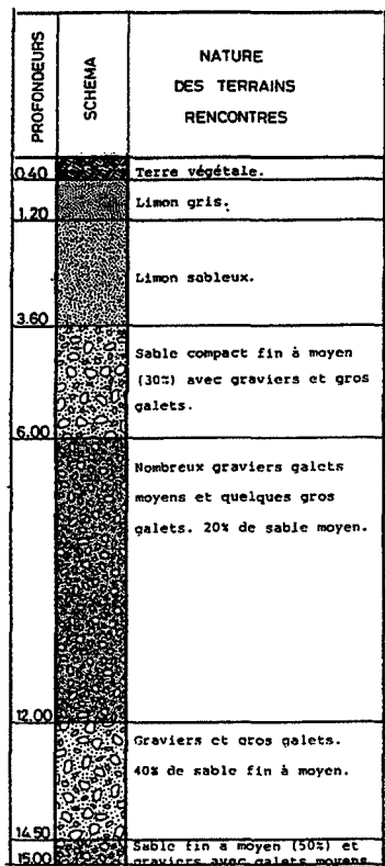
Fig. I.2.8 : Coupe géologique de la zone d'étude
