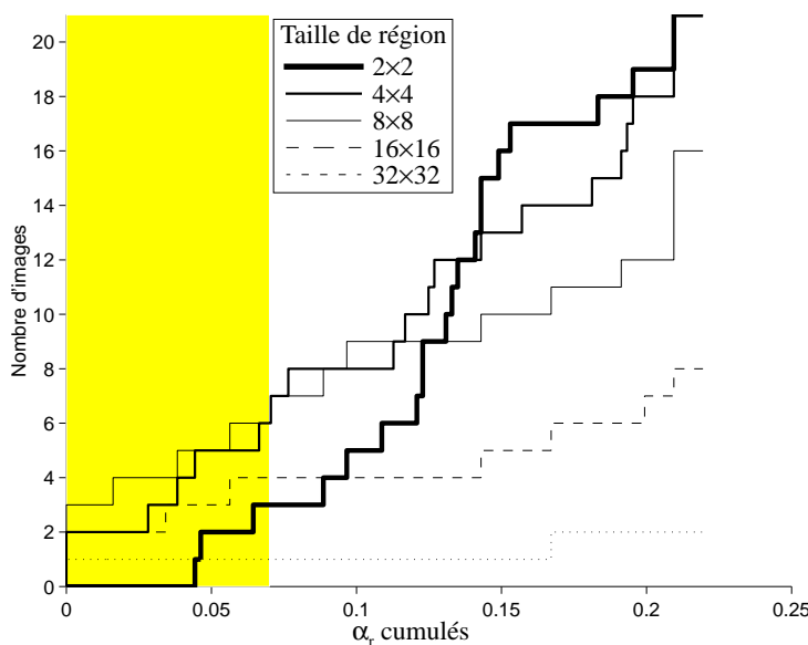
Figure 79: Fréquence cumulée de \alpha_r pour la moyenne approchée sur l’ensemble du panel en fonction de la taille des régions. \alpha = 0,07 (en grisé), \beta = 0,07 , p_h = 0,8
