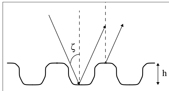
Figure 5: Interférences sur surface rugueuse
