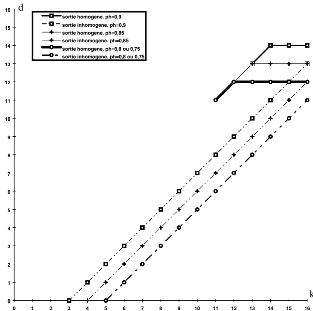
Figure 74: Région critique pour une région de taille 4x4. \alpha = 0,1, 0,01 \leq \beta \leq 0,1, 0,9 \geq p_h \geq 0,75
