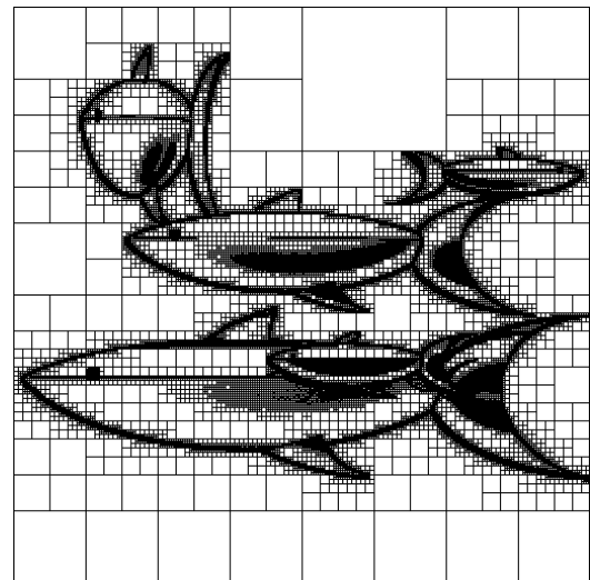
Figure 115: Points échantillonnés avec cohérence
