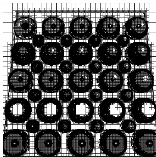
Figure 133: Points échantillonnés avec cohérence
