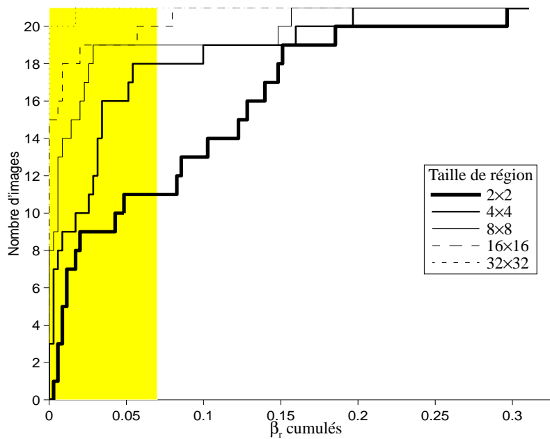
Figure 77: Fréquence cumulée de \beta_r sur l'ensemble du panel en fonction de la taille des régions. \alpha = 0,07 , \beta = 0,07 (en grisé), p_h = 0,9
