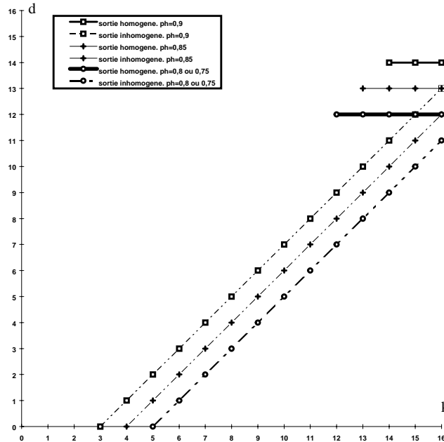
Figure 73: Région critique pour une région de taille 4x4. 0,01 \leq \alpha \leq 0,06, 0,01 \leq \beta \leq 0,1, 0,9 \geq p_h \geq 0,75
