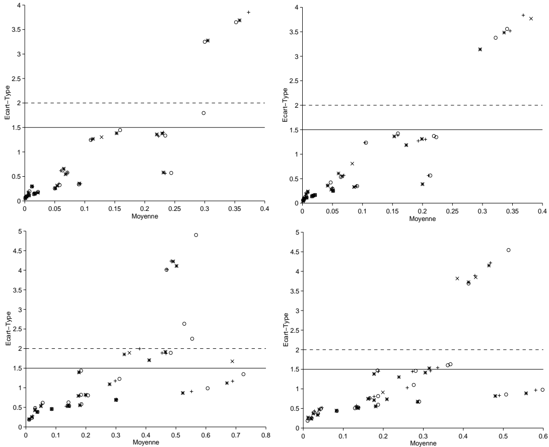
Figure 88: Distances colorimétriques pour les images du panel calculées par le test express. \epsilon = 1 (en haut), \epsilon = 2 (en bas), p_h = 0,8 (à gauche), p_h = 0,95 (à droite), \mu_{hh} : \circ : 0,2 + : 0,15 * : 0,1 \times : 0,05
