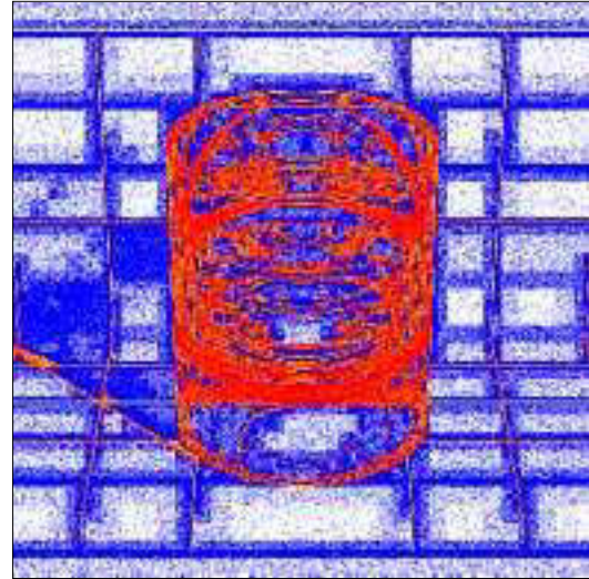
Figure 124: Points échantillonnés avec cohérence
