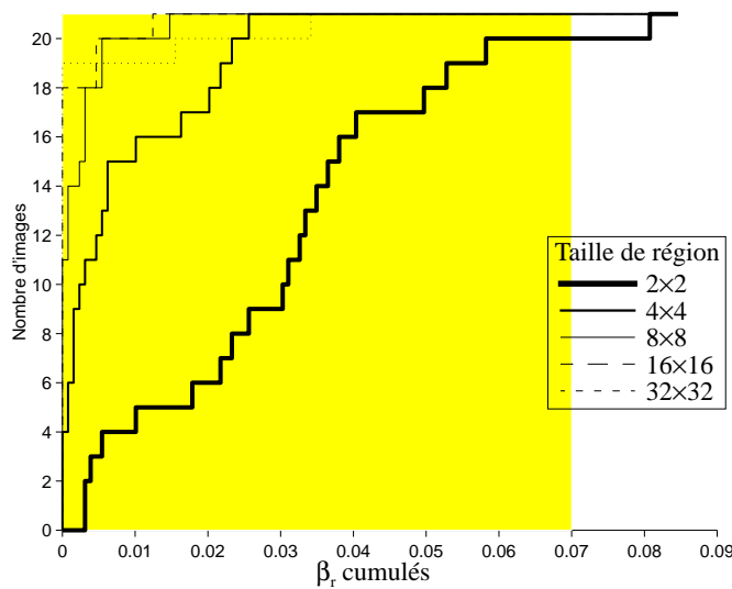
Figure 78: Fréquence cumulée de \beta_r pour la moyenne approchée sur l’ensemble du panel en fonction de la taille des régions. \alpha = 0,07 , \beta = 0,07 (en grisé), p_h = 0,8
