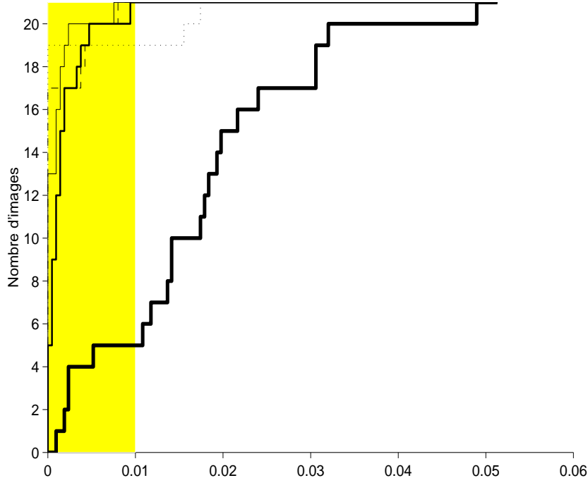
Figure 86: Fréquence cumulée de \beta'_r pour le test express sur l'ensemble du panel en fonction de la taille des régions. \varepsilon = 2 , \alpha' = 0,02 , \beta' = 0,01 (en gris), p_h = 0,95 , \mu_{hh} = 0,05
