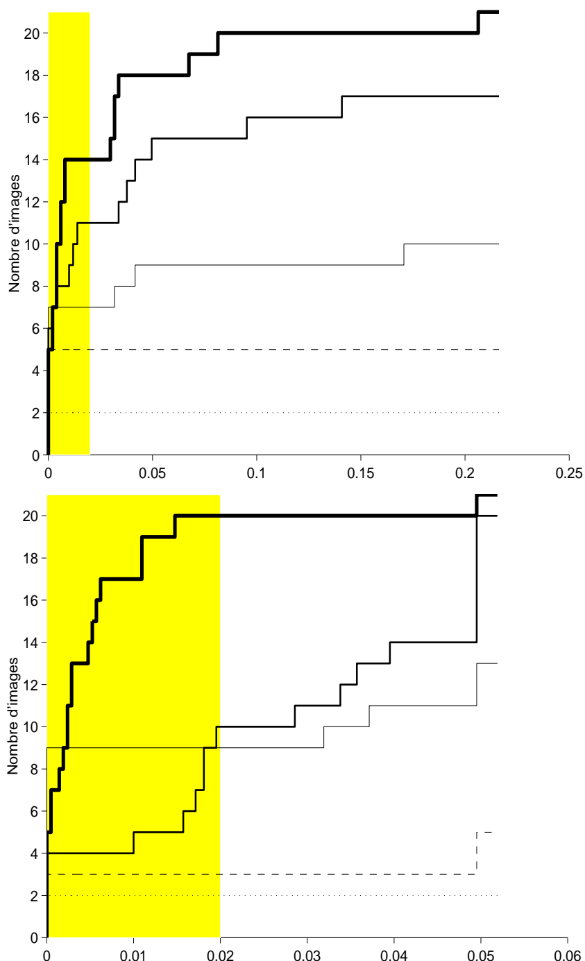
Figure 87: Fréquence cumulée de \alpha'_r pour le test express sur l'ensemble du panel en fonction de la taille des régions. \alpha' = 0,02 (en gris), \beta' = 0,01 , p_h = 0,95 , \mu_{hh} = 0,05 . \varepsilon = 1 (en haut) \varepsilon = 2 (en bas). Noter la différence d'échelle
