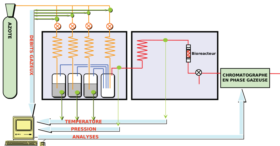
FIG. 4.1 – Schéma du réacteur continu solide/gaz.
