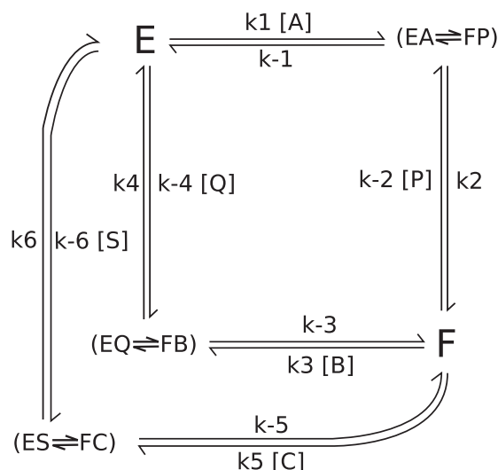
FIG. 8.2 – Représentation de King-Altman avec l'enzyme (E), l'acyl-enzyme (F), l'ester (A), les alcools R et S (respectivement B and C), l'alcool produit partant (P), les esters produits R et S (respectivement Q and S).
