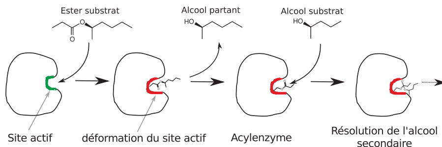
FIG. 3.1 – Schéma de l'effet d'empreinte par la partie alkyle du donneur d'acyle.
