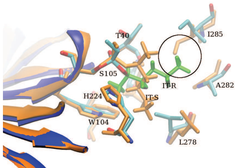
FIG. 8.17 – Représentation du feuillet \beta et du site actif avec enz-IT- R (feuillet en bleu, atomes de carbone en bleu ciel, atomes d'azote en bleu foncé, et atomes d'oxygène en rouge, groupe alcoxyle du substrat en vert) et enz-IT- S (toute la structure en orange).
