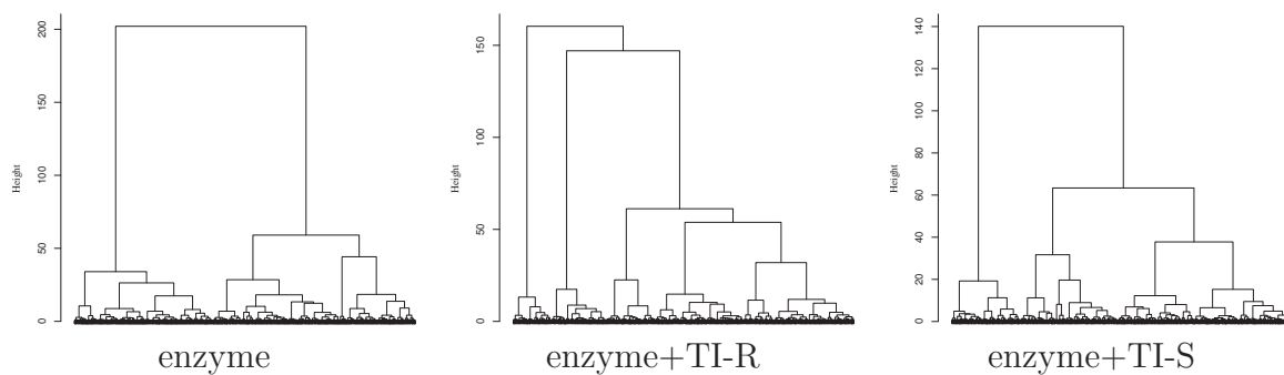
FIG. B.1 – Dendrogrammes définis avec la méthode Ward à partir de la matrice RMSD calculée sur la trajectoire de 20 ns pour l'enzyme seul et l'enzyme avec l'intermédiaire tétraédrique formé avec les énantiomères R et S du propanoate de 1-méthylpentyle.
