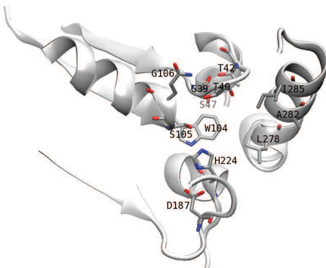
FIG. 1.6 – Site actif de la CALB (vue 2).
