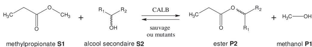
FIG. 1.10 – La réaction de transestérification des alcools secondaires.
