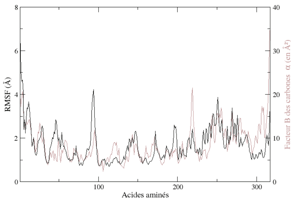
FIG. 6.9 – RMSF du squelette peptidique (en Å) des 317 acides aminés de la CALB dans la trajectoire avec le modèle de solvation EEF1 (en noir). Facteurs B de la structure cristallographique (code PDB : 1TCA) de la CALB (en brun rosé).
