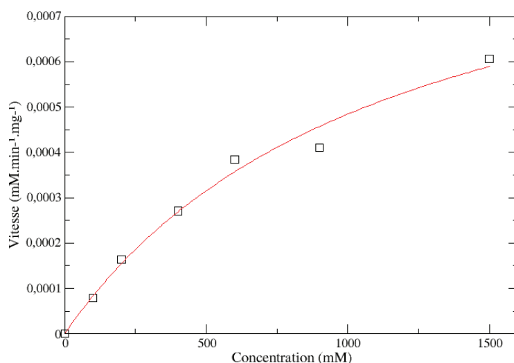
FIG. 7.3 – Courbe de saturation de la CALB avec le ( S )-pentan-2-ol. Réaction de transestérification à 45 °C dans le 2-méthylbutan-2-ol, en présence de 5 g.L -1 de la CALB immobilisée.
