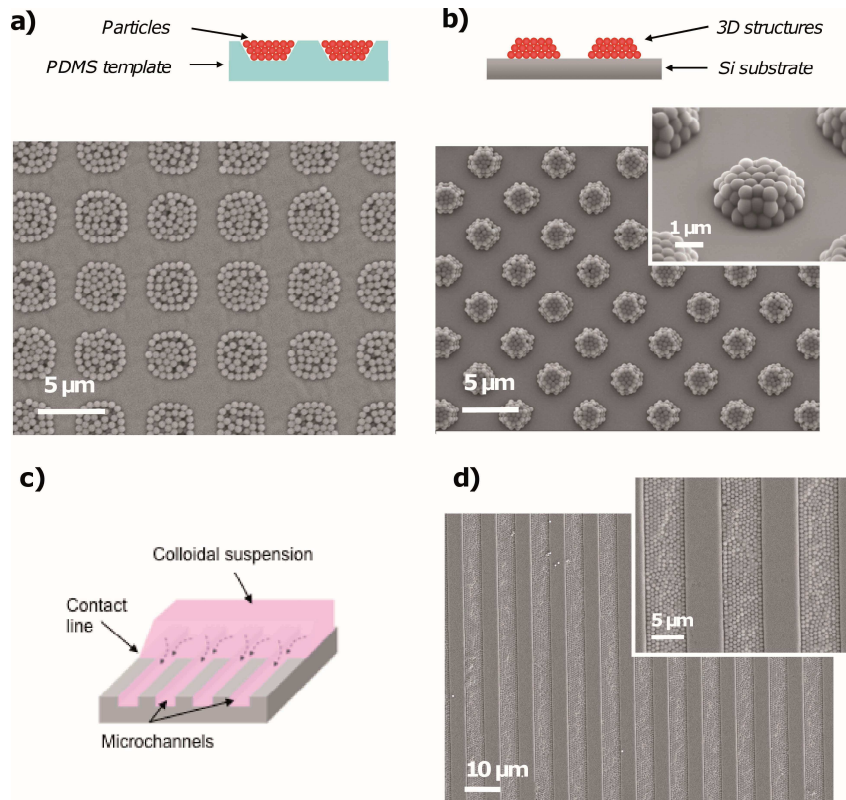
Figure 17: a) Nanoparticules de polystyrène de 500 nm assemblées dans des cavités évasées de 2.5 \mu\text{m} de profondeur sur du PDMS. b) Les structures obtenues après transfert sur du silicium. c,d) Les mêmes particules ont aussi été assemblées dans des « tranchées » de 500 nm de profondeur et de 5 \mu\text{m} de largeur sur du PDMS. Dans ces expériences, la vitesse du substrat est comprise entre 1 et 10 \mu\text{m}\cdot\text{s}^{-1} . 59
