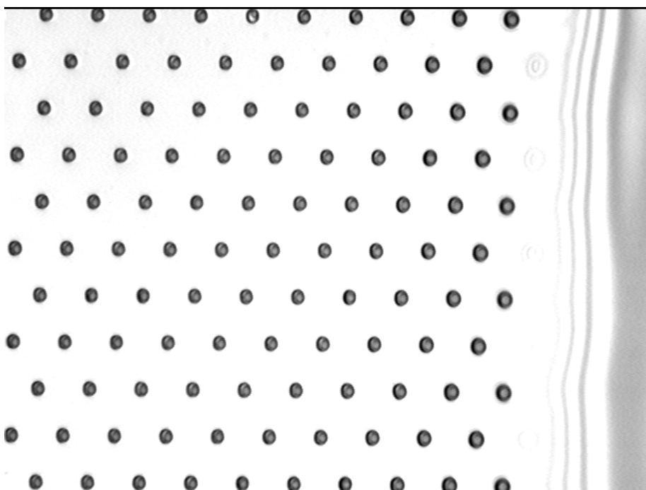
Figure 23: Billes de 4,5 \mu\text{m} dans des plots de polymères. A droite, les billes semblent de diamètres plus gros, il s'agit sans doute d'une illusion d'optique. Diamètre des billes : 4,5 \mu\text{m} . Profondeur des cavités : 2,5-3 \mu\text{m} . Pas du réseau hexagonal : 30 \mu\text{m} .
