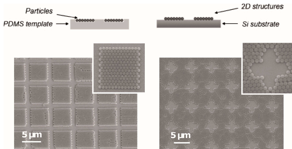
Figure 12 : Assemblage convectif sur substrat structuré. Des particules de polystyrène ont été assemblées sur un substrat en PDMS ( T_s=20^\circ\text{C} , v_s=1.5 \mu\text{m}\cdot\text{s}^{-1} avec des motifs de 200 nm de profondeur). Les structures réalisées ont été transférées sur silicium par contact. 26,48
