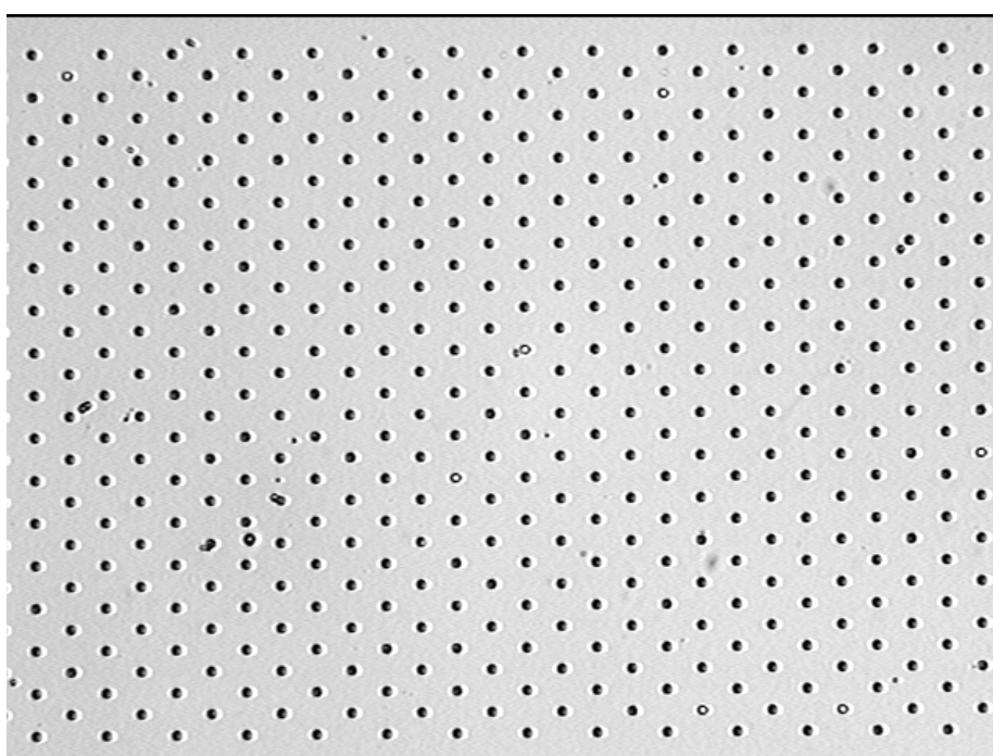
Figure 25: Réseau de billes. En haut sur le PDMS, et en bas sur le silicium après transfert grâce à la NOA61. Diamètre des billes : 4,5 \mu\text{m} . Profondeur des cavités : 2,5-3 \mu\text{m} . Pas du réseau hexagonal : 30 \mu\text{m} .
