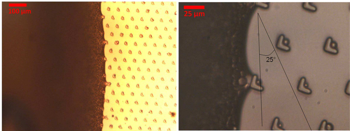
Figure 7 : A gauche: un assemblage capillaire de levures \gamma AT-340 en cours. A droite: un agrandissement. On remarque l'angle formé par l'ouverture des pièges et la ligne de contact. La capture de levures uniques est réalisable. Expériences réalisées à 10 \mu\text{m.s}^{-1} et à température ambiante, directement dans le milieu de culture sans ajout de surfactants.
