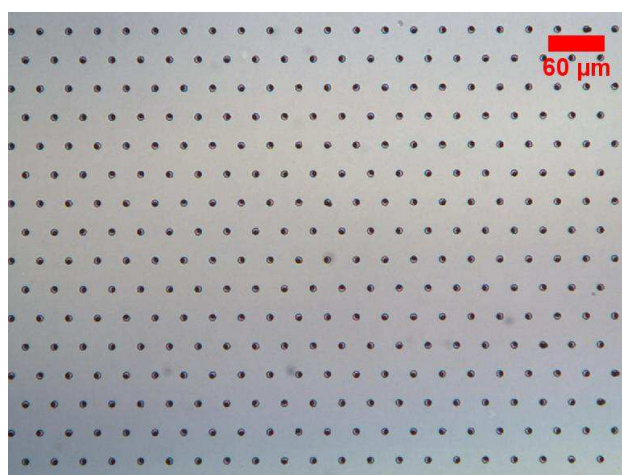
Figure 5 : Un réseau de cavités sur du PDMS. Chaque cavité contient une bille magnétique de 4,5\ \mu\text{m} (Dynabeads®, Invitrogen). On crée un réseau de colonnes à partir d'un tel substrat.
