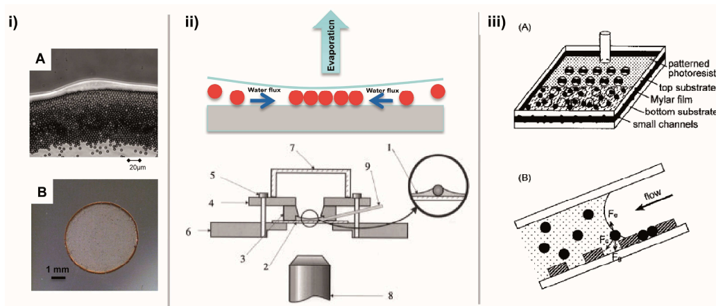
Figure 6 : i) Illustration de l'effet « goutte de café ». A) Le bord d'une goutte de suspension de particules (de 100 nm et de 5 \mu\text{m} ). Durant le séchage, les particules se concentrent au bord de la goutte. 52,67 B) Quand le séchage est terminé, cette concentration sur le bord fait apparaître un anneau. Ici une goutte de café classique. ii) Illustration du processus et du set-up expérimental utilisé par N.D. Denkov et son groupe pour l'assemblage de particules confinées dans un film mince de liquide. 50,68 iii) Schéma de la procédure employée par Y. Xia et son groupe pour construire de petits agrégats avec des particules colloïdales. L'équilibre entre la force gravitationnelle, électrostatique (fonction des charges de surface) et capillaire conduit au piégeage des particules uniquement dans les motifs. 26
