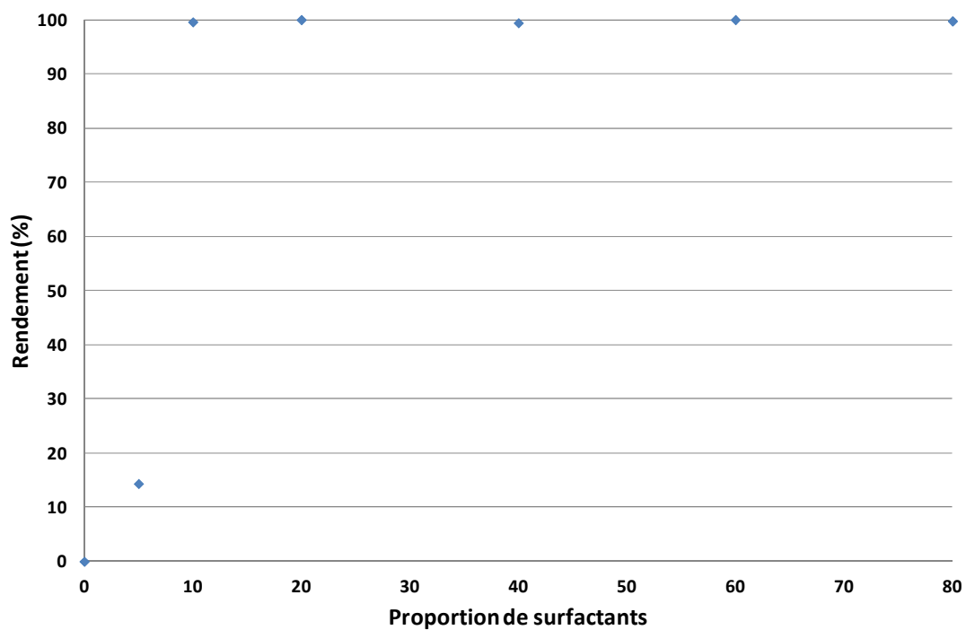
Figure 14 : Rendement de l'assemblage sur un réseau de cavités de 6\ \mu\text{m} de diamètre et de 2,5\ \mu\text{m} de profondeur, pour des particules magnétiques de 4,5\ \mu\text{m} sur du PDMS. T=20^\circ\text{C} . v_s=5\ \mu\text{m}\cdot\text{s}^{-1} . Le rendement très faible au départ bondit rapidement avec la concentration en surfactants avant de se stabiliser.
