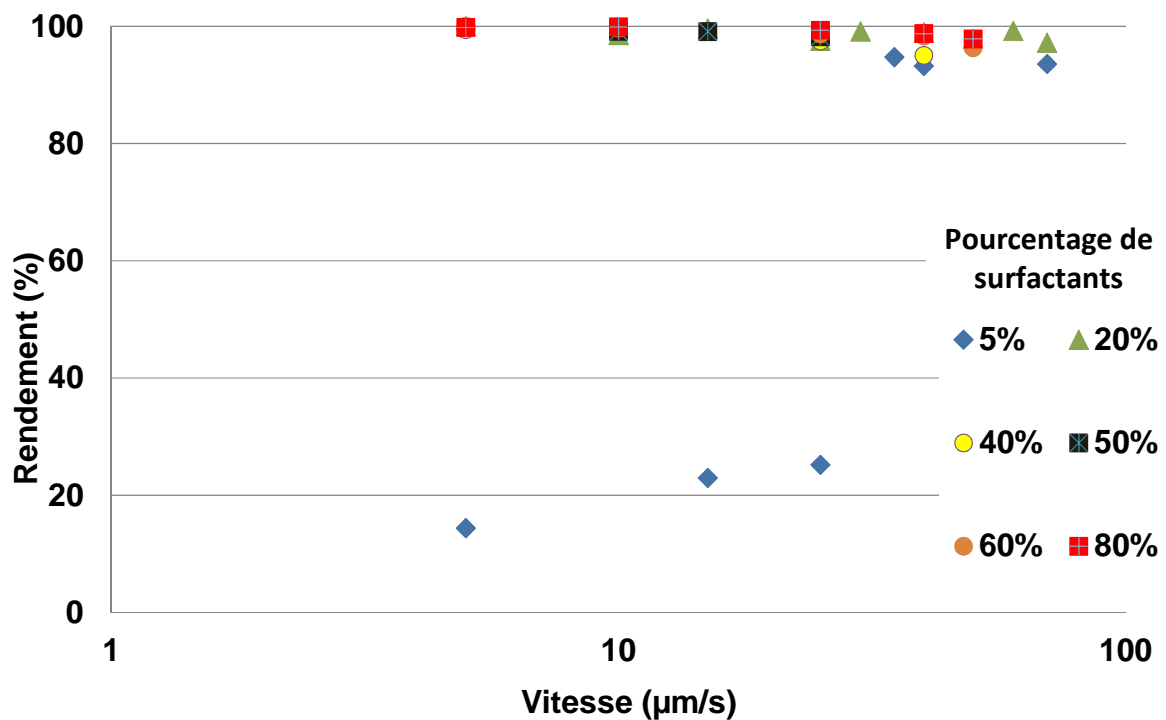
Figure 17 : Courbe représentant le rendement de cavités remplies par une unique particule en fonction de la vitesse et de la concentration en surfactants. Diamètre des cavités : 6 µm. profondeur : 2,5-3 µm. T=20°.
