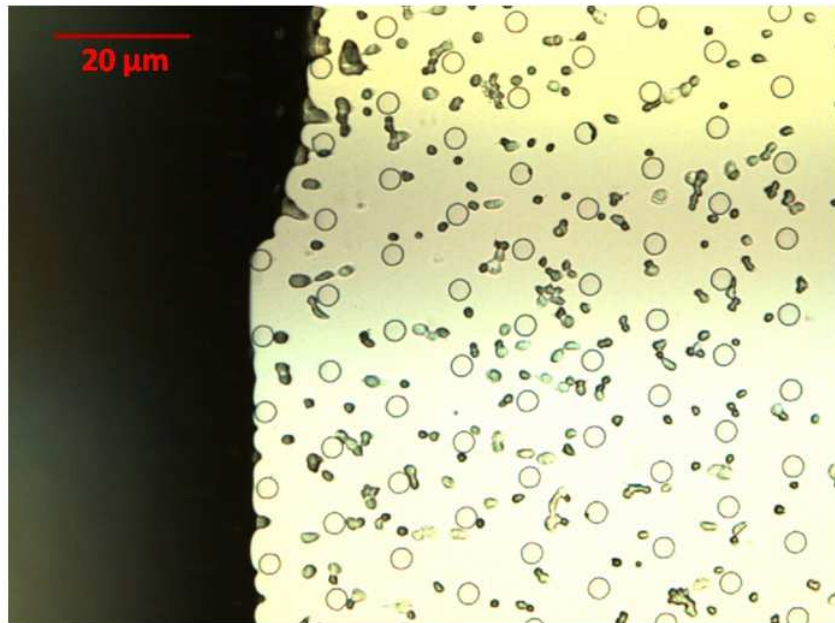
Figure 16 : Tentative d'assemblage capillaire sur du PDMS (dans du PBS) avec des neurones de souris fixées. v_c = 5 \mu\text{m}\cdot\text{s}^{-1} .
