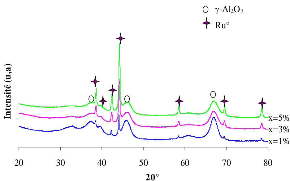
Figure III.11 : Diffractogrammes des rayons X pour les catalyseurs \text{Ru}(x\%)/\text{Al}_2\text{O}_3 après test de vaporeformage du méthane
