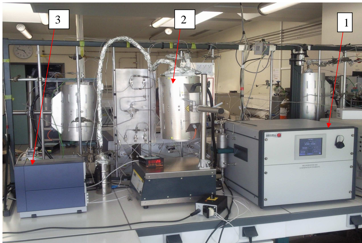
Figure III.2 : Montage expérimental pour la réaction de vaporeformage du méthane
