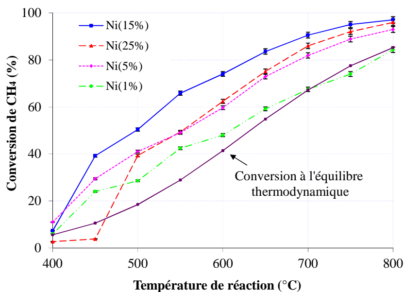
Figure III.8 : Conversion du méthane en fonction de la température de réaction pour Ni(x%)/CeO 2 avec x = 1, 5, 15 et 25 % en masse
