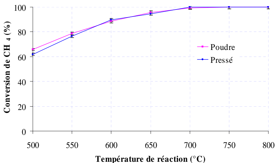
Figure III.33 : Conversion de CH 4 sur Ni(15%)/CeO 2 en fonction de la température à différentes formes
