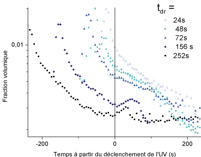
Figure C.2: Evolution de la fraction volumique de liquide pour des mousses ayant plus ou moins drainé avant le déclenchement de l'UV, en fonction du temps d'irradiation UV. Le poreux utilisé pour générer la mousse est de porosité 1, et L_{PB} est évaluée à 1,2mm environ.
