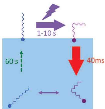
Figure 4.15: Schéma des flux moléculaires à l'interface stimulée La conversion d'une partie des trans en cis à l'interface déclenche la désorption rapide des cis, toutefois la ré-adsorption des cis et trans est peu importante car beaucoup plus lente. La stimulation déclenche un dépeuplement de l'interface. Les flèches de flux sont d'autant plus épaisses que le temps caractéristique est court.
