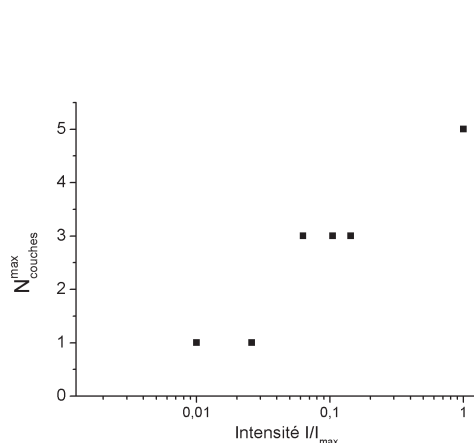
Figure 5.10: (gauche) Effet de l'intensité sur le nombre maximal de couches observées en 3min de stimulation UV ( c=3,5\text{mM} d'AzoTAB ; [\text{NaCl}]=10\text{mM} ; I_{max} = 2\dot{a}4\text{mW}/\text{cm}^2 )
