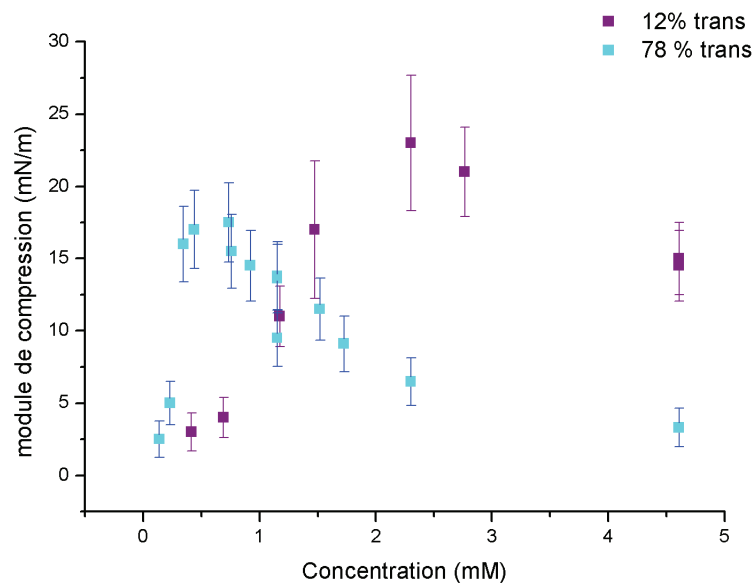
Figure C.1: Module élastique de compression à 2Hz en fonction de la concentration en AzoTAB pour deux fractions en trans différentes.
