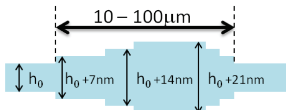
Figure 5.8: Profil schématisé d'une galette. Le rayon varie typiquement entre 10\mu\text{m} et 100\mu\text{m} et l'épaisseur d'une couche est de l'ordre de 5 à 10 nm. Plusieurs couches peuvent se superposer.
