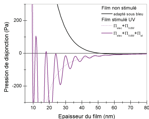
Figure 5.25: (droite) Isothermes de pression de disjonction sous stimulus UV. L'isotherme en pointillés ne comprend que les termes électrostatiques et de Van der Waals, l'isotherme en traits pleins inclut la contribution stérique liée à l'augmentation de la concentration.
