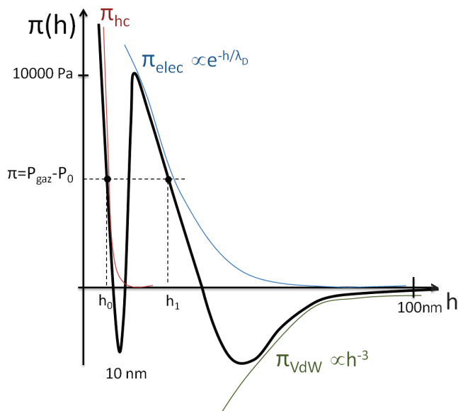
Figure 1.5: Isotherme de pression de disjonction schématisé, avec les différentes contributions, \Pi_{elec} , \Pi_{vdW} , \Pi_{hc} . La pression de disjonction est déterminée par la différence P_{gaz} - P_0 , ce qui fixe les épaisseurs de film possibles, h_0 et h_1
