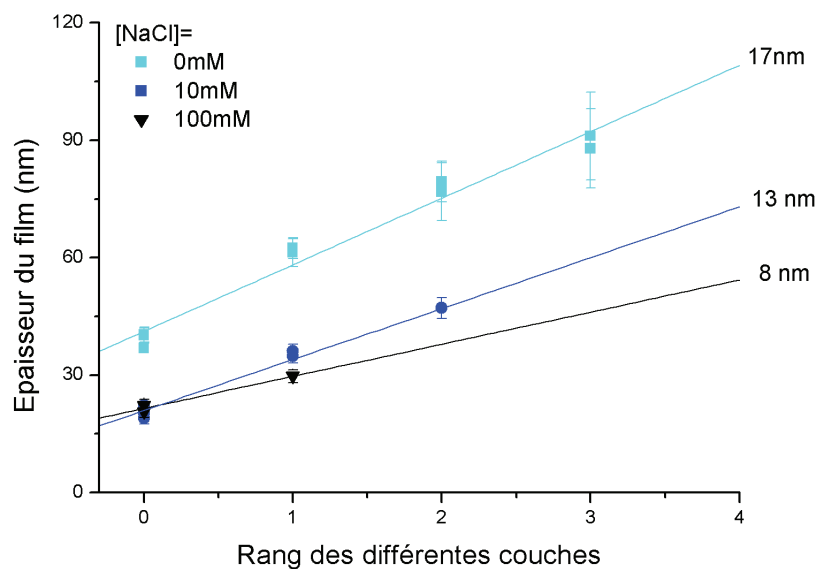
Figure 5.23: Epaisseurs de couches de stratification observées lors du drainage pour différentes concentrations en NaCl (0,10 et 100mM) pour une film d'AzoTAB de concentration 46mM, de composition équilibrée sous bleu et placé dans l'obscurité. L'épaisseur des couches et leur nombre diminue avec la concentration en sel, comme observé également pour les galettes.
