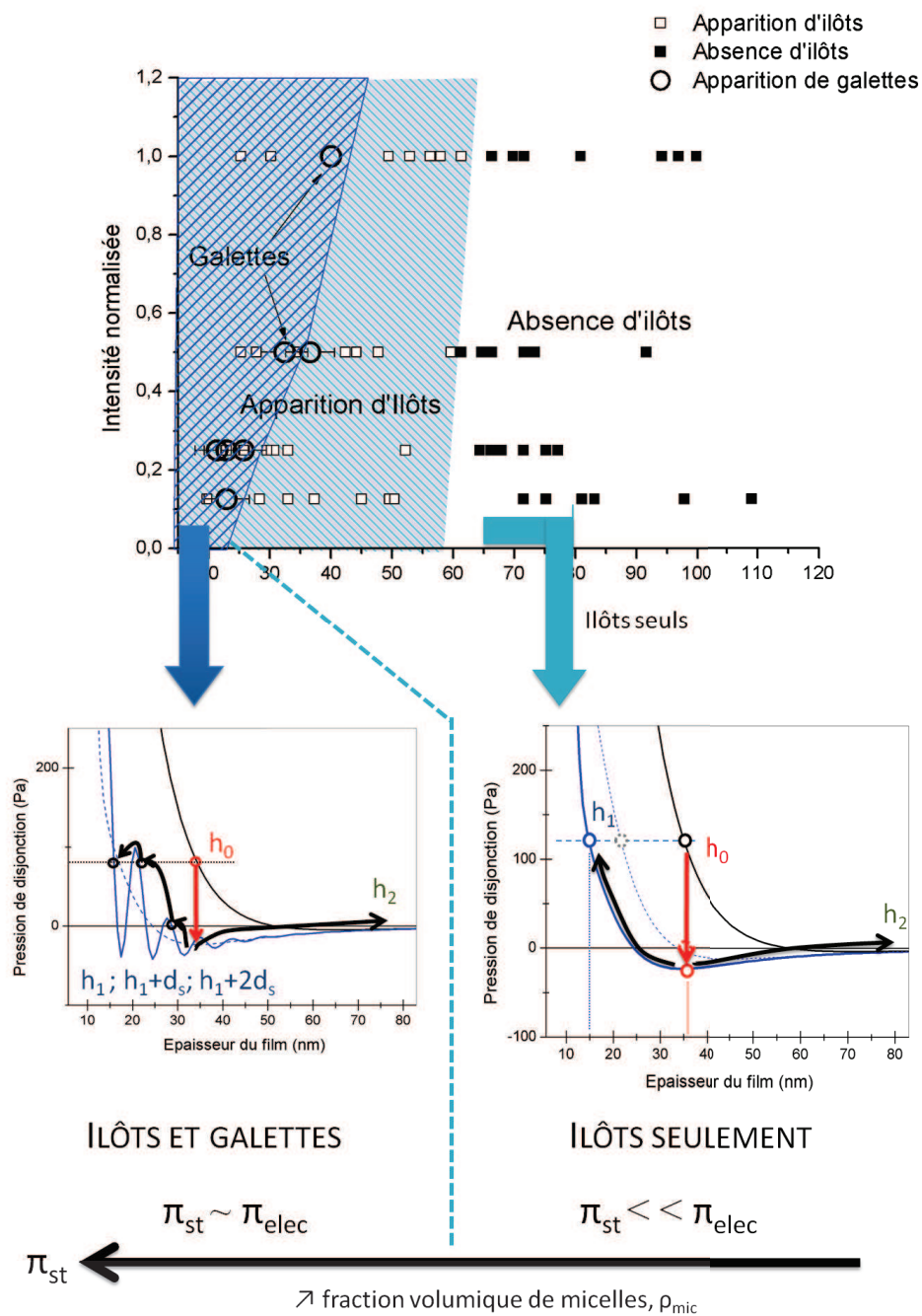
Figure 5.27: Isothermes de pression de disjonction associés à chaque domaine du diagramme de phase des îlots et gallettes. La formation des îlots s'explique seulement par la modification des interactions électrostatiques alors que le formation des gallettes nécessite l'apparition du terme stérique pour une augmentation importante de la concentration sous stimulus
