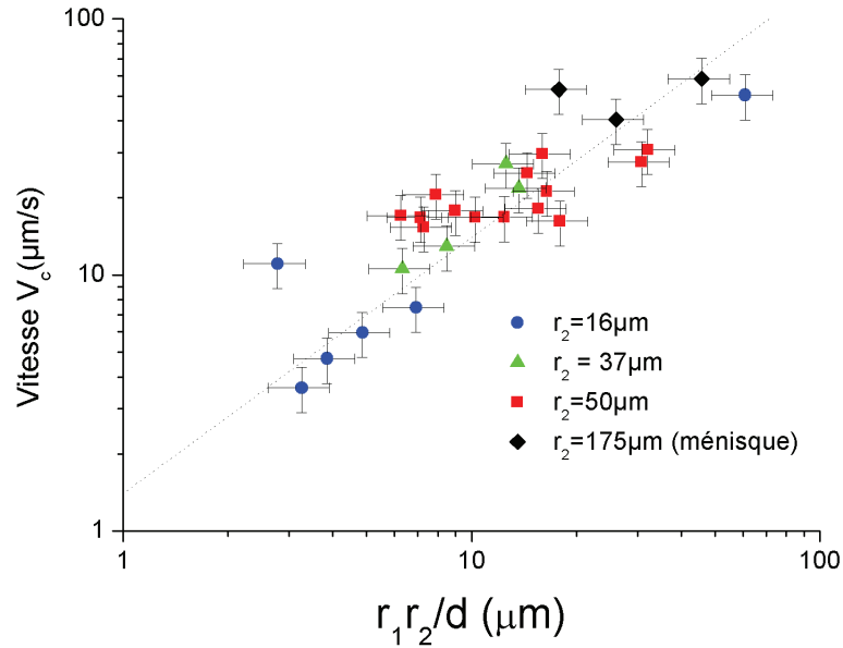
Figure 5.22: Vitesse relative des îlots, V_c avant leur coalescence en fonction du paramètre \frac{r_1 r_2}{d_i} , pour différentes tailles d'îlots r_2 . Les différentes vitesses ne semblent dépendre que du paramètre \frac{r_1 r_2}{d_i} , indiquant que le moteur de la coalescence est les interactions capillaires. La pente est de \nu=1,4s^{-1} . Les grandeurs r_1, r_2, d_i sont respectivement les rayons des deux îlots et la distance les séparant.
