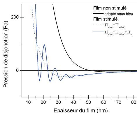
Figure 5.24: (gauche) Isothermes de pression de disjonction sous stimulus bleu. L'isotherme en pointillés ne comprend que les termes électrostatiques et de Van der Waals, l'isotherme en traits pleins inclut la contribution stérique liée à l'augmentation de la concentration.
