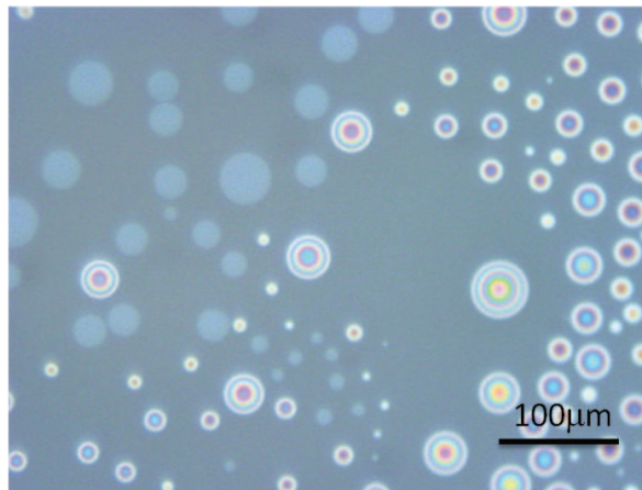
Figure 5.1: Observations d'un film de savon sous stimulus UV ou bleu : génération de deux types de formes sur le film. Les "galettes" sont des disques peu épais (disques grisés) et d'épaisseur bien définie ( \sim 10\text{nm} ). Les "îlots" sont des calottes sphériques (anneaux colorés concentriques) et peuvent atteindre une hauteur de plusieurs centaines de nanomètres.
