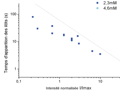
Figure 5.7: (droite) Temps d'apparition des îlots en fonction de l'intensité du stimulus pour une solution équilibrée en bleu et stimulée sous bleu, de concentration 2,3mM et 4,6mM. Le temps d'apparition des îlots semble inversement proportionnel à l'intensité tout comme le temps de photo-conversion, tracé pointillé. I_{max} \simeq 10\text{à}20\text{mW/cm}^2 .
