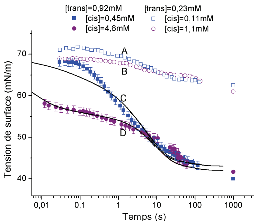
Figure 4.9: Ajustement du modèle mathématique d'adsorption avec les données expérimentales pour obtenir les différentes constantes d'adsorption du système. Les constantes d'adsorption k_{ads}^0 sont obtenues par fit aux temps courts et les constantes de désorption aux temps longs.
