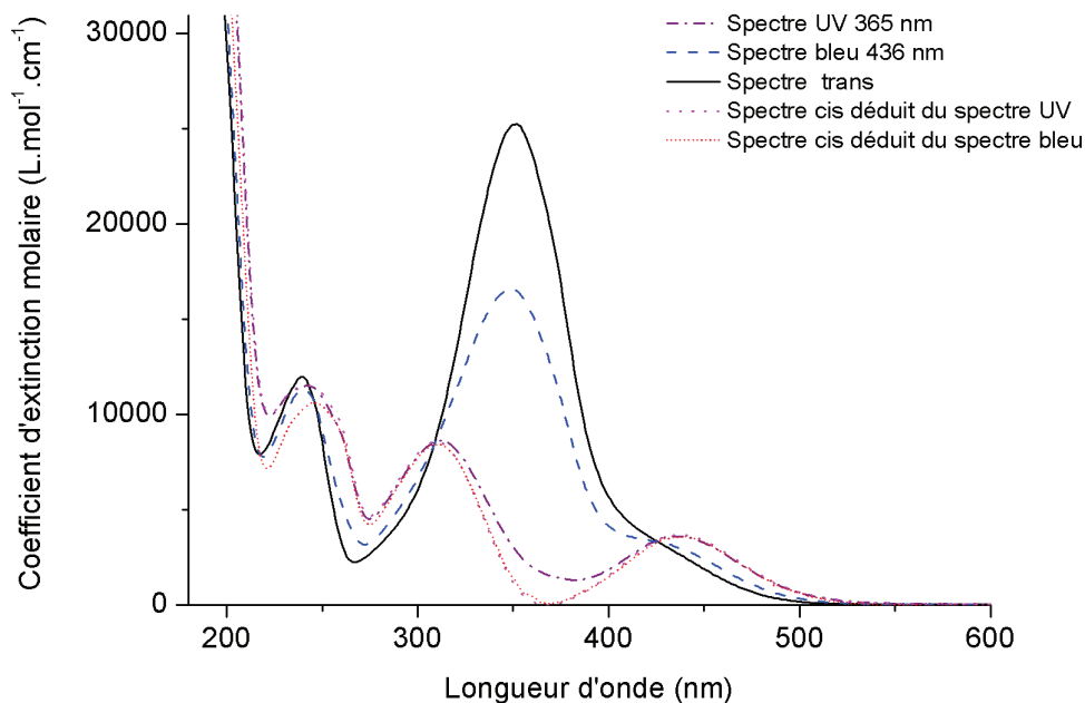
Figure 3.5: Spectres Uv-Vis de l'AzoTAB dans l'eau pour différentes compositions Les spectres des solutions équilibrées en UV, bleu et obscurité(100 % trans) sont mesurés sur une solution à 10mg/L. Le spectre d'une solution 100 % cis est déduit du spectre sous bleu et du spectre sous UV.
