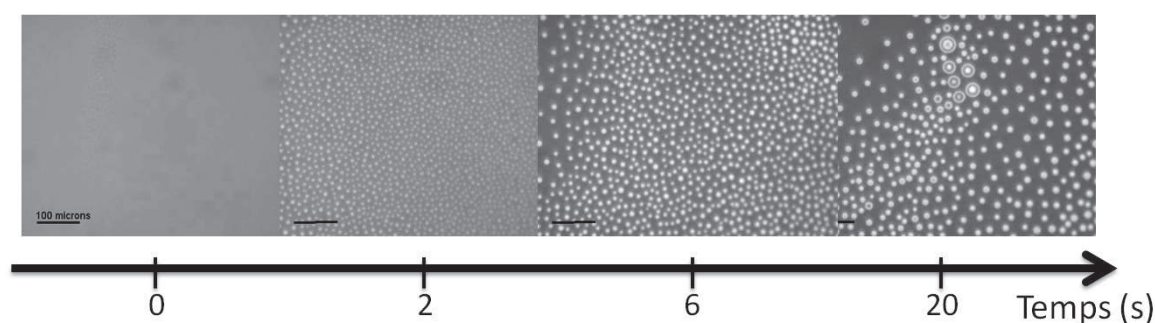
Figure 5.4: Photos de l'apparition d'îlots sous une stimulation bleue uniforme. Les îlots apparaissent simultanément et avec un motif très régulier.
