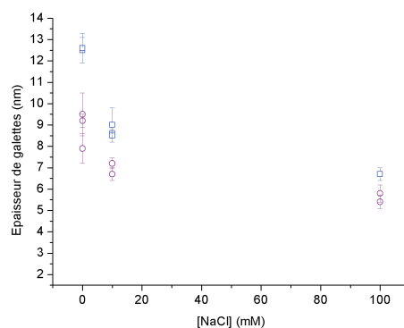
Figure 5.11: (droite) Épaisseurs des galettes pour différentes concentrations en NaCl (0,10 et 100mM) Les deux séries de données correspondent au stimulus bleu et au stimulus UV. Pour une même concentration en sel, les points correspondent à différentes intensités. ( c=3,5\text{mM} ) )
