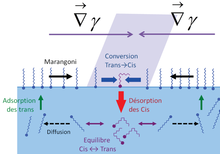
Figure 4.21: Bilan des flux d'adsorption à une interface photo-stimulée localement : génération d'un effet Marangoni
