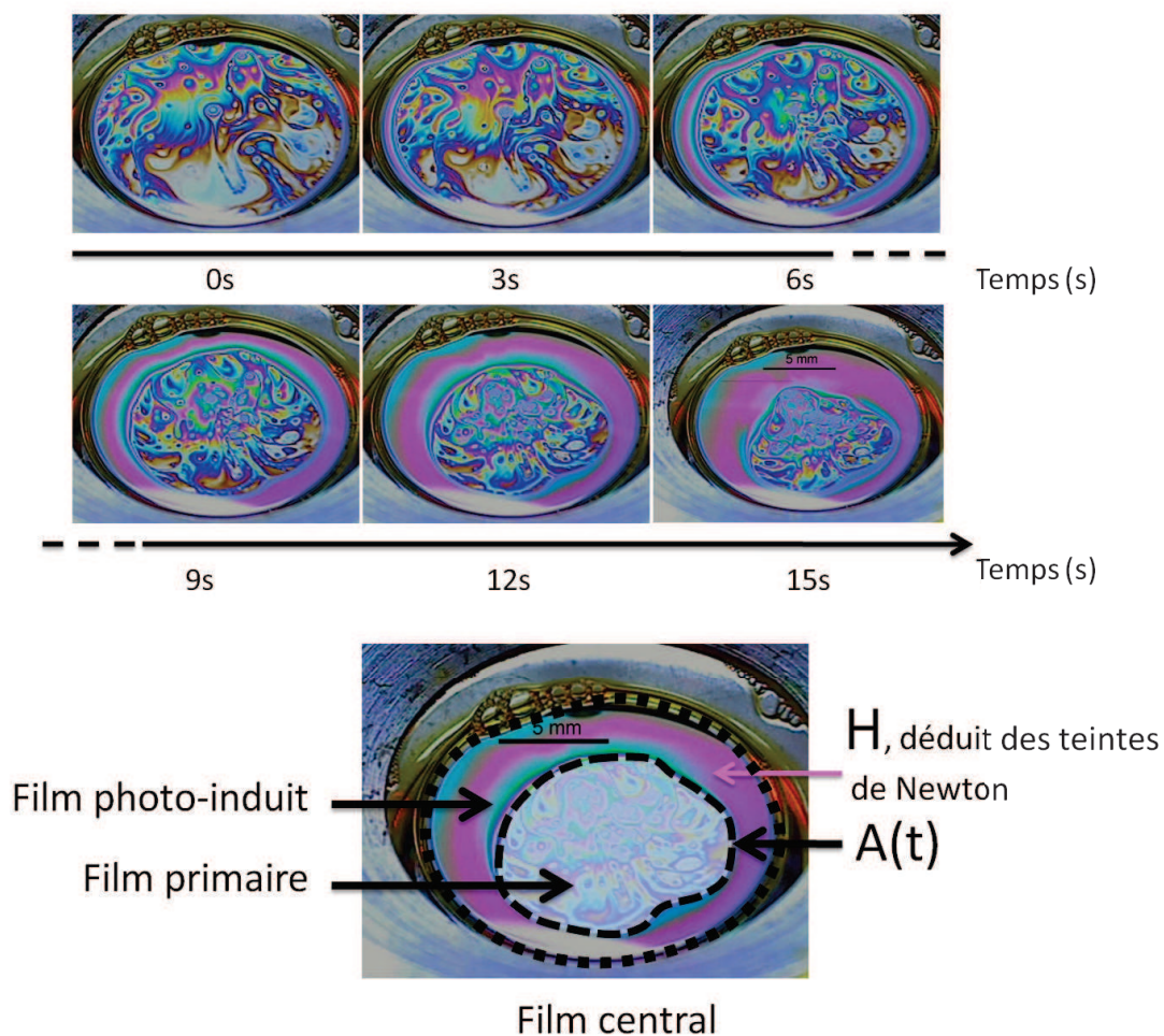
Figure 6.7: Séquence d'images de l'écoulement photo-induit par l'UV ( c=1,1 mM, I=0,5mW/cm^2 ). Un film d'épaisseur bien définie s'avance du bord de Plateau vers le centre du film.
