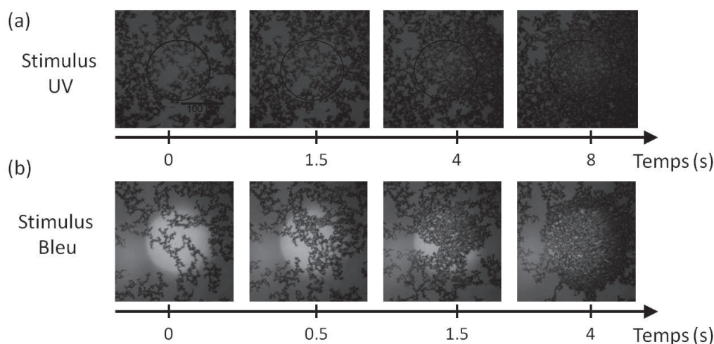
Figure 4.13: Observations des écoulements de Marangoni sur un interface stimulée grâce à une poudre de talc. Le cas (a) représente le cas usuel où une solution équilibrée en bleu est stimulée en UV, le mouvement du talc vers le spot UV traduit l'augmentation locale de tension de surface. La même observation est faite pour une solution équilibrée en bleu puis stimulée en bleu (cas (b)), traduisant la perturbation de l'interface sous stimulus. (Echelle de 100 \mu\text{m} donnée sur la première image)
