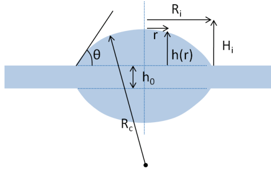
Figure 5.21: Profil d'un îlot et des grandeurs associées. R_c est le rayon de courbure.
