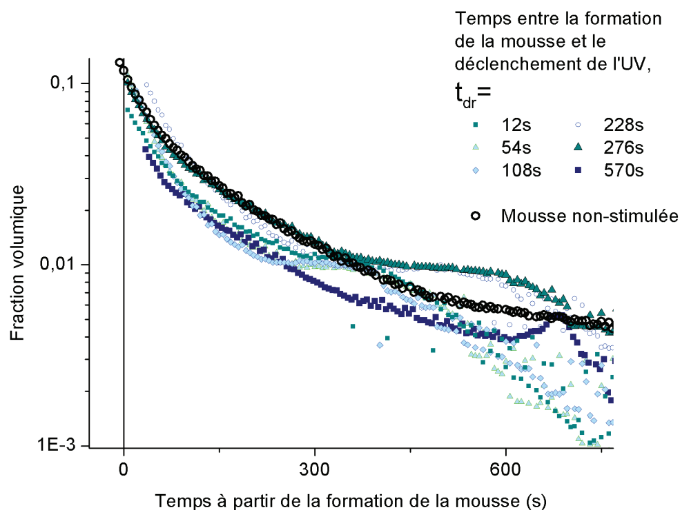
Figure 6.21: Evolution de la fraction volumique de liquide pour des mousses ayant plus ou moins drainé avant le déclenchement de l'UV, en fonction du temps de drainage des mousses. Le drainage des mousses irradiées après un temps t_{dr} variable est comparé au drainage d'une mousse non stimulée. Jusqu'à des fractions supérieures à \phi \simeq 1\% environ, le drainage est semblable malgré le déclenchement de l'UV.
