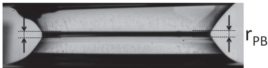
Figure 6.6: Mesures du rayon de bord de Plateau sur une image de profil en rétro-éclairage.
