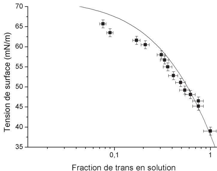
Figure 4.3: Tension de surface en fonction de la fraction molaire de trans pour une solution de concentration 1,15mM
