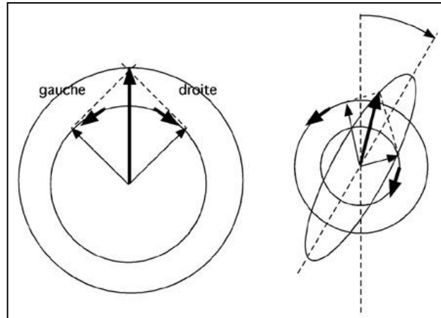
Figure 18 : Représentation du dichroïsme circulaire. Gauche absorption équivalente de la lumière polarisée droite et gauche. Droite : Absorption préférentielle de la lumière polarisée droite
