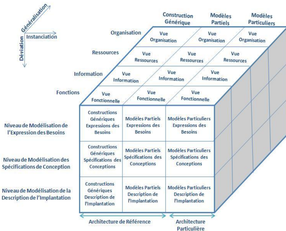
Figure 3.4. Cadre de Modélisation CIMOSA (Vernadat, 1996)
