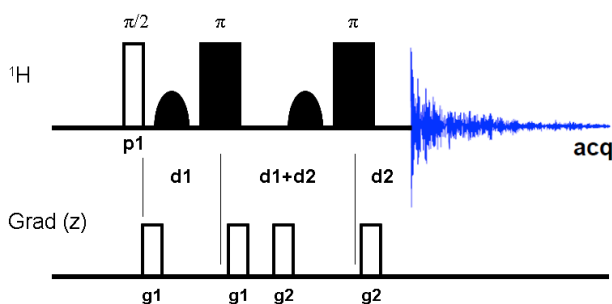
Figure 37 : Séquence d'impulsions excitation sculpting.
