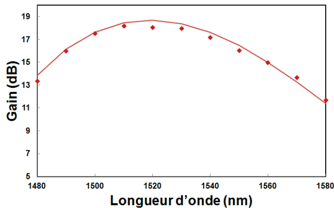
Figure 3-4 : Mesures (points) et simulations (trait continu) du gain optique en fonction de la longueur d'onde pour un courant de polarisation de 200 \text{ mA} et une puissance d'entrée de -20 \text{ dBm} .
