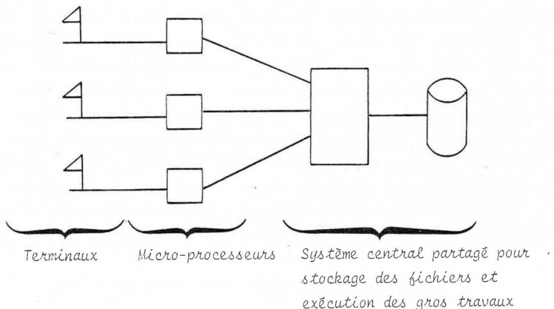
Figure 2: Exemple de système multi-processeurs
