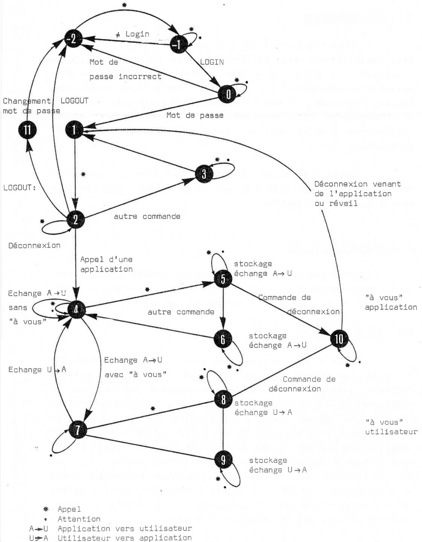
Figure_32: Automate associé à chaque utilisateur
