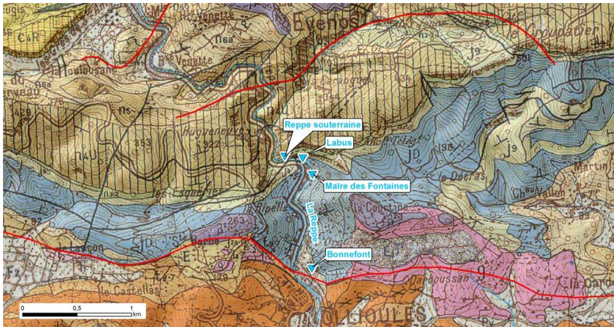
Figure 4.8 : Localisation sur la carte géologique au 1/50000 du BRGM de la source de la Maire des Fontaines, ainsi que des sources de la Reppe souterraine, du Labus et de Bonnefont. Les deux dernières ont été suivies pour ce travail.
