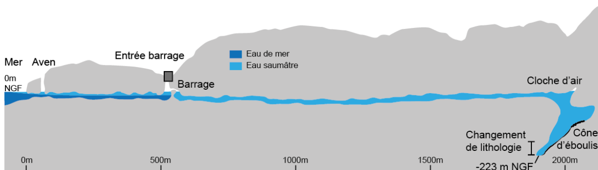
Figure 3.3 : Topographie en coupe de la partie explorée au 07/05/2012 de la source sous-marine de Port-Miou (modifié d'après Méniscus, 2012).
