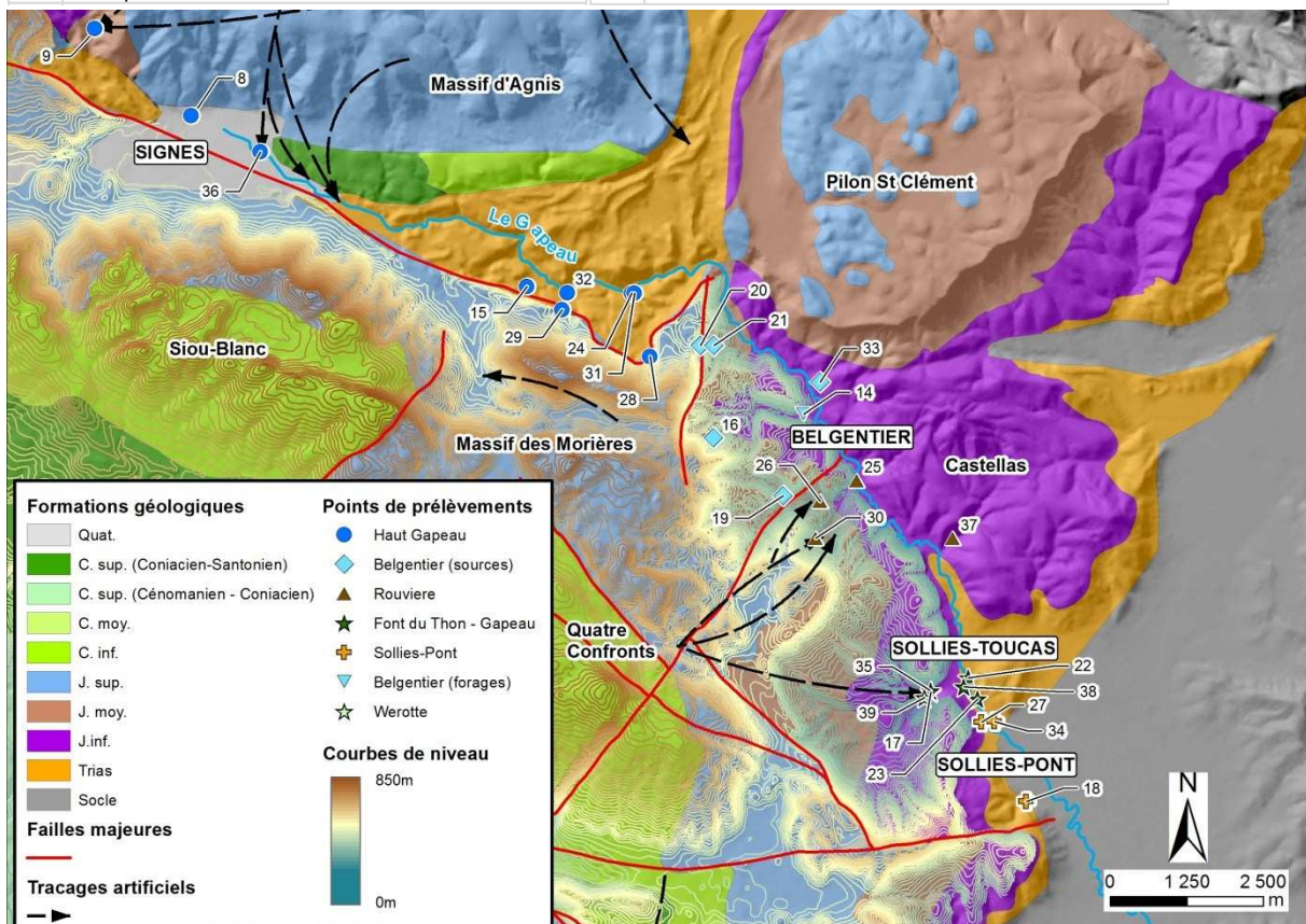
Figure 4.10 : Localisation des prélèvements des ions majeurs et des sous-secteurs pour l'aire du Gapeau. Les tracages artificiels sont issus des travaux de Lamarque & Maurel (2001) et de Gilli (2000).
