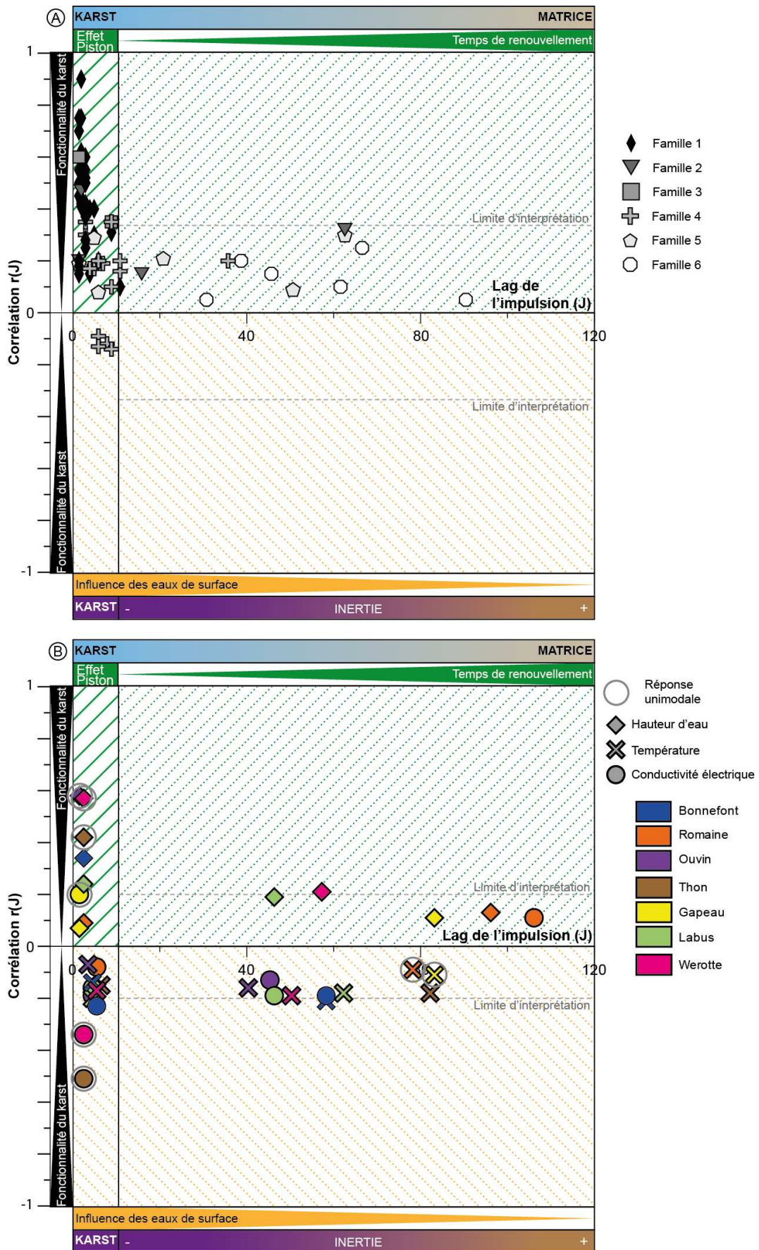
Figure 3.30 : Réponses impulsionnelles des sources issues de la bibliographie (A) et de l'Unité du Beausset (B) replacées dans la classification MIB.
