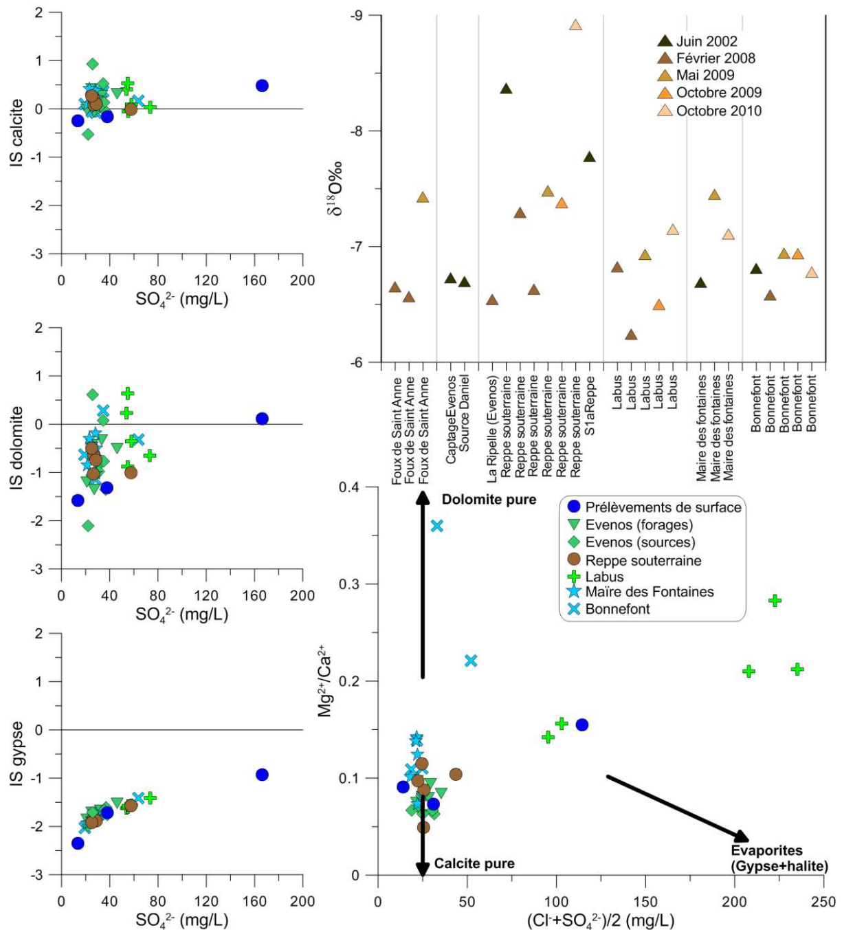
Figure 4.16 : Discrimination de l'origine de l'eau selon les sous-secteurs de l'aire d'Evenos – Ollioules en fonction des teneurs en calcium, magnésium, chlorures et sulfates et \delta^{18}O .
