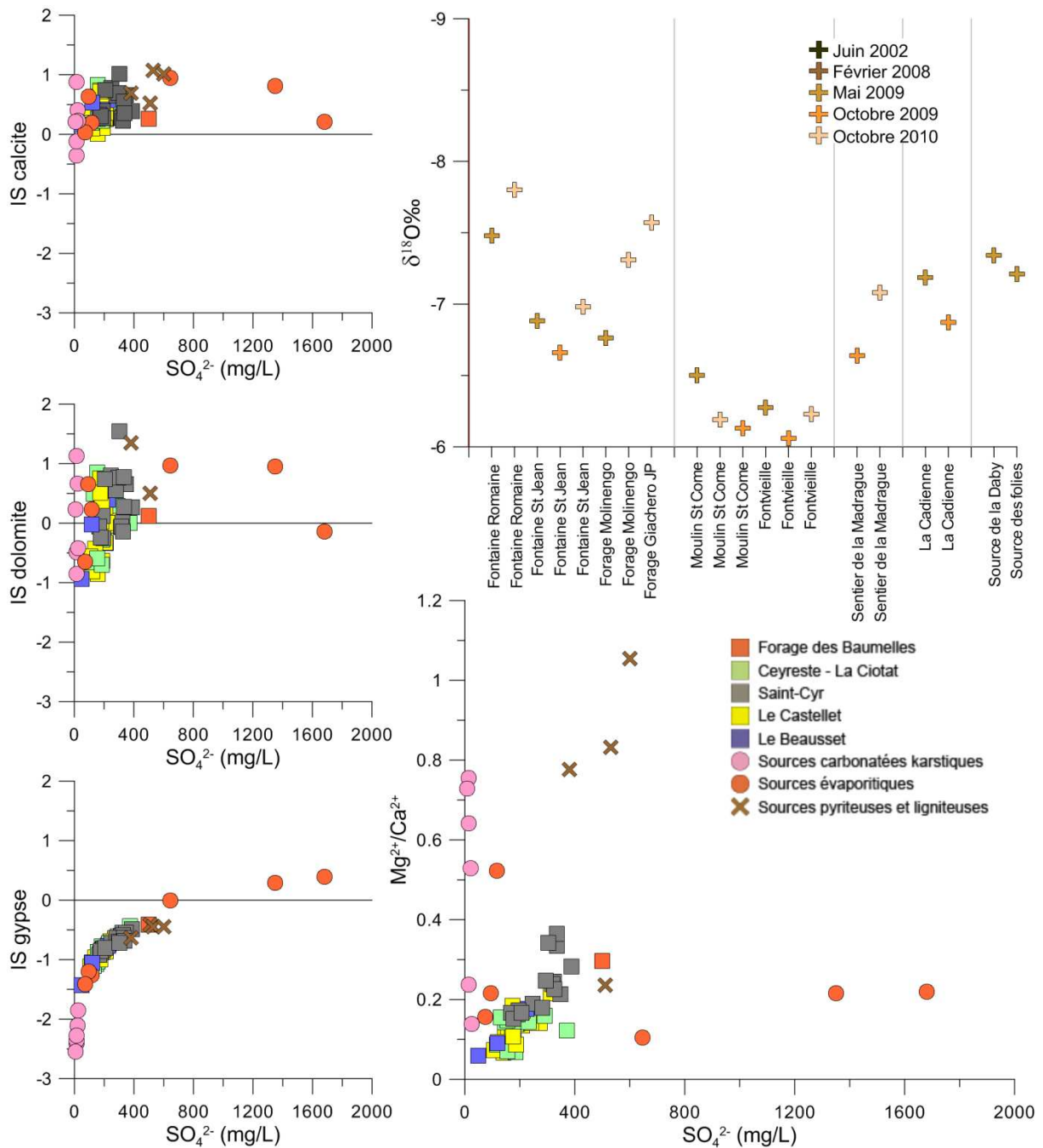
Figure 4.19 : Discrimination de l'origine de l'eau selon les sous-secteurs de l'aire d'Evenos – Ollioules en fonction des teneurs en calcium, magnésium, sulfates et \delta^{18}\text{O} .
