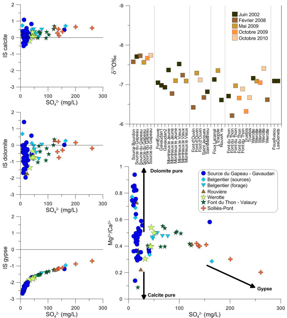
Figure 4.11 : Discrimination de l'origine de l'eau selon les sous-secteurs de l'aire du Gapeau en fonction des teneurs en calcium, magnésium, sulfates et \delta^{18}\text{O} .
