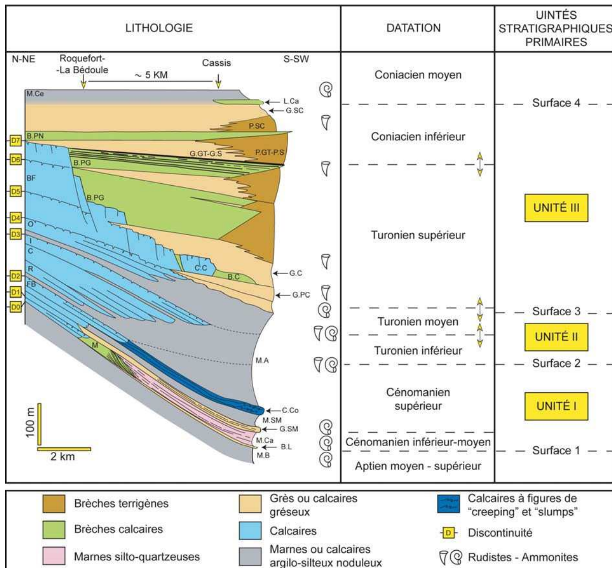
Figure 2.11 : Schéma synthétique des séries sédimentaires d'âge Cénomaniens à Coniaciens moyens de la bordure nord-nord-est à sud-sud-ouest de la marge carbonatée du Bassin Sud-Provençal. Position et datation des unités lithostratigraphiques. M.B : Marnes Bleues ; B.L : Banc des Lombards ; M : Formation de la Marcouline ; M.Ca : Marnes de Cassis ; G.SM : Grès de l'Anse Sainte Magdeleine ; M.SM : Marnes de l'Anse Sainte Magdeleine ; FB : Formation de Font Blanche ; C.Co : Calcaires du Corton ; M.A : Marnes de l'Anse de l'Arène ; R : Barre de Roquefort ; C : Barre des Cuettes ; I : Barre Intermédiaire ; O : Barre du Pas d'Ourié ; BF : Barre de Bellefille ; G.PC : Grès du Pas de la Colle ; C.C : Couronne de Charlemagne ; B.C : Barre de Canaille ; G.C : Grès de Canaille ; B.PG : Barre du Pin de Galaban ; G.GT-GS : Grès de la Grand Tête et du Sémaphore ; P.GT-P.S : Poudingues de la Grand Tête et du Sémaphore ; B.PN : Barre du Pont Naturel ; G.SC : Grès de Sainte-Croix ; P.SC : Poudingues de Sainte-Croix ; L.Ca : Lentille de Cabot ; M.Ce : Marnes de Ceyreste. D'après Gari (2008), établi à partir des travaux de Jolet (1996 ; Turonien inférieur à moyen) et de Hennuy (2003 ; Turonien moyen à Coniacien moyen).
