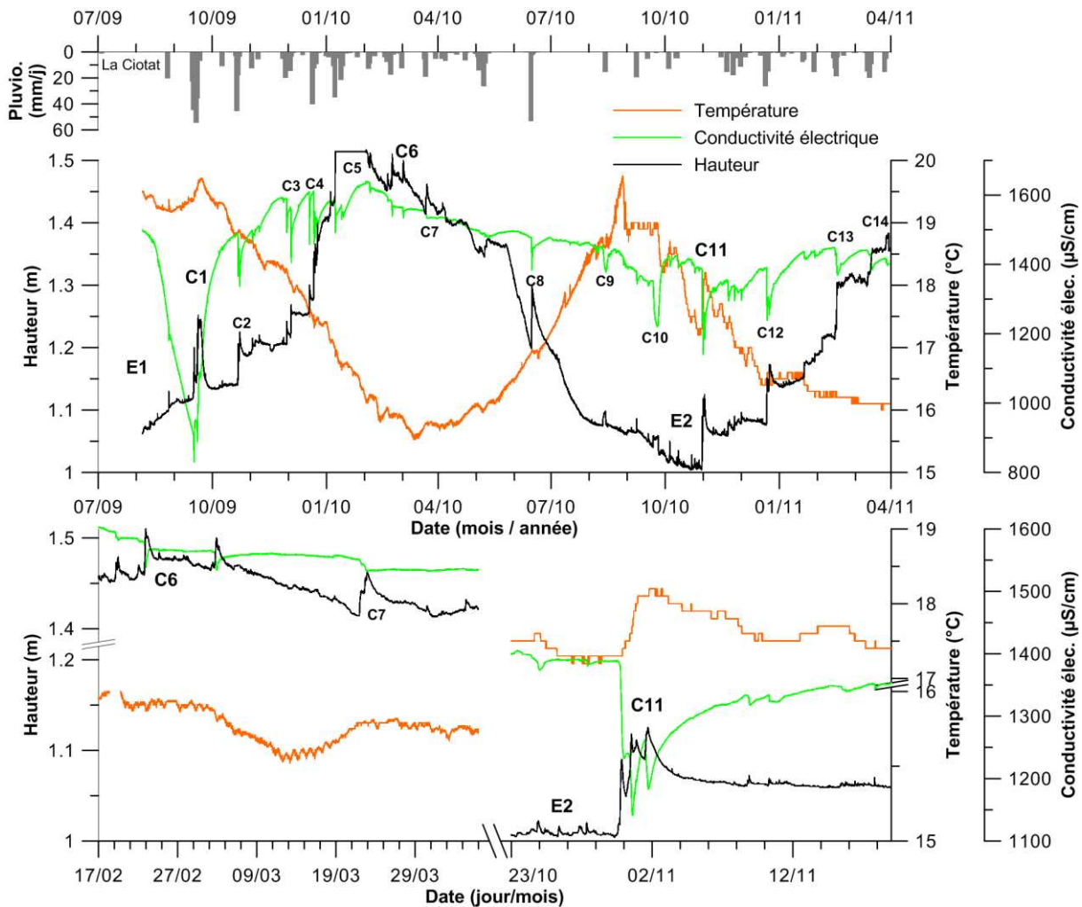
Figure 3.2 : Enregistrement CTD de la source de la Fontaine Romaine, associé aux précipitations journalières sur la même période. Les périodes d'étiage sont notées « E » et les crues « C ». Deux crues, C6 et C11, sont exposées à titre d'exemple.
