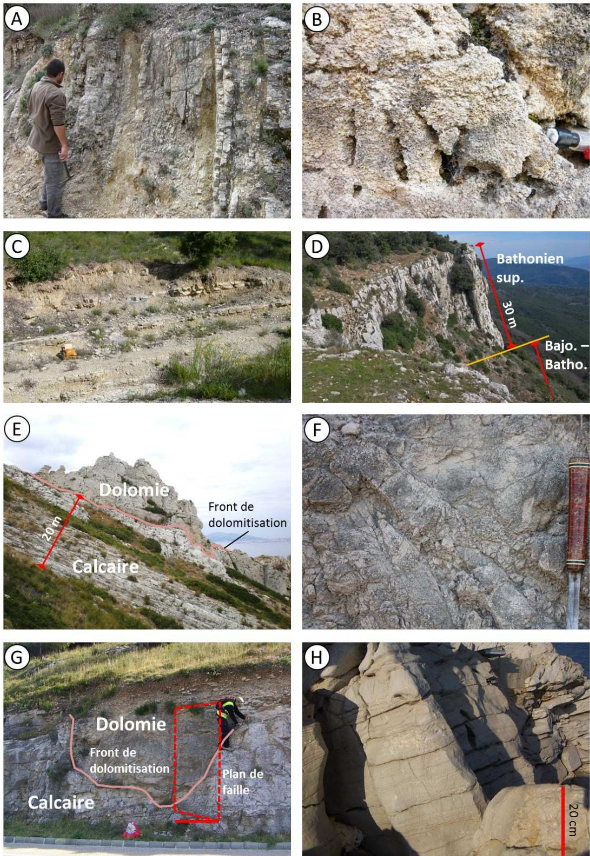
Figure 2.5 : Illustrations des principales formations jurassiques. (A) Marnes vertes et dolomies sucrosiques fracturées de l'Hettangien (Signes). (B) Calcaires à entroques du Pliensbachien (Solliès-Toucas). (C) Alternances marno-calcaires du Bajocien (Solliès-Toucas). (D) Calcaires fracturés du Bathonien sup. et début
