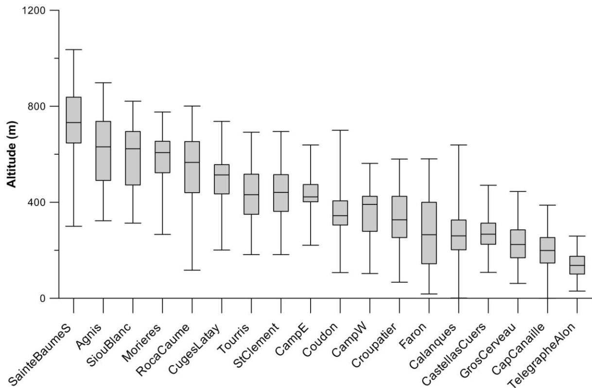
Figure 4.7 : Box-plots des altitudes des différents massifs de l'Unité du Beausset extraites du MNT au 1/25000 de l'IGN (IGN-BD Alti, 2011).
