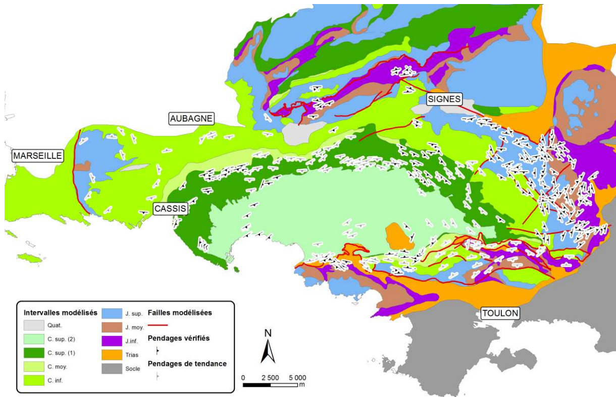
Figure 3.3 : Base de données pendages répartis selon les pendages vérifiés (en noir) et ceux servant seulement de tendance (en gris).
