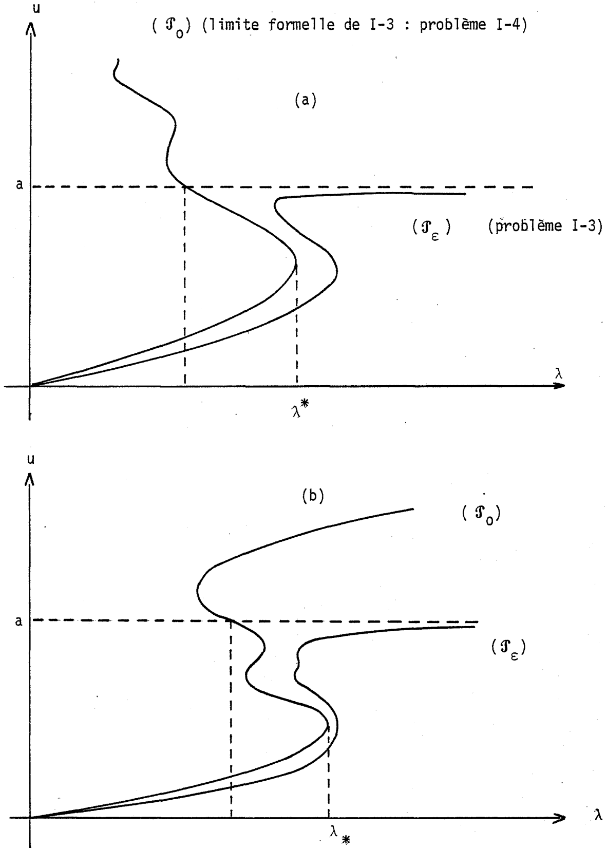
Figure 1 : (a) cas où ( \mathcal{F}_0 ) n'a pas de solution pour \lambda assez grand. (b) cas où ( \mathcal{F}_0 ) a toutes ses solutions > a pour \lambda grand.
