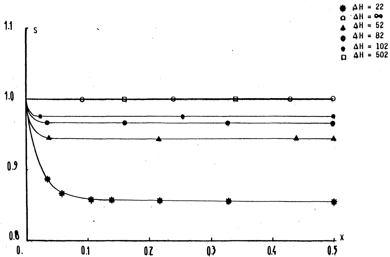
Figure 8 : Profils des concentrations normalisées lorsque \Delta H tend vers +\infty .
