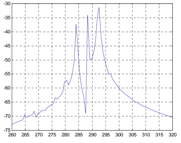
Fig 3-25 FFT Couple - Deux barres cassées Zoom 260-320 Hz
