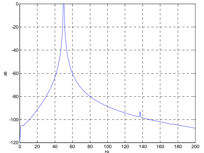
Fig 3-35 - FFT induction d'entrefer - machine saine - zoom 0-200 Hz.
