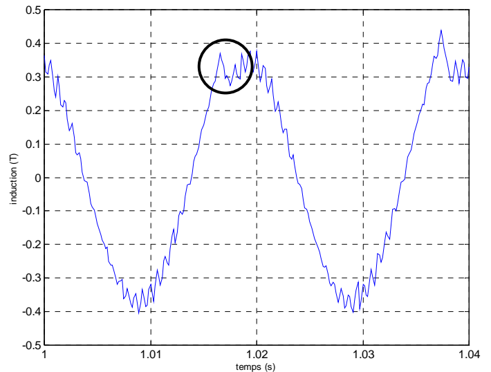
Fig 3-32 - Induction d'entrefer en fonction du temps - une barre cassée
