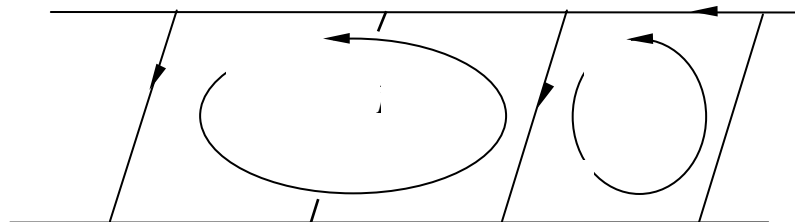
figure 1-11 : Schématisation d'une barre cassée sur un rotor à cage d'écureuil.
