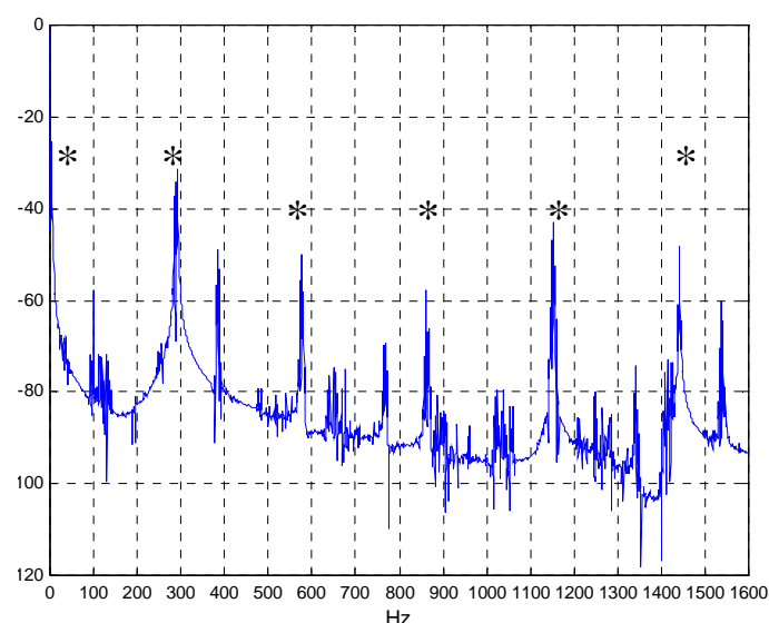
Fig 3-23 - FFT Couple Deux barres cassées - \approx 2883 trs/min
