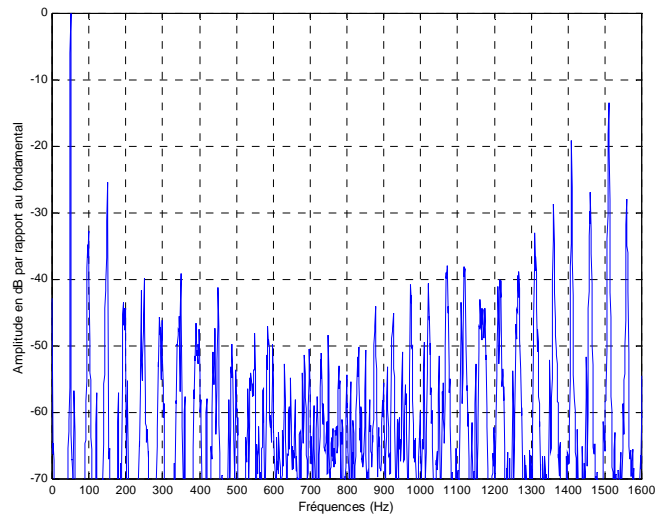
Fig 4-27 FFT induction d'entrefer Deux barres cassées
